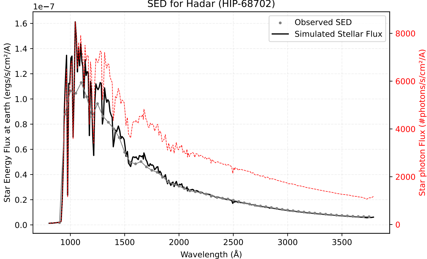
SED for Hadar (HIP-68702)
