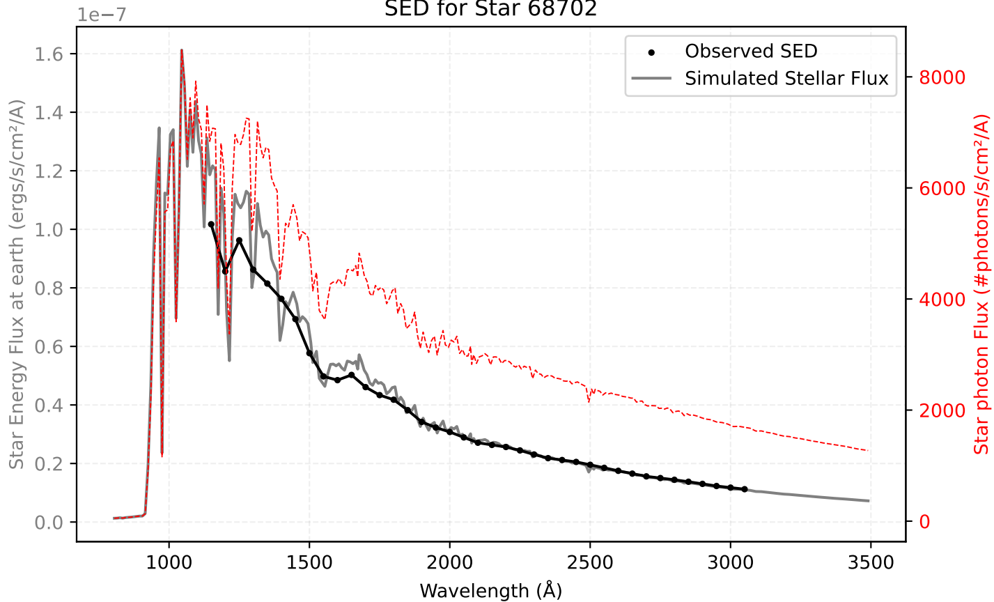
SED for Star 68702
