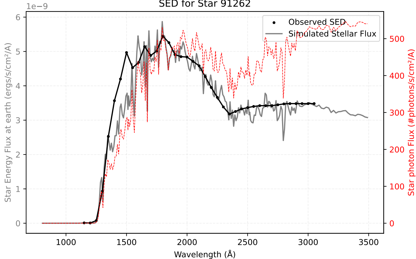
SED for Star 91262
