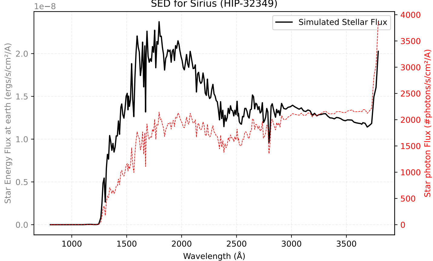
SED for Sirius (HIP-32349)
