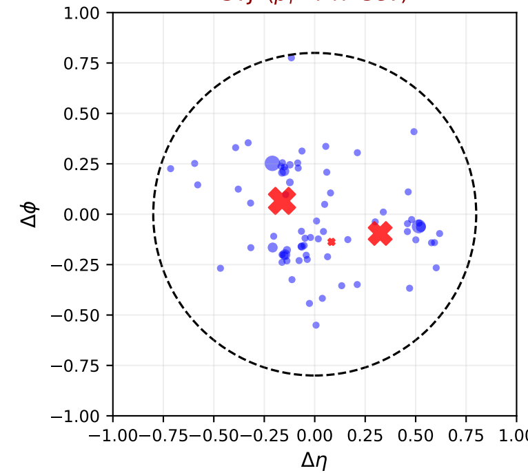
SM Jet ( p_T=100 GeV)
