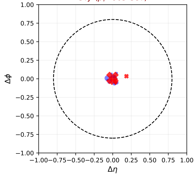
SM Jet ( p_T=134 GeV)
