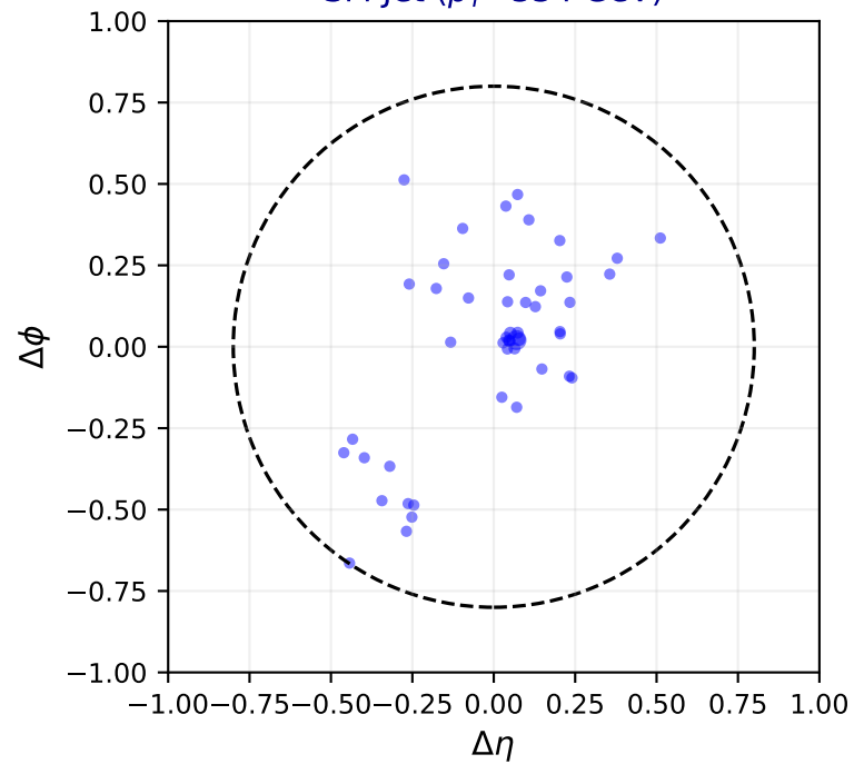
SM Jet ( p_T=334 GeV)
