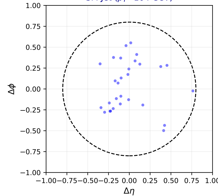
SM Jet ( p_T=104 GeV)
