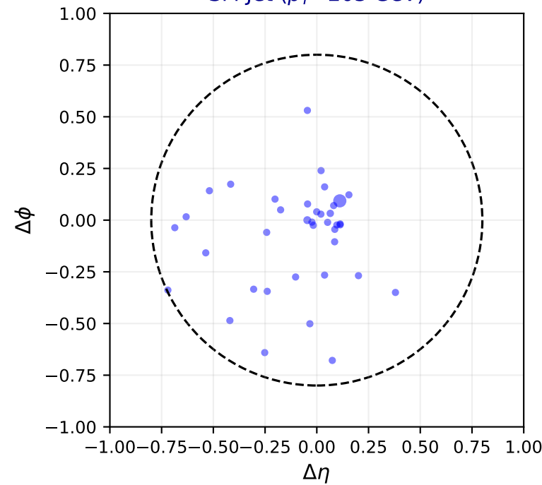
SM Jet ( p_T=203 GeV)
