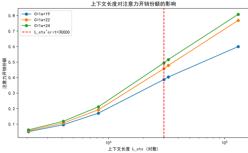
图 7.33 注意力开销份额随上下文长度的变化（红色虚线为临界点 30000）。
