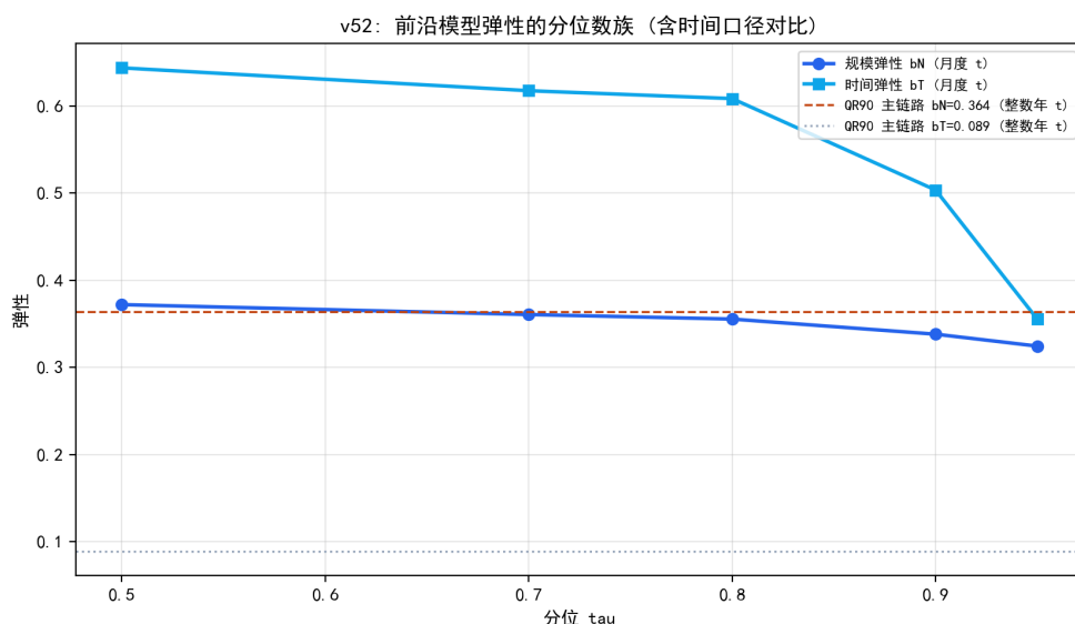
图 9.49 前沿弹性的分位数族与时间口径对比（ b_N 稳健， b_T 对口径敏感）。
