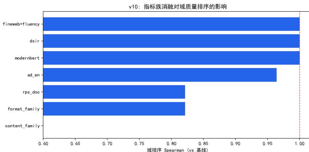
图 9.50 指标族消融对域质量排序的影响（红虚线为完全一致）。
