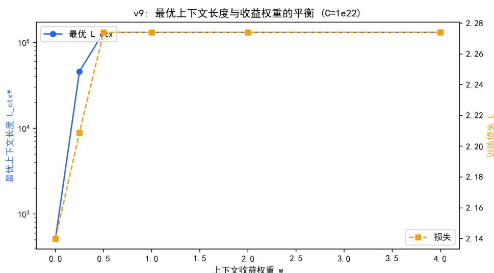
图 7.40 最优上下文长度与收益权重 w 的平衡（ C = 10^{22} ）。
