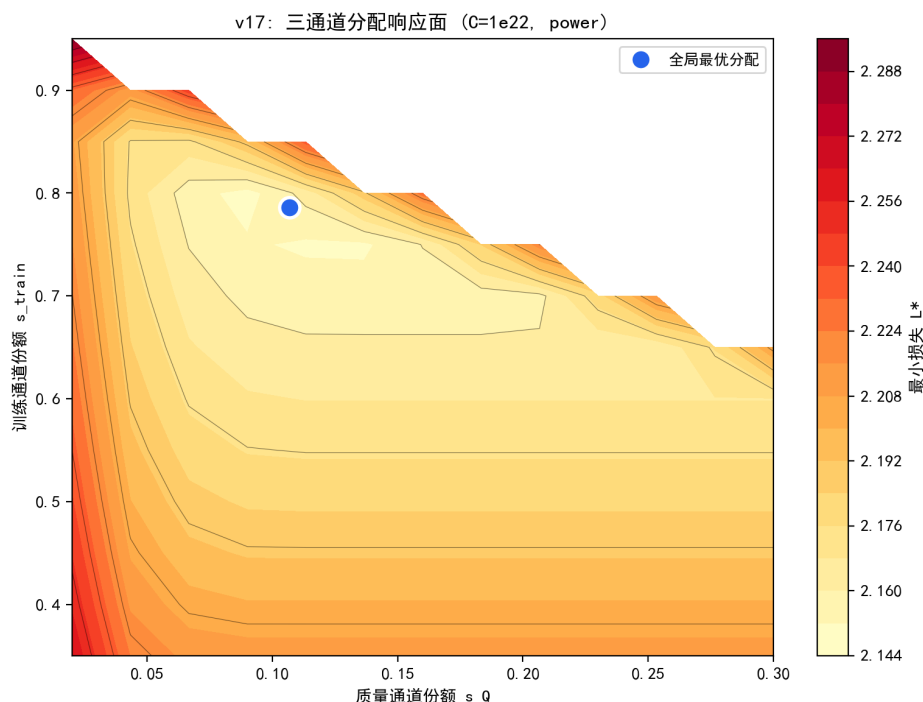
图 7.41 三通道分配响应面（ C = 10^{22} ，幂成本；蓝点为全局最优分配）。
