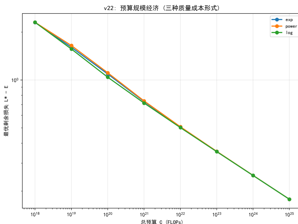
图 7.30 预算-最优损失的对数线性规律（三种质量成本形式）。
