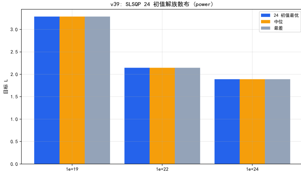
图 7.28 SLSQP 24 初值解族散布：三档预算全部初值收敛到同一最优。
