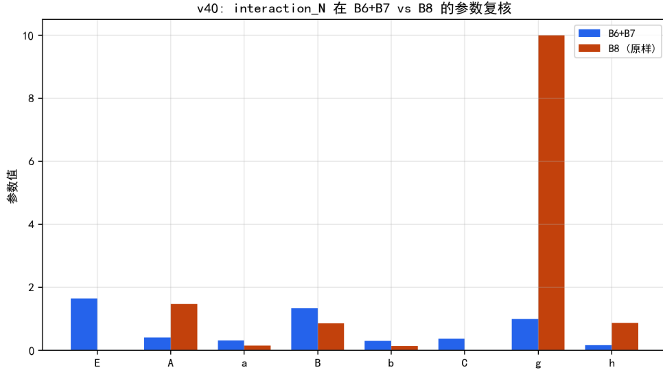
图 6.21 B8 原样 vs B6+B7 的参数对比：B8 质量项退化（ E = C = 0 , g 撞界）。
