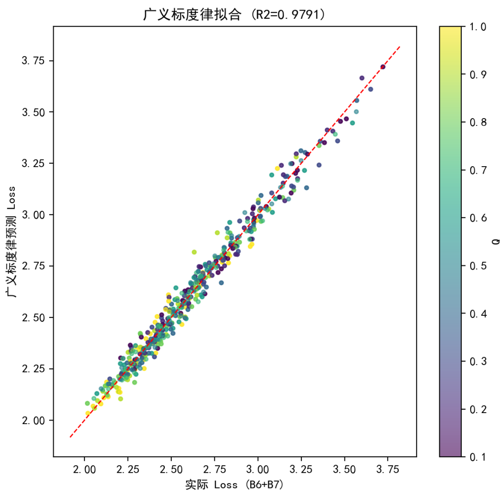
图 6.19 广义标度律在 B6+B7 数据上的拟合（质量-参数量交互形式， R^2 = 0.979 ）。
