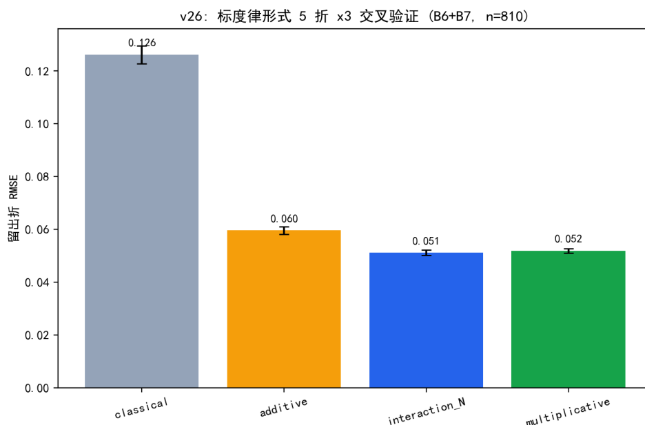
图 6.17 标度律形式 5 折交叉验证的留出 RMSE 对比。
