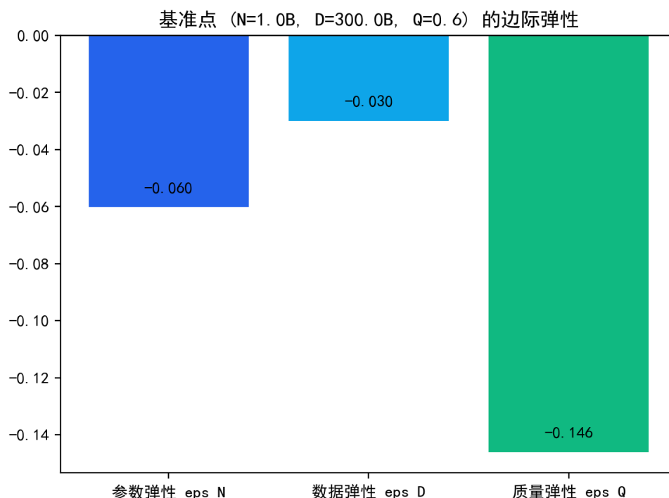
图 6.24 基准点处三个维度的损失弹性对比（质量弹性最高）。
