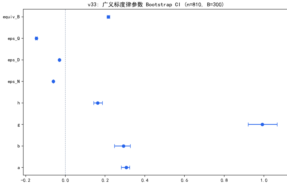
图 6.20 广义标度律参数与弹性的 Bootstrap 置信区间。
