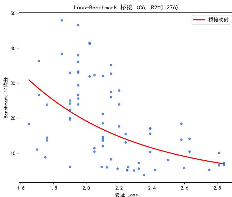
图 8.53 Loss-Benchmark 桥接映射 (C6, 75 个模型)。
