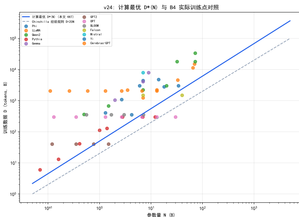
图 7.32 计算最优数据曲线 D^*(N) 、Chinchilla 经验规则与 B4 实际训练点。
