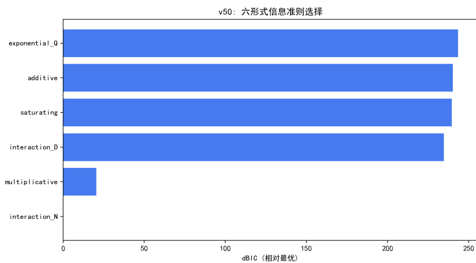
图 6.18 六种形式的 BIC/AIC 选择：interaction_N 决定性胜出。
