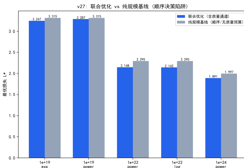
图 7.39 联合优化 vs 纯规模基线的最优损失（顺序决策陷阱：质量需预算预留）。
