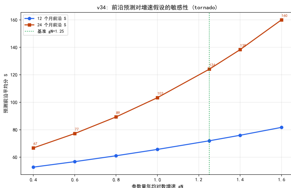
图 8.45 前沿预测对参数量增速假设 g_N 的敏感性（12/24 个月）。
