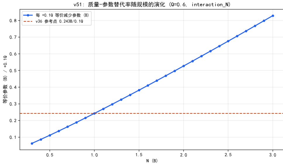
图 6.26 每 +0.1Q 等价减少的参数随规模的演化（近线性上升）。
