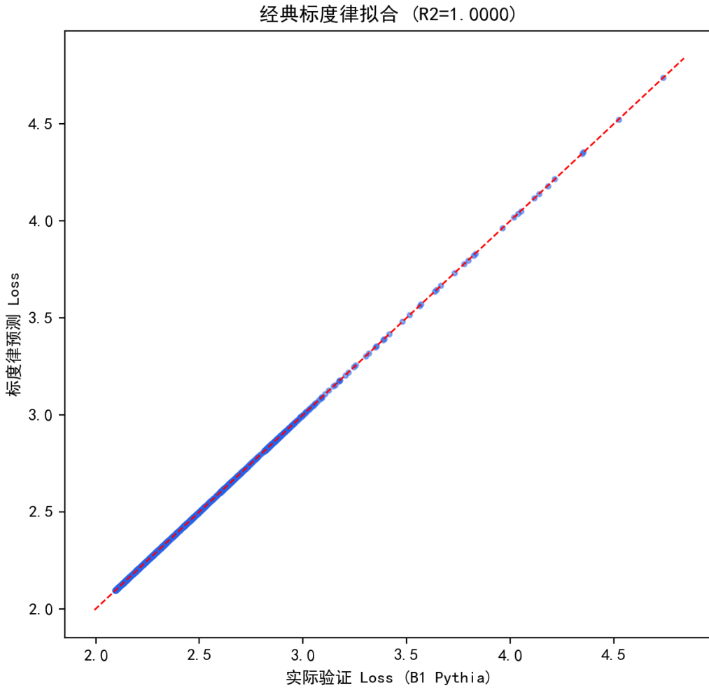
图 6.16 经典标度律在 B1 轨迹上的拟合与跨家族验证。
