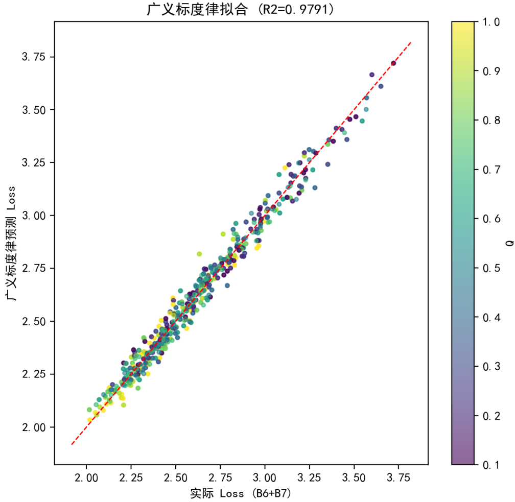
图 6.8 广义标度律在 B6+B7 数据上的拟合（质量-参数量交互形式， R^2 = 0.979 ）。
