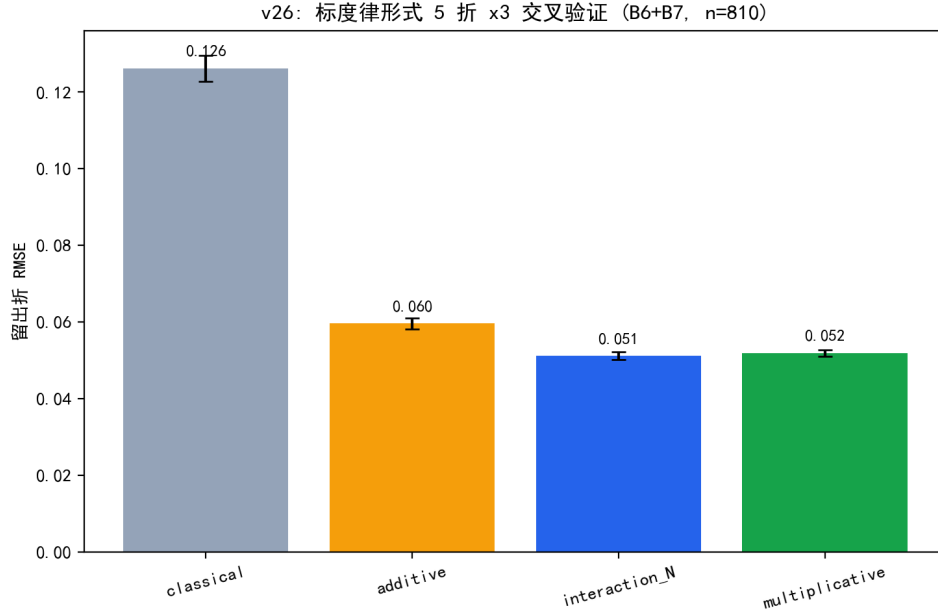
图 6.7 标度律形式 5 折交叉验证的留出 RMSE 对比。
