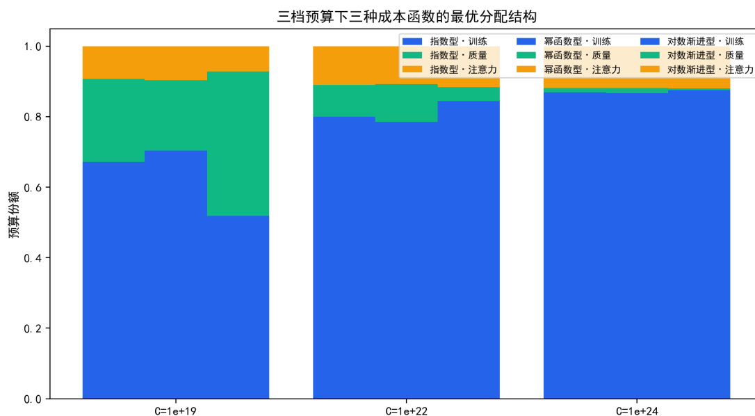
图 7.12 三档预算下三种质量成本函数的最优成本份额结构。
