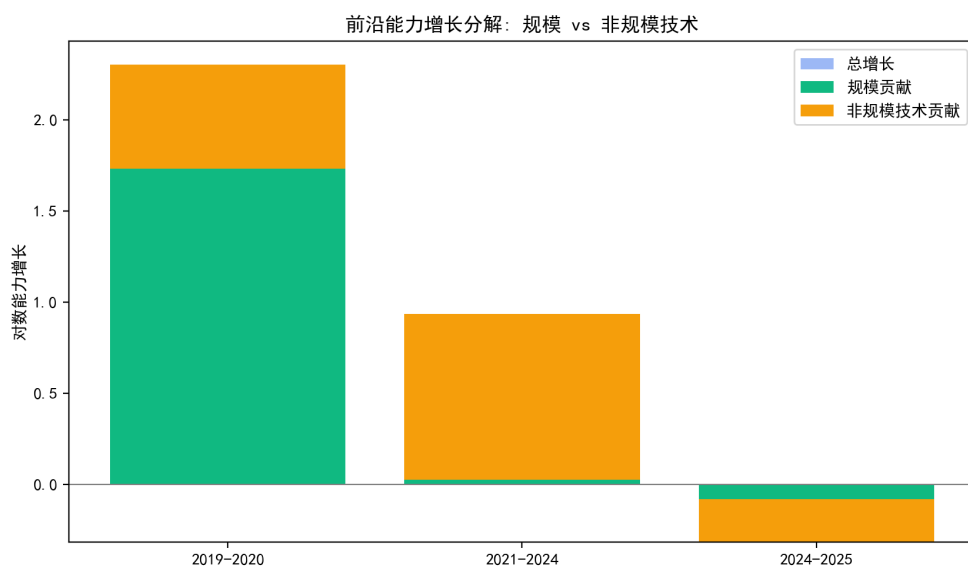
图 8.23 前沿能力增长分解：规模贡献与非规模技术贡献。
