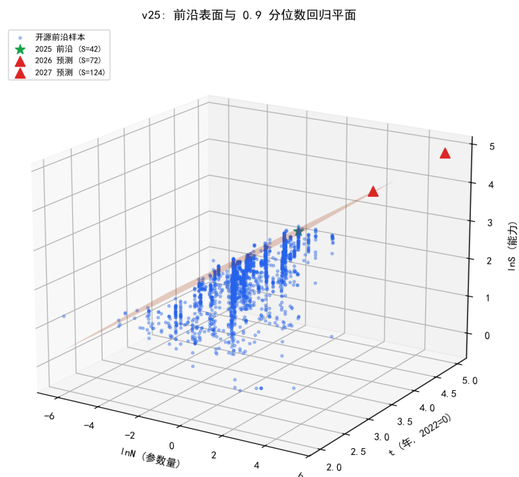
图 8.22 能力前沿 3D 表面与 0.9 分位数回归平面（星标 = 2025 前沿，三角 = 预测点）。
