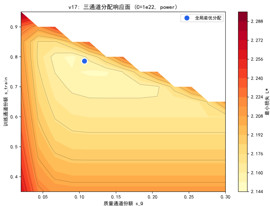
图 7.20 三通道分配响应面 ( C = 10^{22} ，幂成本；蓝点为全局最优分配)。
