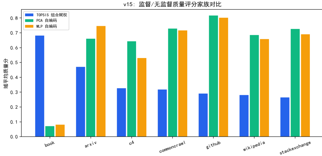
图 9.27 TOPSIS 组合赋权与自编码典型性评分的域级对照（方向相反）。
