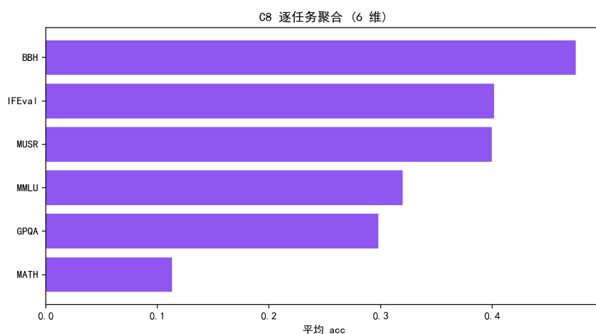
图 8.25 C8 逐任务聚合得分 (6 维)。
