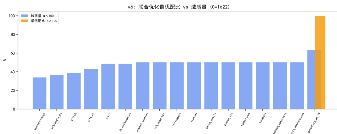
图 7.17 联合优化最优配比与域质量对比（ C = 10^{22} ）：配比向最高质量域（小说）集中。
