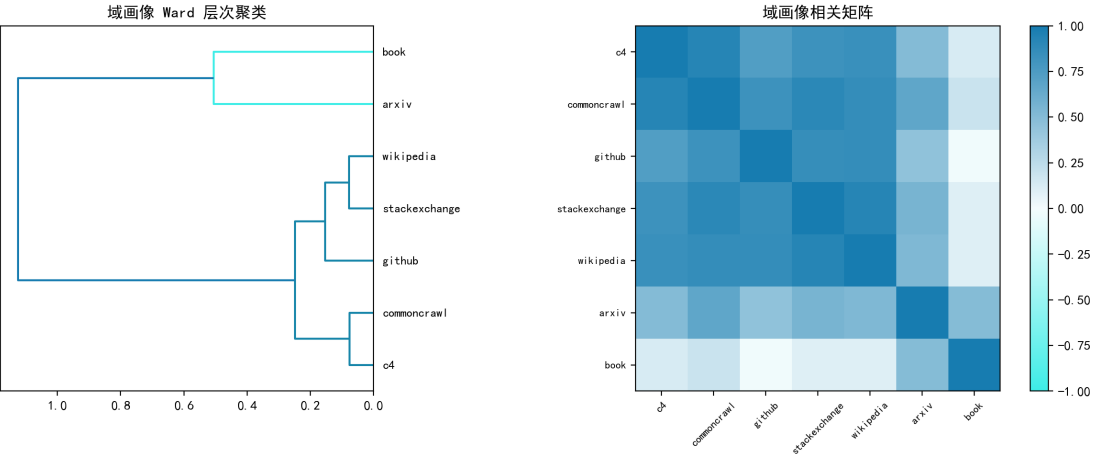
图 5.17 域画像层次聚类与相关矩阵： book 独树一帜、低质域聚簇。
