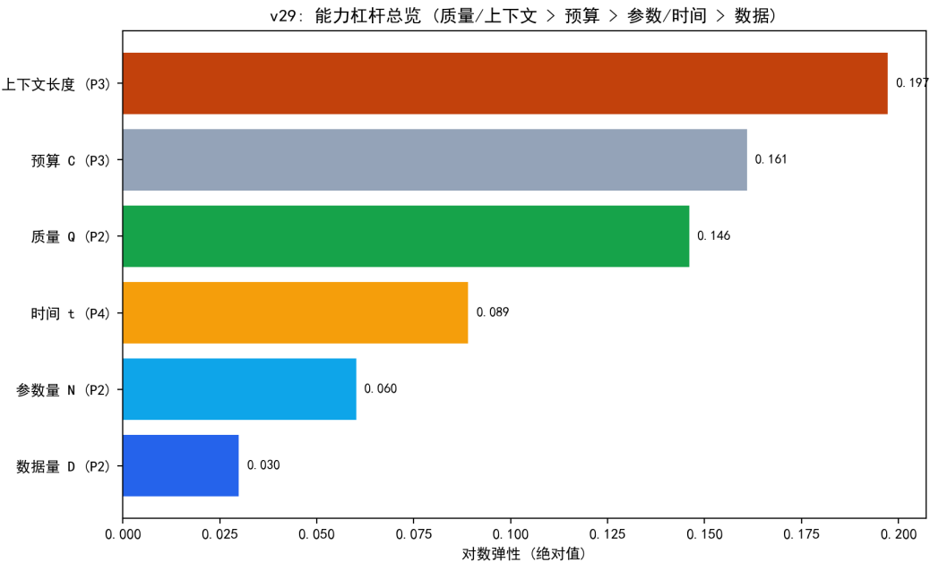
图 10.44 能力杠杆总览：各投入的对数弹性排序（质量/上下文 > 预算 > 参数/时间 > 数据）。
