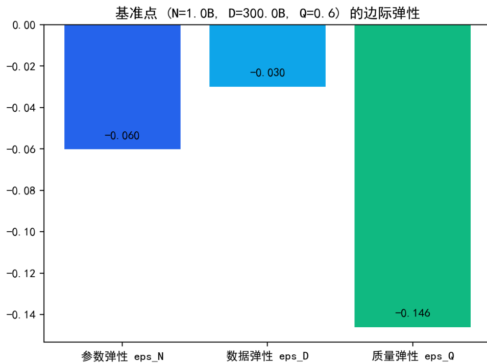
图 6.25 基准点处三个维度的损失弹性对比（质量弹性最高）。
