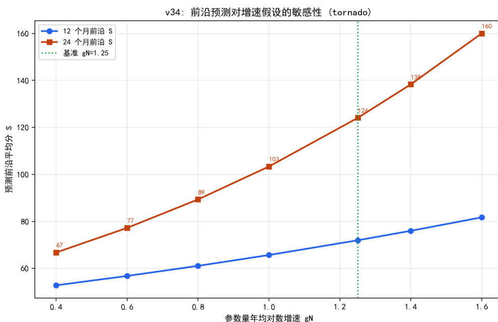
图 8.47 前沿预测对参数量增速假设 g_N 的敏感性（12/24 个月）。
