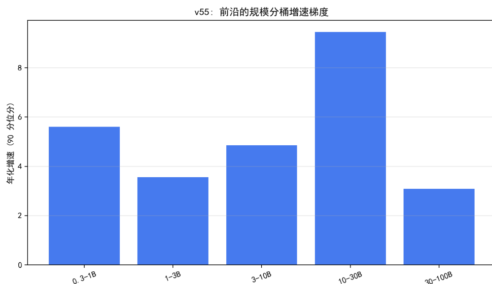
图 8.49 规模分桶的前沿年化增速：10–30B 甜点区最快，30–100B 最慢。
