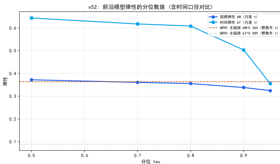
图 9.57 前沿弹性的分位数族与时间口径对比（ b_N 稳健， b_T 对口径敏感）。
