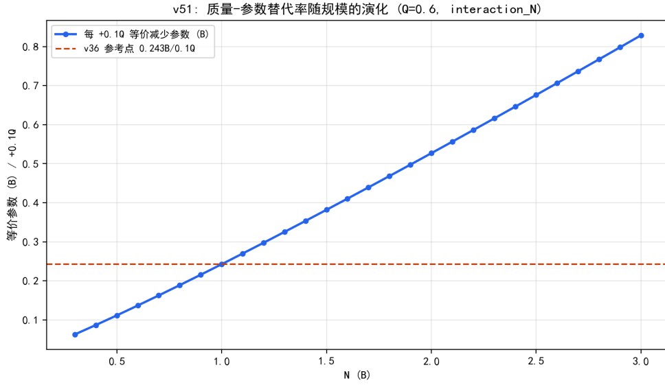
图 6.27 每 +0.1Q 等价减少的参数随规模的演化（近线性上升）。
