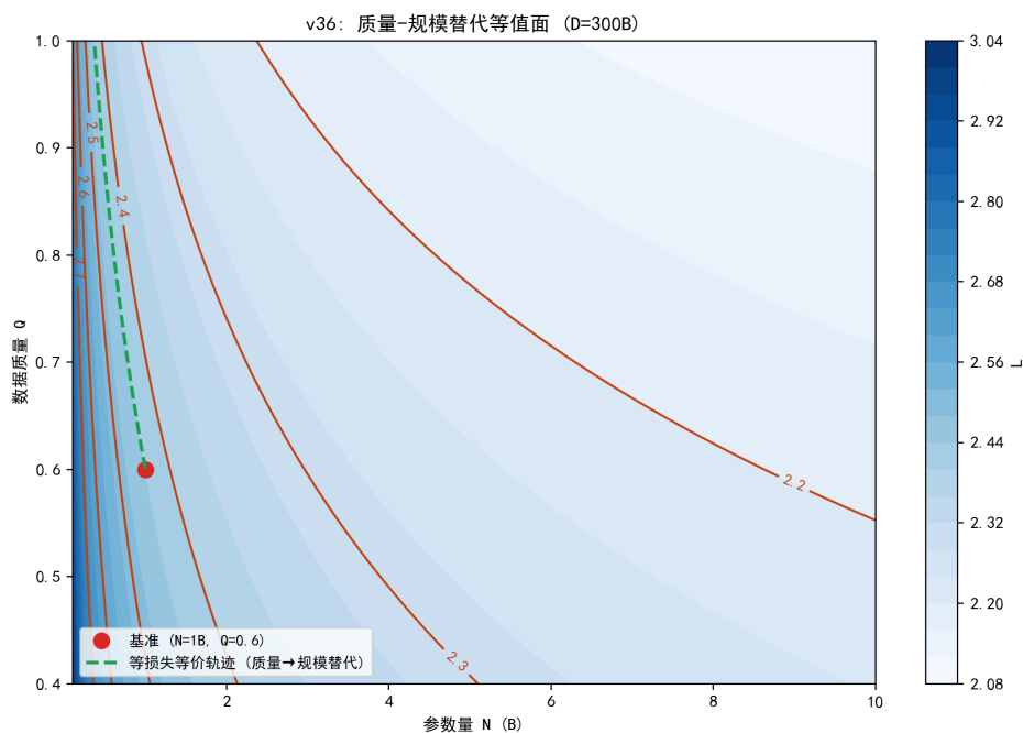
图 6.26 质量-规模替代等值面：等损失轨迹显示质量对参数的替代关系。
