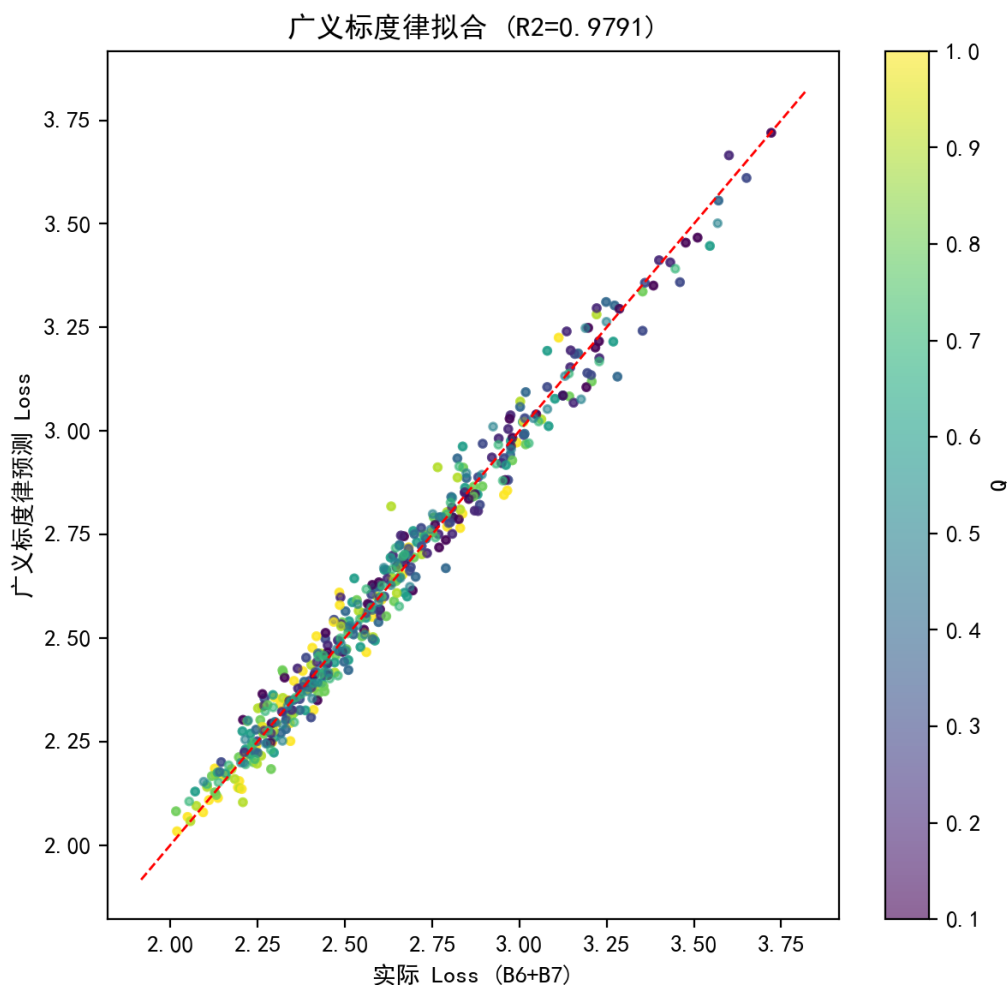
图 6.20 广义标度律在 B6+B7 数据上的拟合（质量-参数数量交互形式， R^2 = 0.979 ）。
