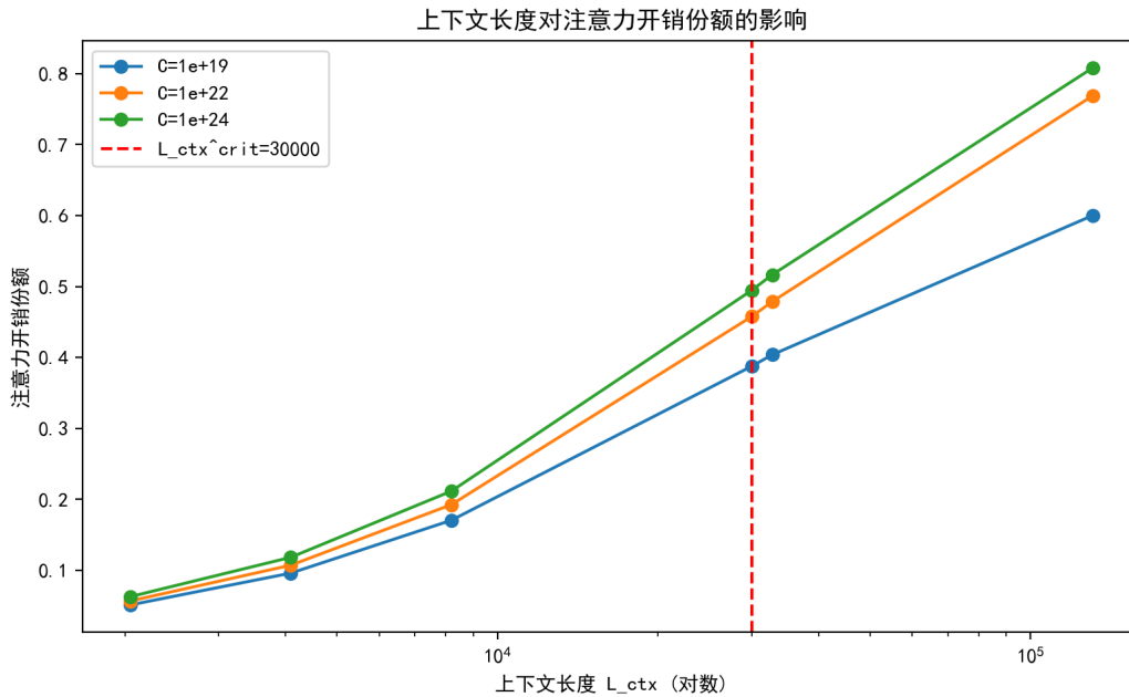
图 7.38 注意力开销份额随上下文长度的变化（红色虚线为临界点 30000）。
