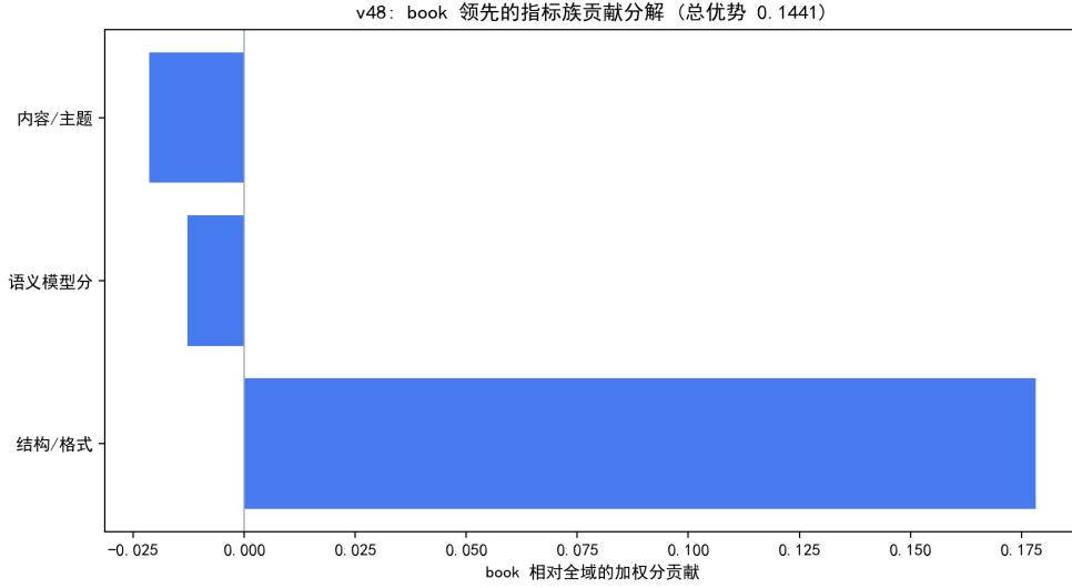
图 5.16 book 领先的指标族贡献分解：结构/格式族主导。
