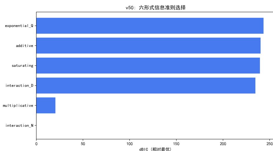
图 6.19 六种形式的 BIC/AIC 选择：interaction_N 决定性胜出。
