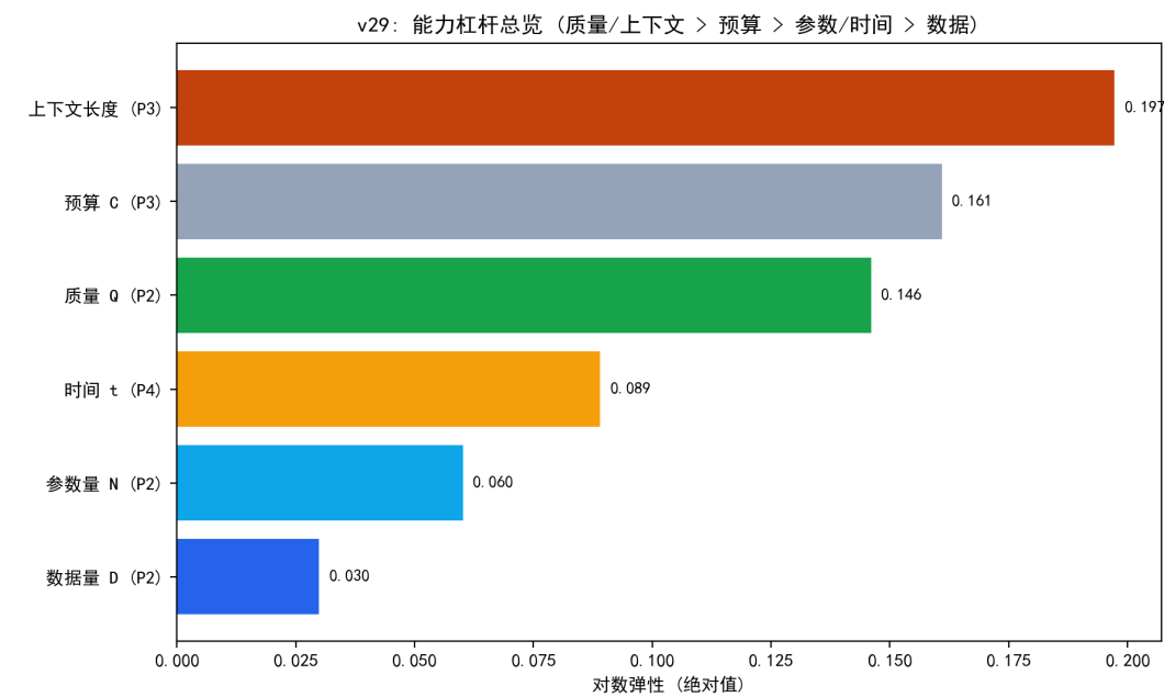
图 10.60 能力杠杆总览：各投入的对数弹性排序（质量/上下文 > 预算 > 参数/时间 > 数据）。
