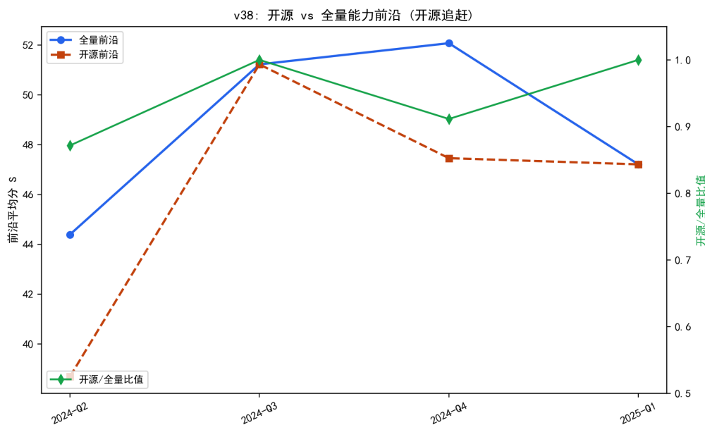
图 8.43 开源 vs 全量能力前沿：开源在 2024Q3/2025Q1 追平全量领跑。
