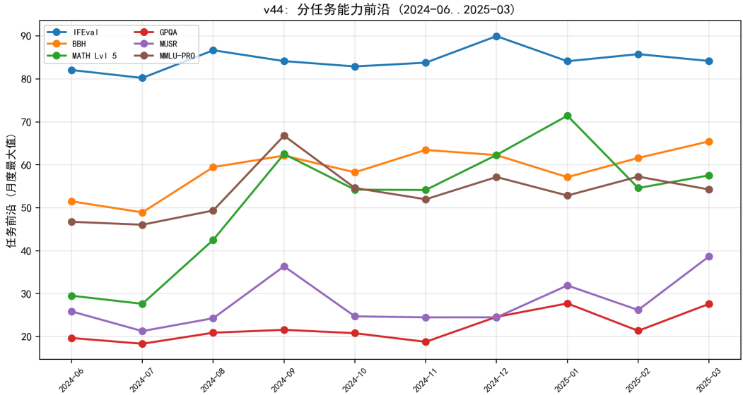
图 8.48 分任务能力前沿：推理类（MATH/GPQA/MUSR）增长快于知识/指令类。
