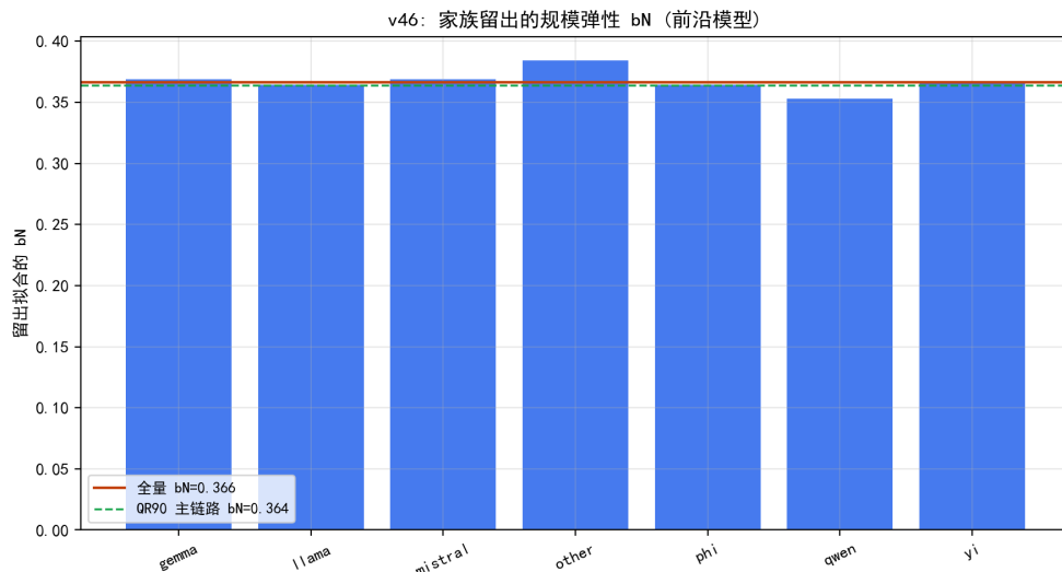
图 8.53 家族留出的规模弹性 b_N ：全家族稳定在 0.36 附近。
