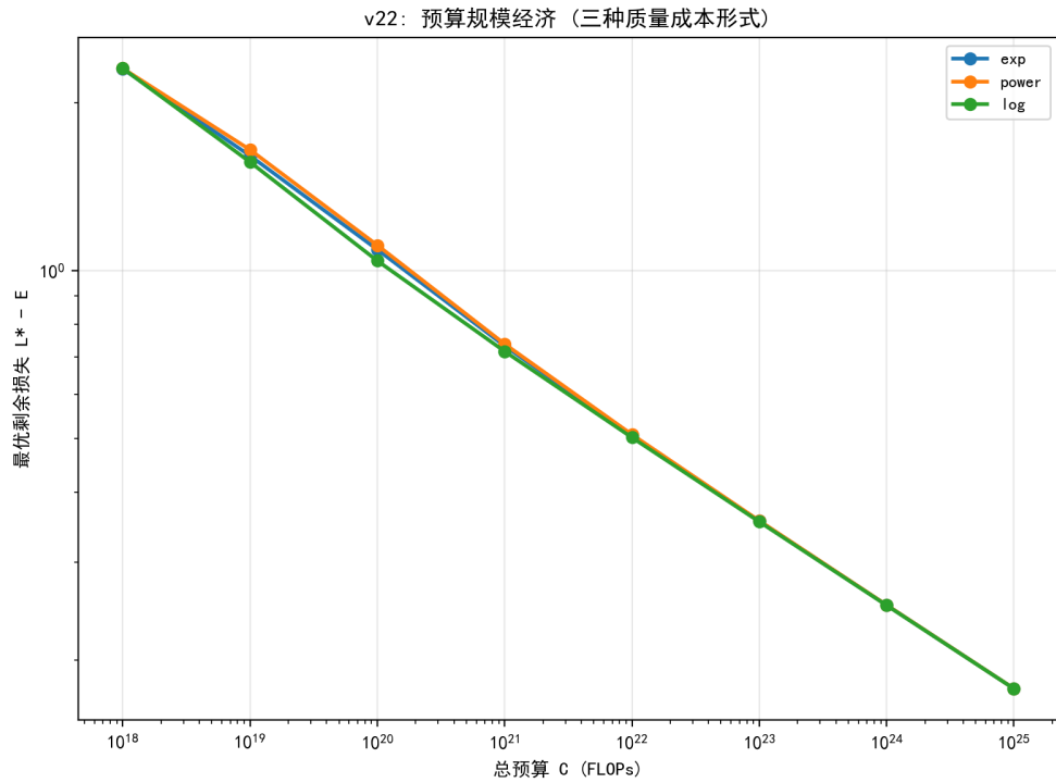
图 7.31 预算-最优损失的对数线性规律（三种质量成本形式）。
