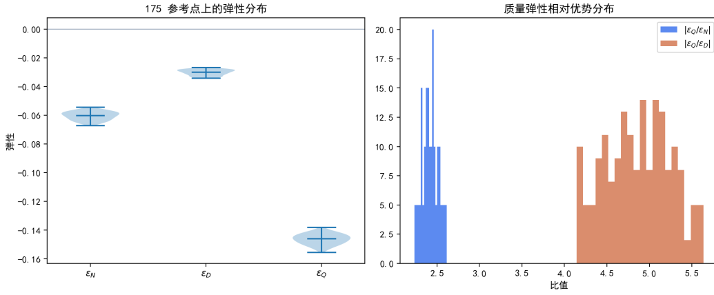
图 6.28 175 个参考点上弹性分布与质量弹性相对优势比值。
