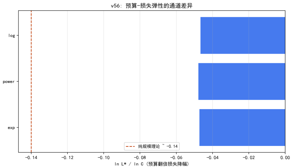
图 7.32 总损失口径的预算弹性：三形式几乎重合，低于超额口径斜率。
