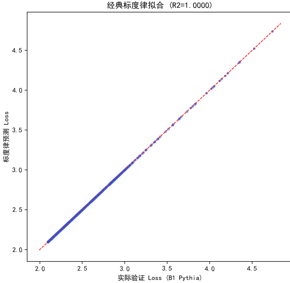
图 6.17 经典标度律在 B1 轨迹上的拟合与跨家族验证。
