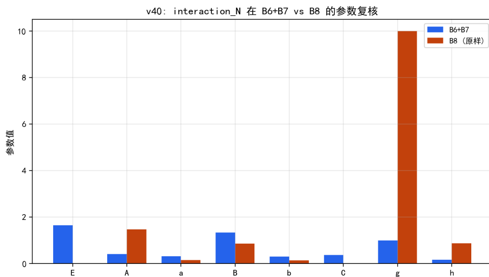
图 6.22 B8 原样 vs B6+B7 的参数对比：B8 质量项退化（ E = C = 0 ， g 撞界）。
