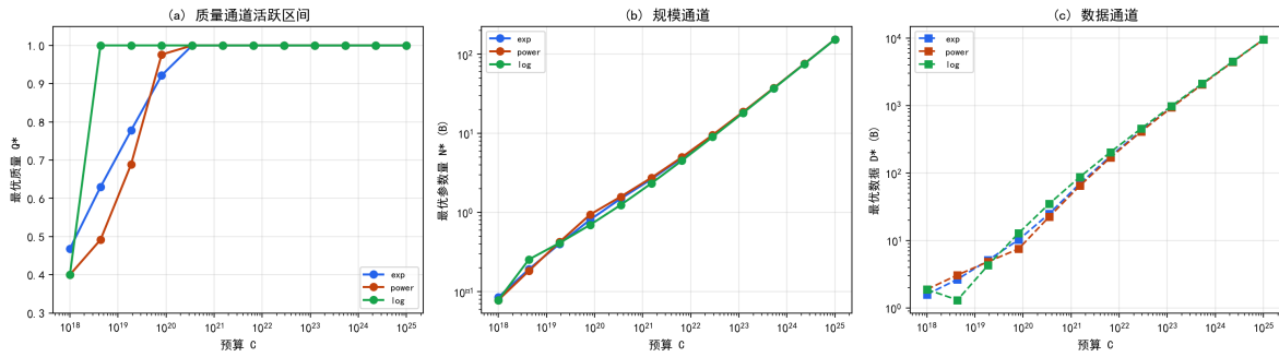
图 7.37 最优解族随预算轨迹：质量通道活跃区间由成本形式决定。
