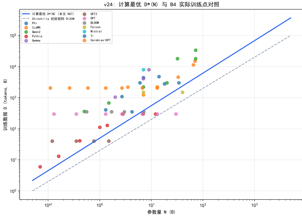
图 7.33 计算最优数据曲线 D^*(N) 、Chinchilla 经验规则与 B4 实际训练点。
