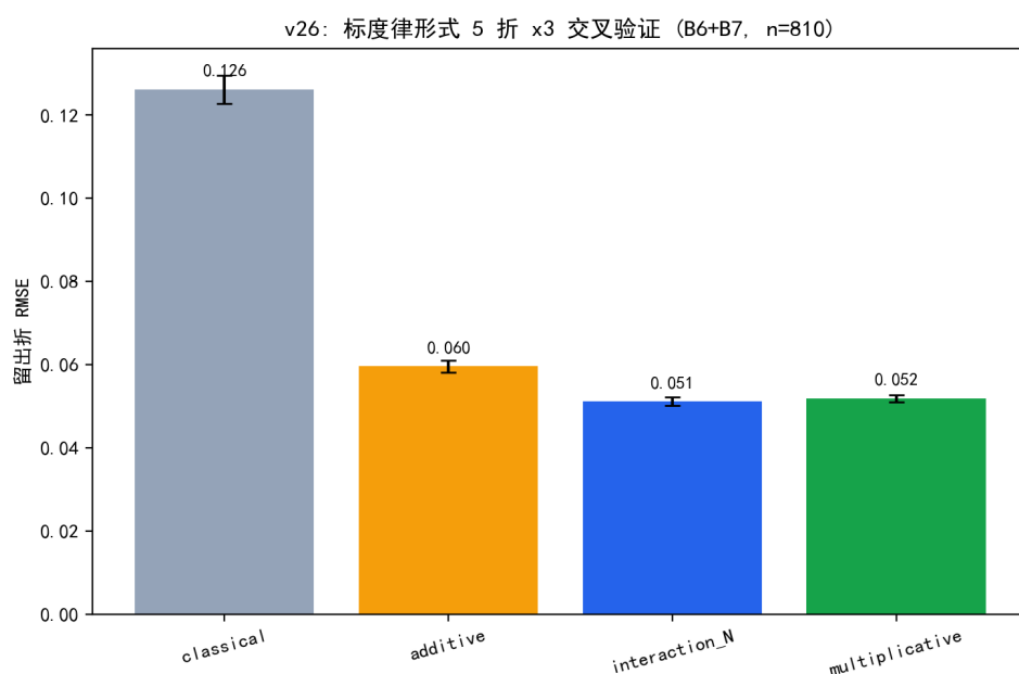
图 6.18 标度律形式 5 折交叉验证的留出 RMSE 对比。
