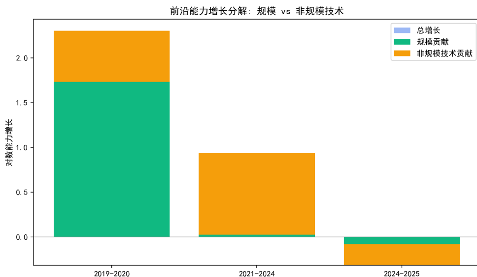
图 8.54 前沿能力增长分解：规模贡献与非规模技术贡献。
