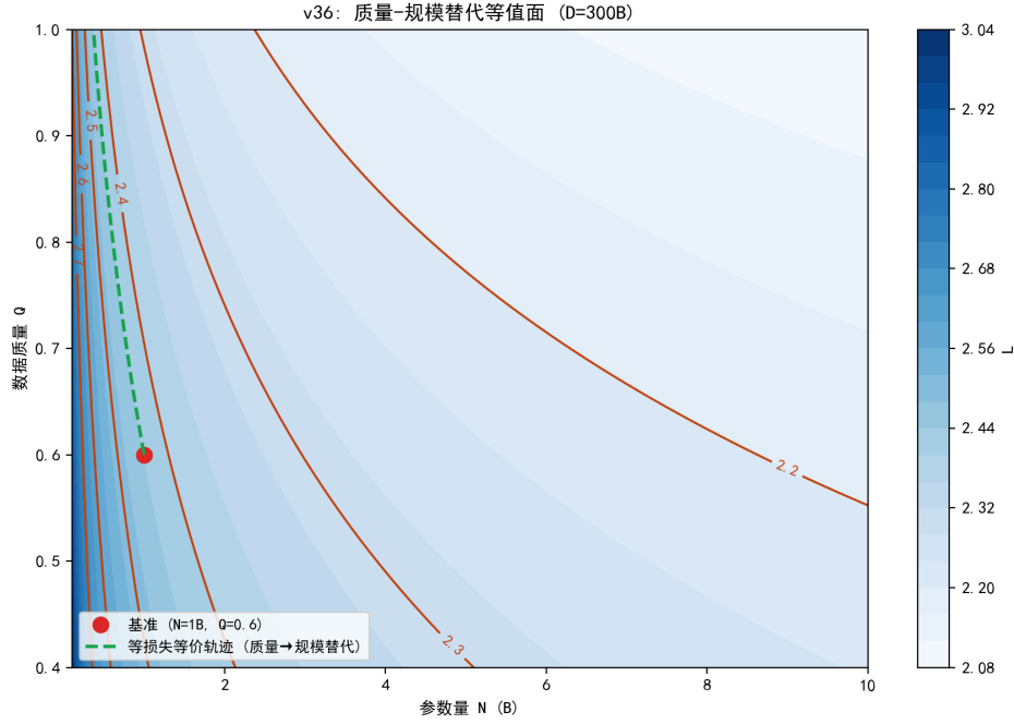
图 6.20 质量-规模替代等值面：等损失轨迹显示质量对参数的替代关系。
