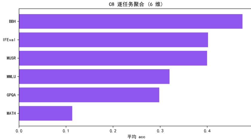
图 8.43 C8 逐任务聚合得分（6 维）。
