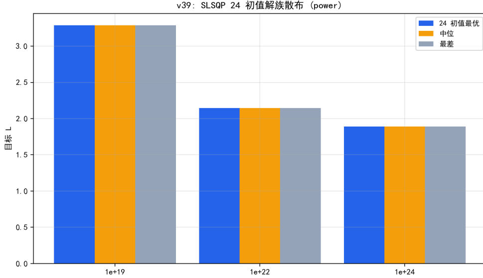
图 7.22 SLSQP 24 初值解族散布：三档预算全部初值收敛到同一最优。
