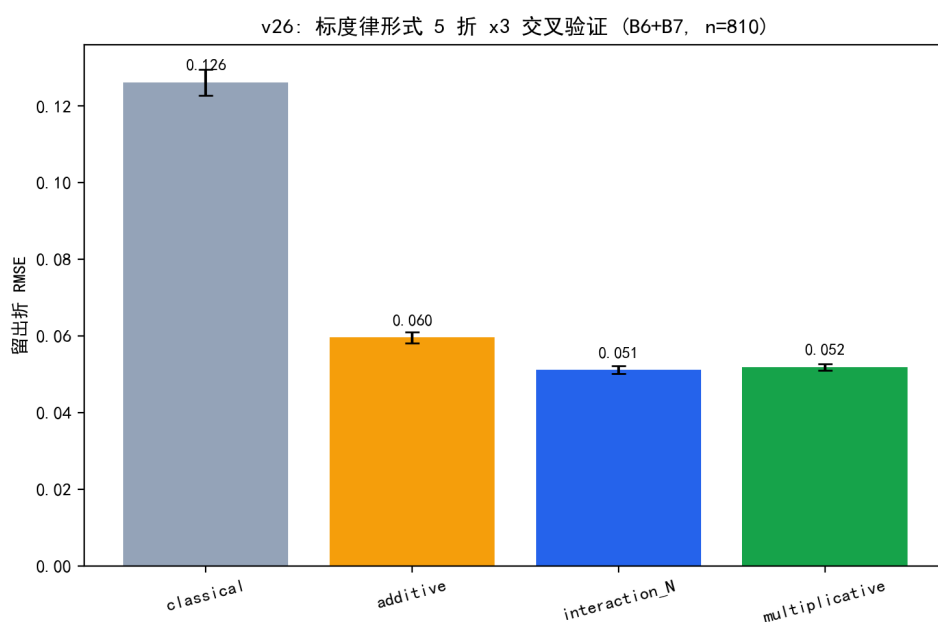
图 6.13 标度律形式 5 折交叉验证的留出 RMSE 对比。
