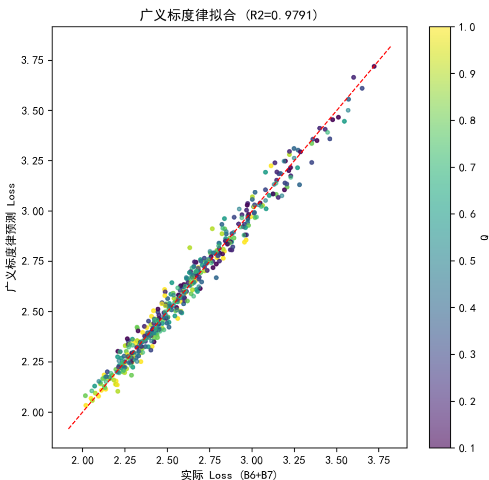
图 6.14 广义标度律在 B6+B7 数据上的拟合（质量-参数数量交互形式， R^2 = 0.979 ）。
