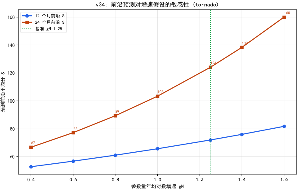
图 8.35 前沿预测对参数量增速假设 g_N 的敏感性（12/24 个月）。
