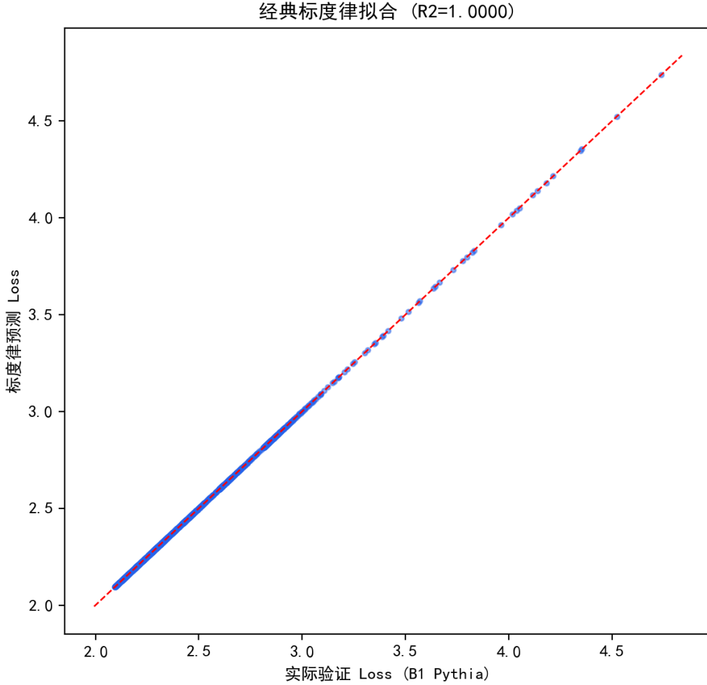
图 6.12 经典标度律在 B1 轨迹上的拟合与跨家族验证。
