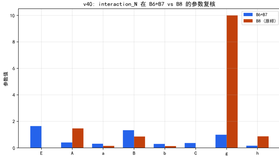
图 6.16 B8 原样 vs B6+B7 的参数对比：B8 质量项退化 ( E = C = 0 , g 撞界)。
