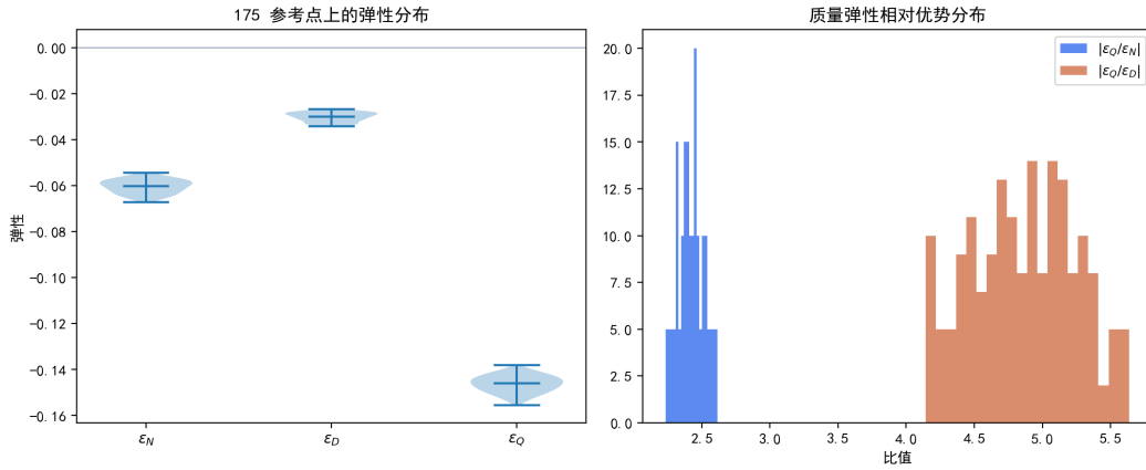
图 6.21 175 个参考点上弹性分布与质量弹性相对优势比值。
