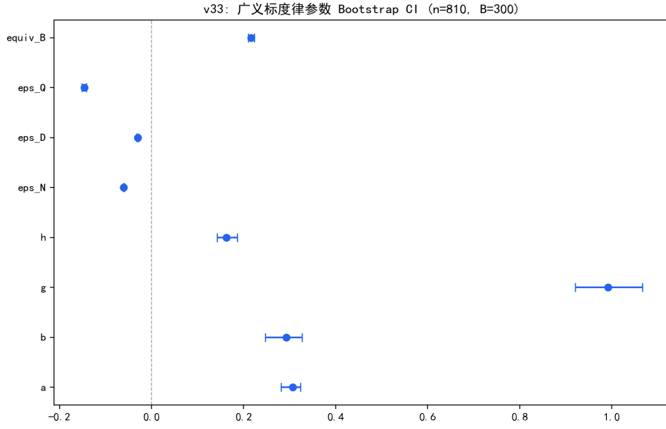
图 6.15 广义标度律参数与弹性的 Bootstrap 置信区间。
