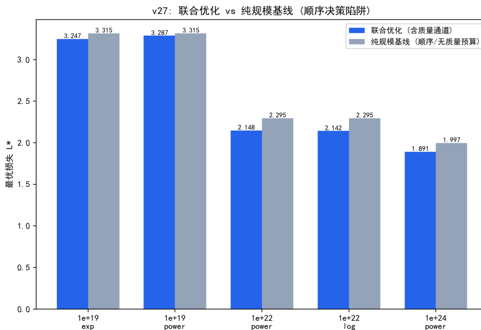
图 7.30 联合优化 vs 纯规模基线的最优损失（顺序决策陷阱：质量需预算预留）。
