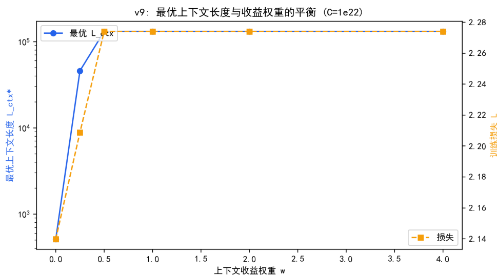
图 7.15 最优上下文长度与收益权重 w 的平衡 ( C = 10^{22} )。
