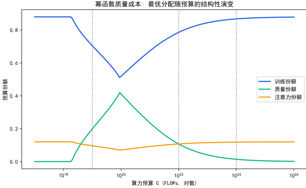
图 7.12 幂函数质量成本下最优成本份额随预算的结构性演变（竖线为三档预算）。
