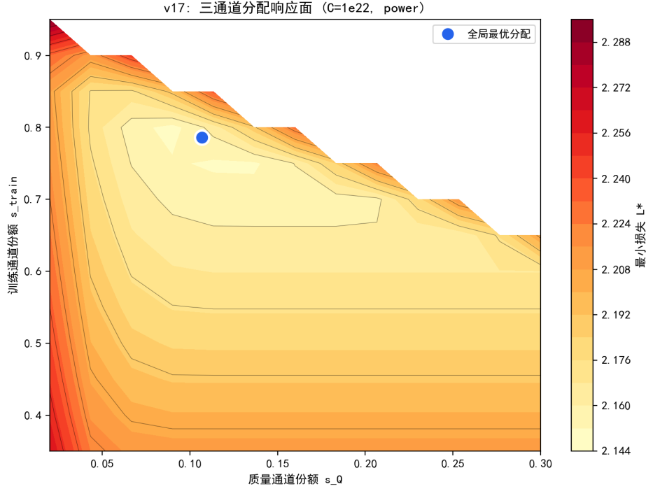
图 7.16 三通道分配响应面 ( C = 10^{22} , 幂成本; 蓝点为全局最优分配)。
