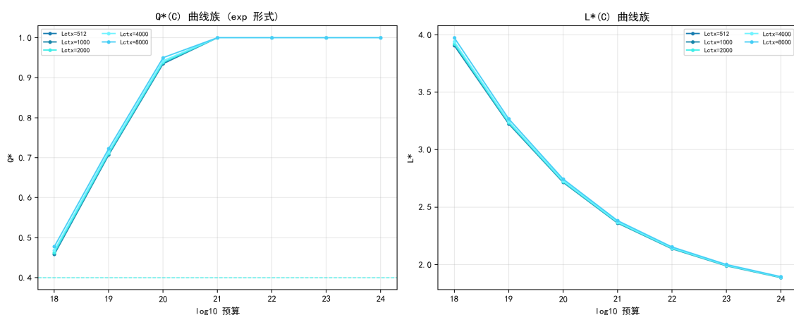
图 7.43 上下文长度 \times 预算响应面： L^* 路径几乎不随 L_{ctx} 移动。
