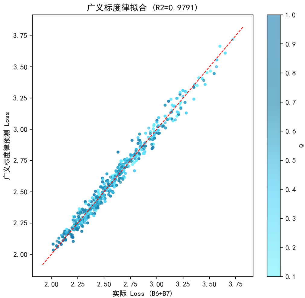
图 6.27 广义标度律在 B6+B7 数据上的拟合（质量-参数量交互形式， R^2 = 0.979 ）。
