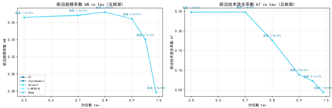
图 8.59 分位数族 \times 五框架：每个 \tau 上五框架一致； b_T 随 \tau 单调递减、 b_N 峰后回落。
