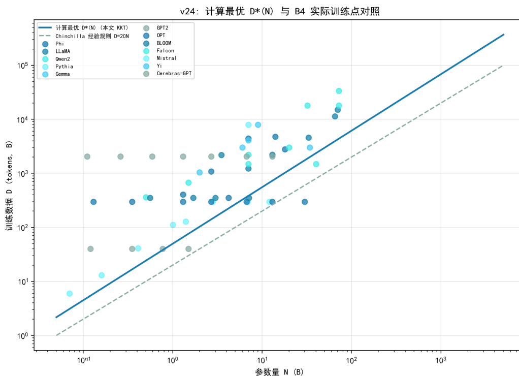
图 7.43 计算最优数据曲线 D^*(N) 、Chinchilla 经验规则与 B4 实际训练点。
