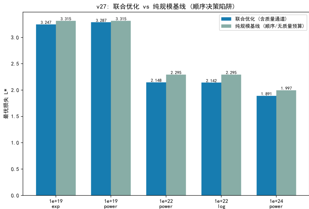
图 7.50 联合优化 vs 纯规模基线的最优损失 (顺序决策陷阱: 质量需预算预留)。
