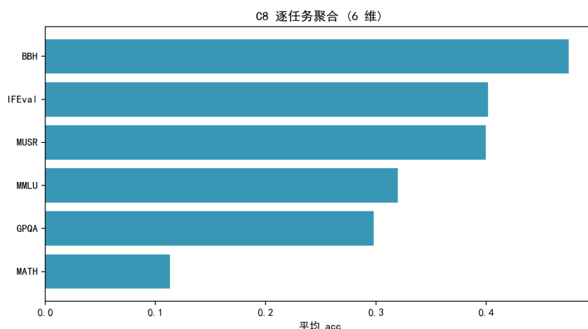
图 8.74 C8 逐任务聚合得分（6 维）。
