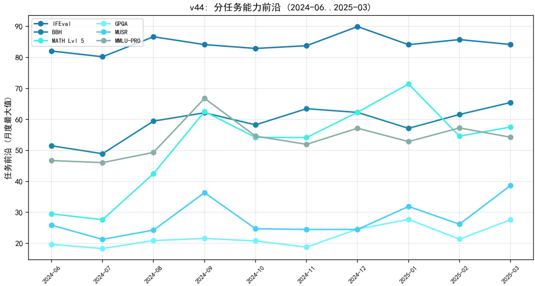
图 8.64 分任务能力前沿：推理类（MATH/GPQA/MUSR）增长快于知识/指令类。
