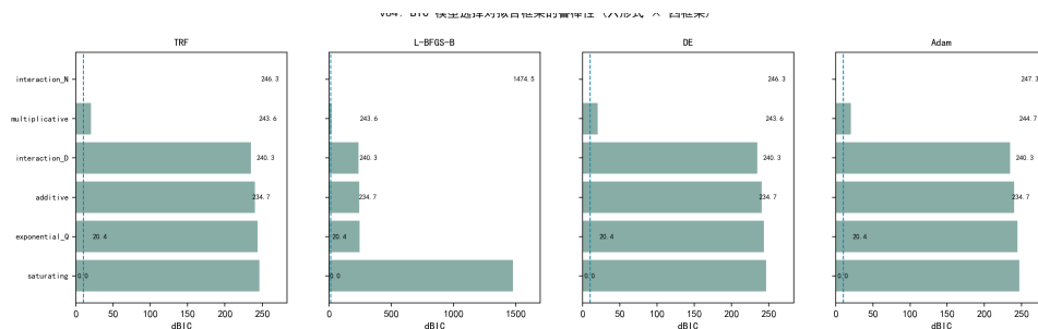
图 6.23 拟合框架鲁棒性: 四种独立拟合框架 (TRF/L-BFGS-B/DE/Adam) 下的 BIC 排序完全一致 (虚线为 \Delta\text{BIC} = 10 决定性阈值)。
