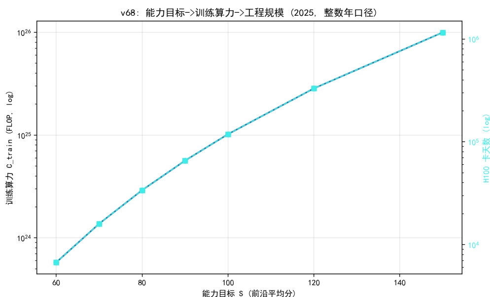
图 8.61 能力目标 → 训练算力 (对数轴)：S=90 约需 6.6 万卡天。
