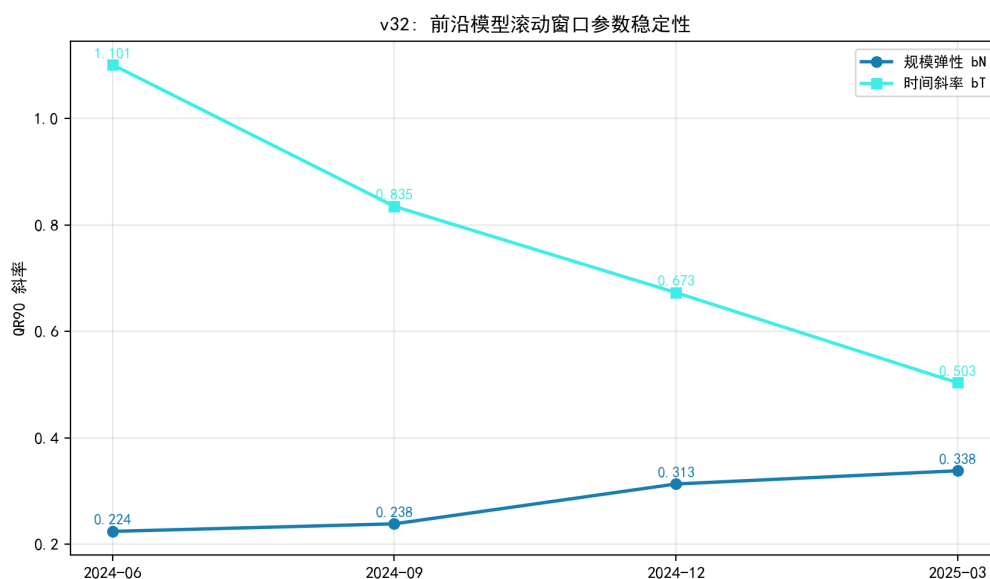
图 8.68 前沿 QR90 滚动窗口参数：规模弹性上升、时间斜率持续下降。
