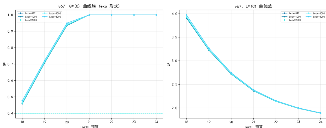
图 7.42 上下文长度 \times 预算响应面： L^* 路径几乎不随 L_{ctx} 移动。
