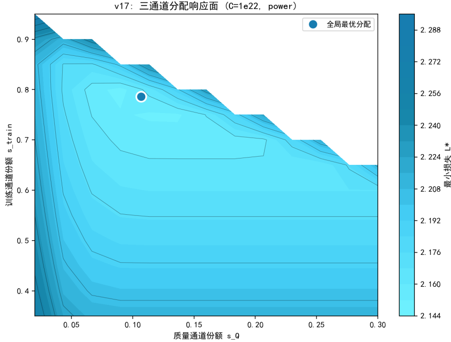
图 7.52 三通道分配响应面 ( C = 10^{22} , 幂成本；蓝点为全局最优分配)。
