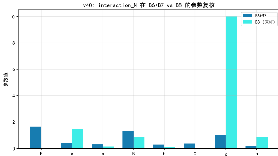
图 6.28 B8 原样 vs B6+B7 的参数对比：B8 质量项退化（ E = C = 0 ， g 撞界）。
