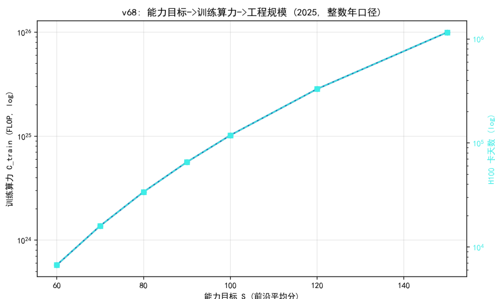
图 8.60 能力目标 \rightarrow 训练算力（对数轴）： S=90 约需 6.6 万卡天。
