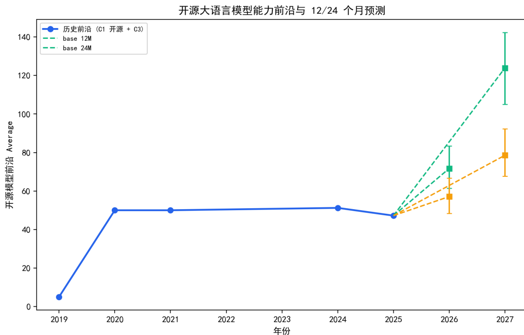
图 8.14 开源模型能力前沿（历史点）与 12/24 个月预测（基础/放缓情景，90% 区间）。
