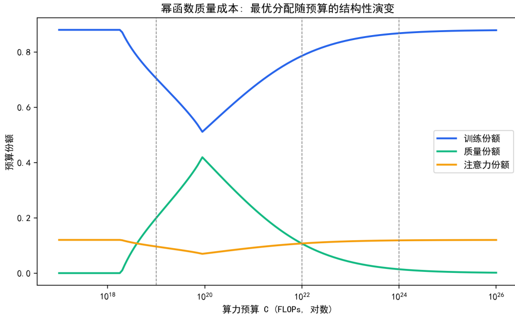
图 7.29 幂函数质量成本下最优成本份额随预算的结构性演变（竖线为三档预算）。
