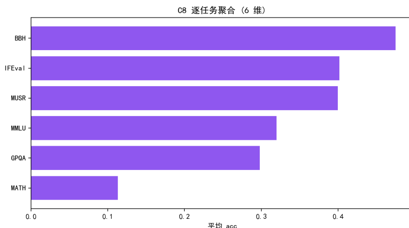
图 8.46 C8 逐任务聚合得分（6 维）。
