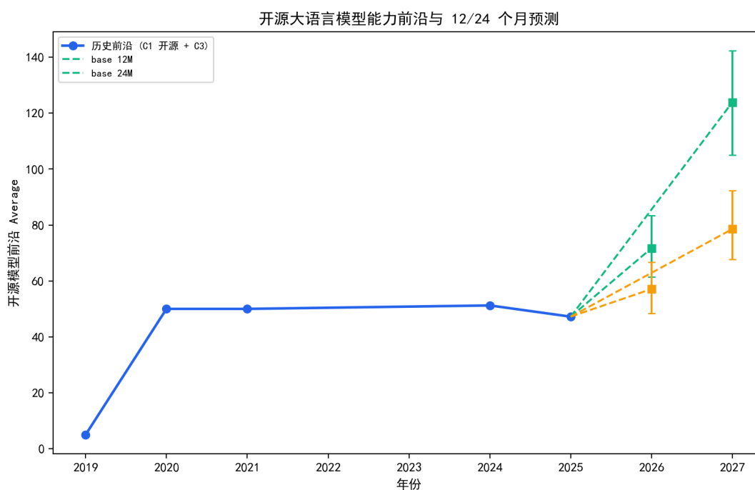
图 8.41 开源模型能力前沿（历史点）与 12/24 个月预测（基础/放缓情景，90% 区间）。
