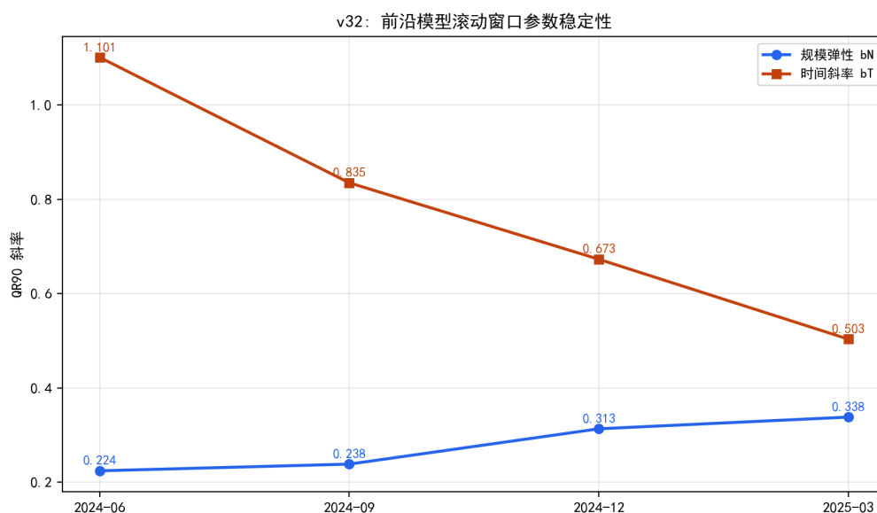
图 8.40 前沿 QR90 滚动窗口参数：规模弹性上升、时间斜率持续下降。
