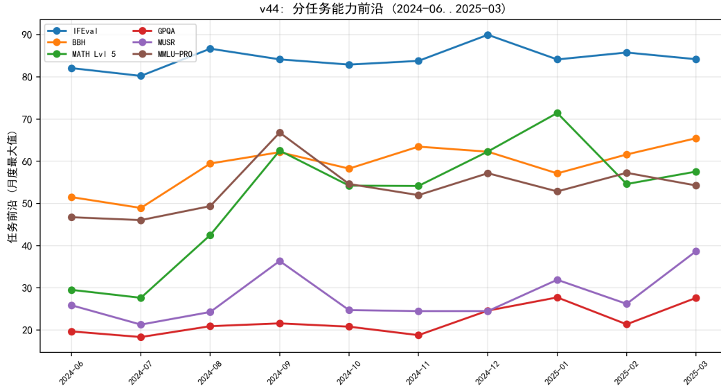
图 8.39 分任务能力前沿：推理类（MATH/GPQA/MUSR）增长快于知识/指令类。
