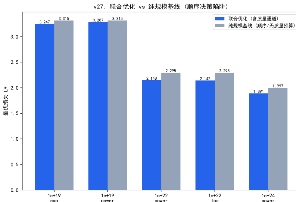
图 7.33 联合优化 vs 纯规模基线的最优损失（顺序决策陷阱：质量需预算预留）。
