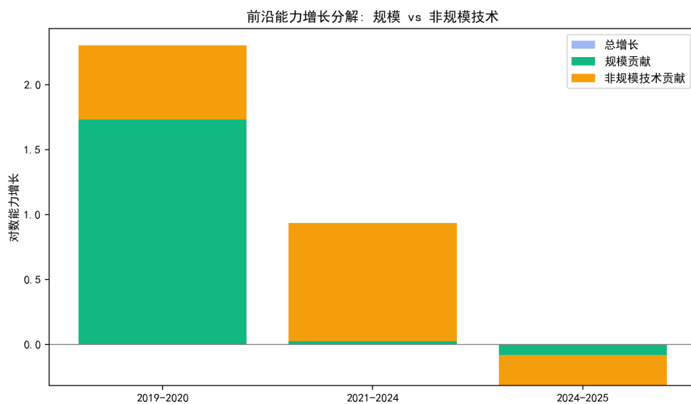
图 8.44 前沿能力增长分解：规模贡献与非规模技术贡献。
