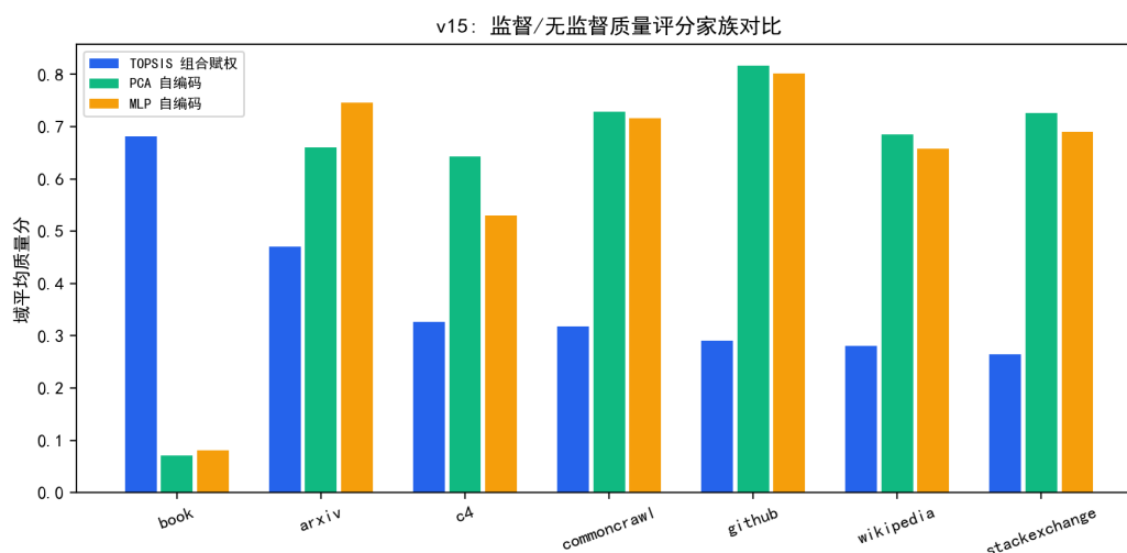
图 9.48 TOPSIS 组合赋权与自编码典型性评分的域级对照（方向相反）。
