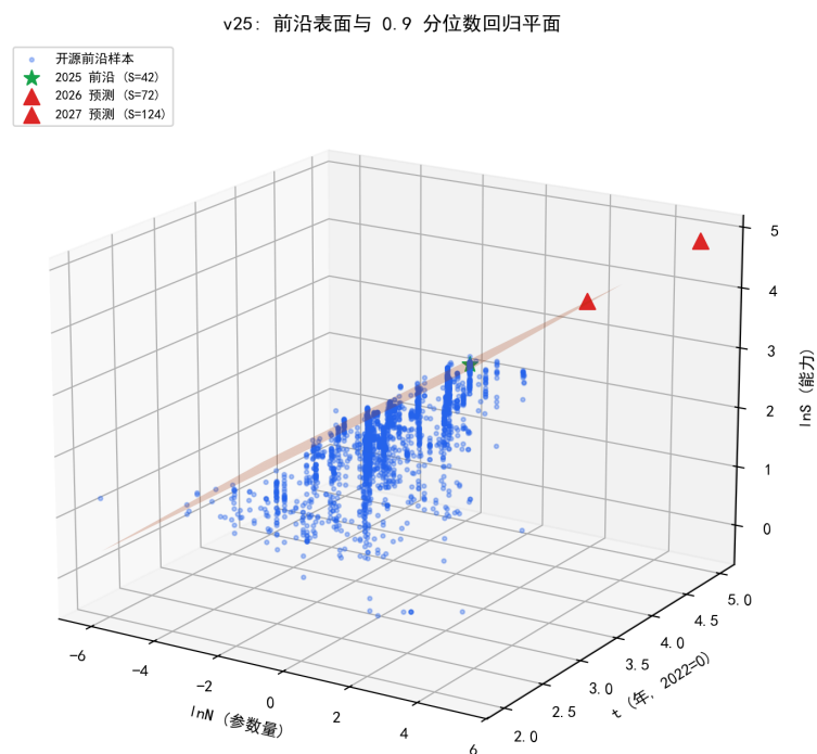
图 8.42 能力前沿 3D 表面与 0.9 分位数回归平面（星标 = 2025 前沿，三角 = 预测点）。
