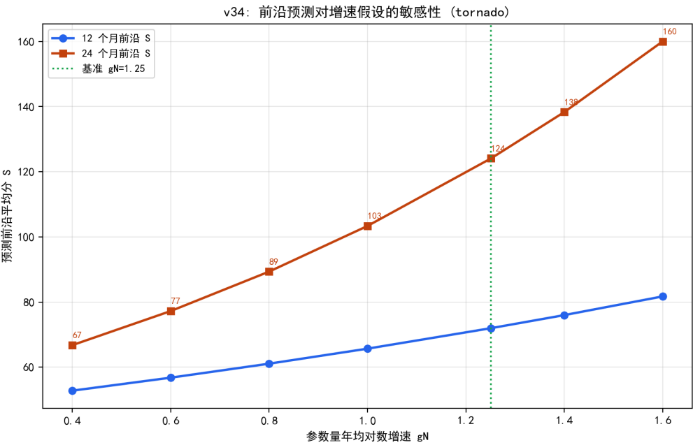
图 8.38 前沿预测对参数量增速假设 g_N 的敏感性（12/24 个月）。
