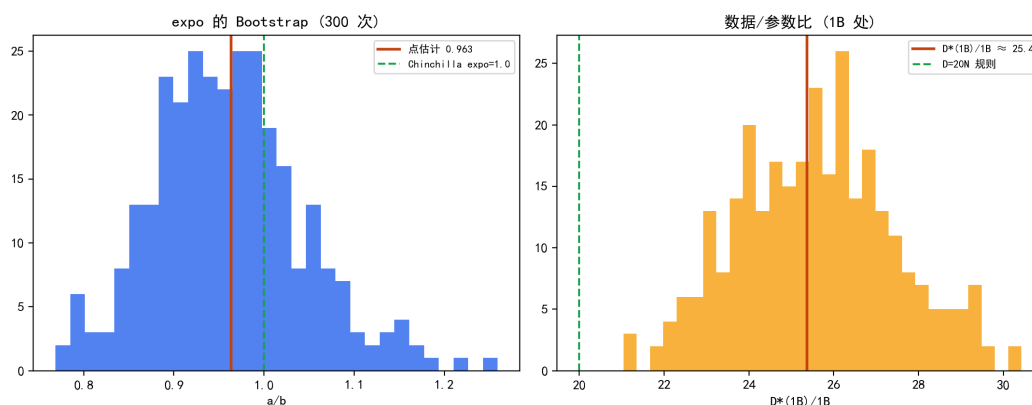
图 7.28 D^*(N) 参数 Bootstrap: 指数 CI 含 1.0, 常数 CI 高于 D = 20N 。
