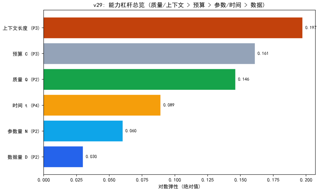
图 10.49 能力杠杆总览：各投入的对数弹性排序（质量/上下文 > 预算 > 参数/时间 > 数据）。
