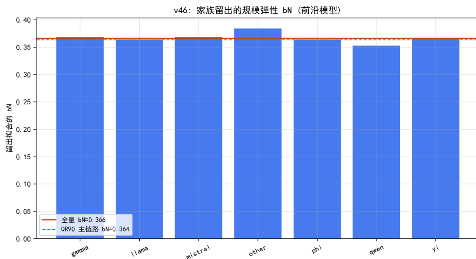
图 8.43 家族留下的规模弹性 b_N ：全家族稳定在 0.36 附近。
