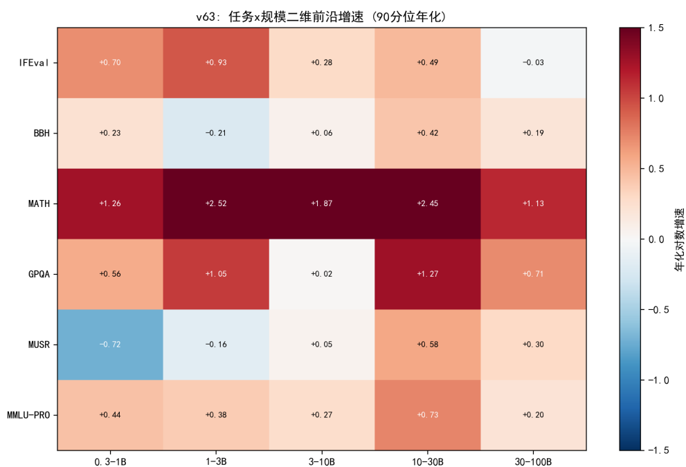
图 8.58 任务 × 规模二维前沿增速：MATH/GPQA 在 1-3B 与 10-30B 双峰。
