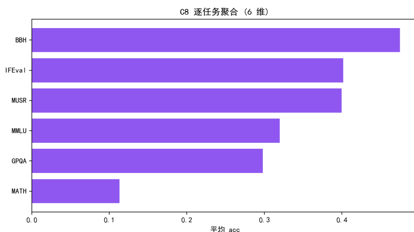
图 8.66 C8 逐任务聚合得分 (6 维)。
