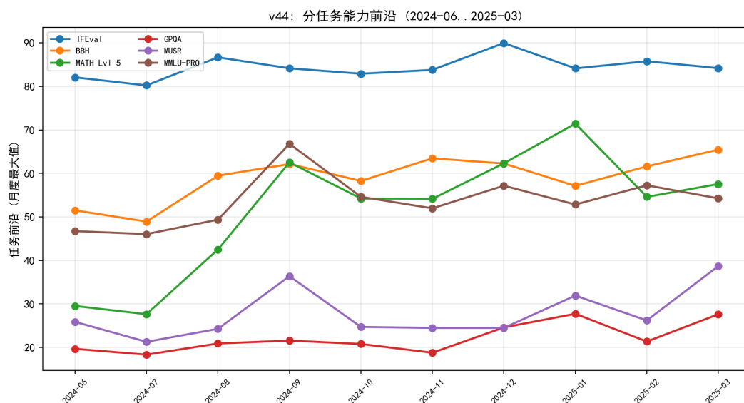
图 8.56 分任务能力前沿：推理类（MATH/GPQA/MUSR）增长快于知识/指令类。
