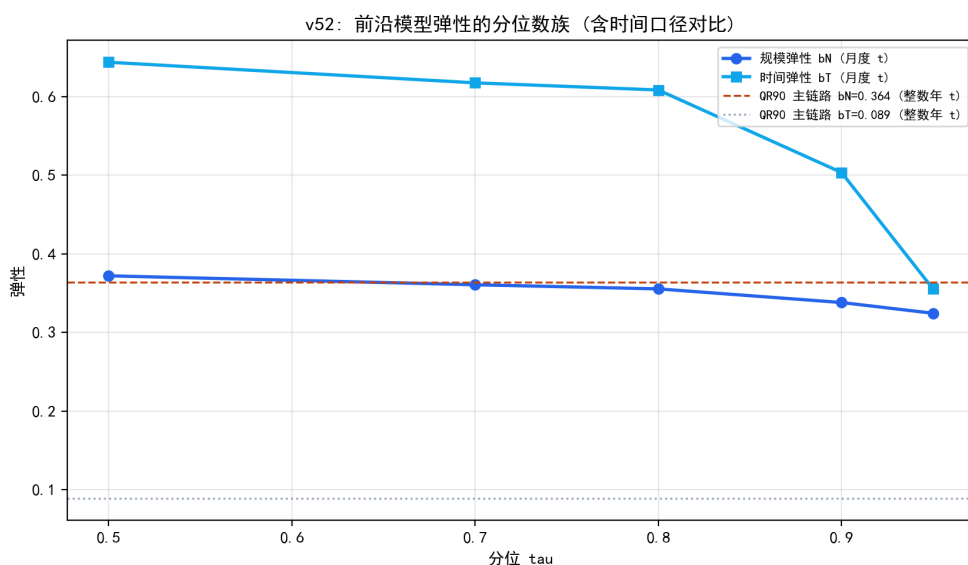
图 9.67 前沿弹性的分位数族与时间口径对比（bN 稳健，bT 对口径敏感）。
