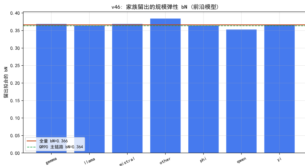
图 8.63 家族留出的规模弹性 b_N ：全家族稳定在 0.36 附近。
