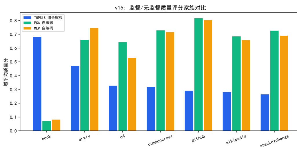
图 9.69 TOPSIS 组合赋权与自编码典型性评分的域级对照（方向相反）。
