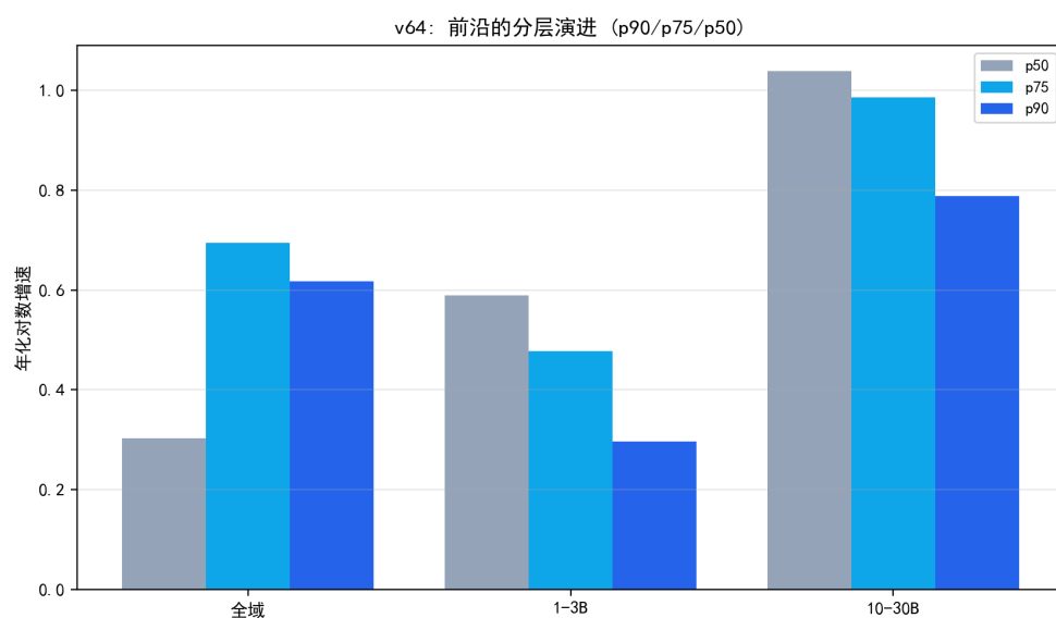
图 8.59 分层演进：全域顶层分化 ( p_{90}/p_{50} \approx 2 )，段内普惠 ( p_{50} 快于 p_{90} )。
