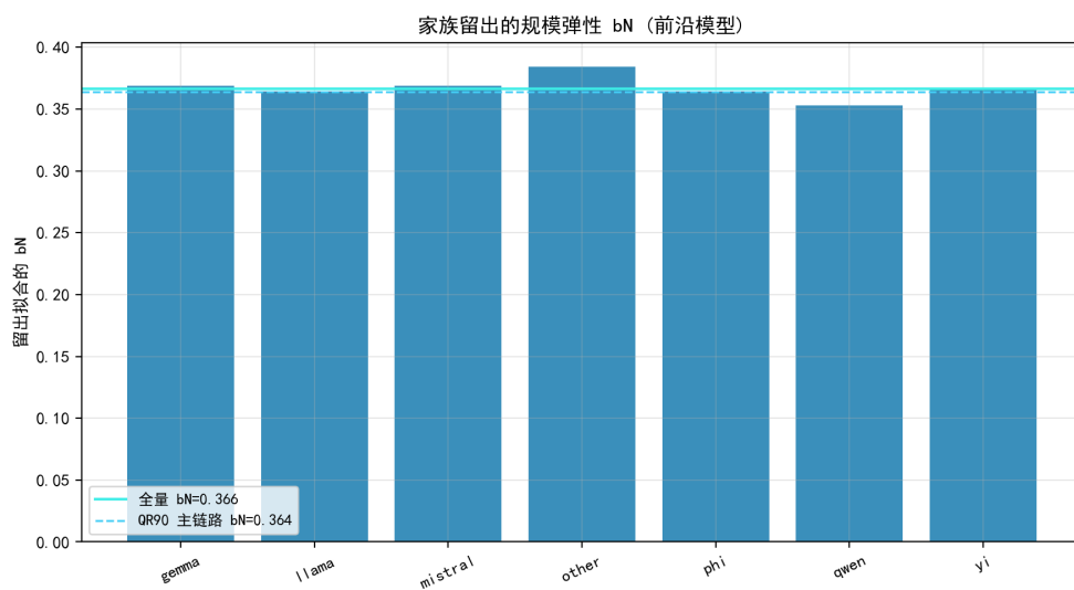
图 8.73 家族留出的规模弹性 b_N ：全家族稳定在 0.36 附近。
