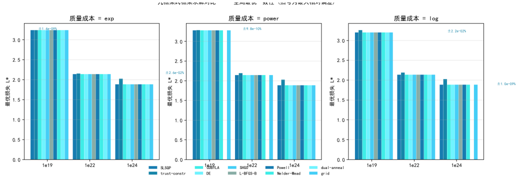
图 7.39 九框架求解对比：SLSQP/COBYLA/DE/SHGO/L-BFGS-B/Powell/Nelder-Mead/ 双退火/网格在 9 实例上一致到 10^{-6} 量级（括号为九路径最大相对偏差），trust-constr 内点法在边界角点最优处失稳。
