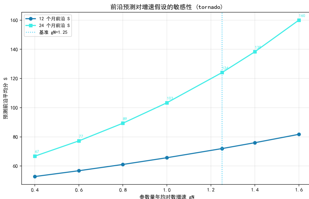
图 8.65 前沿预测对参数量增速假设 g_N 的敏感性（12/24 个月）。
