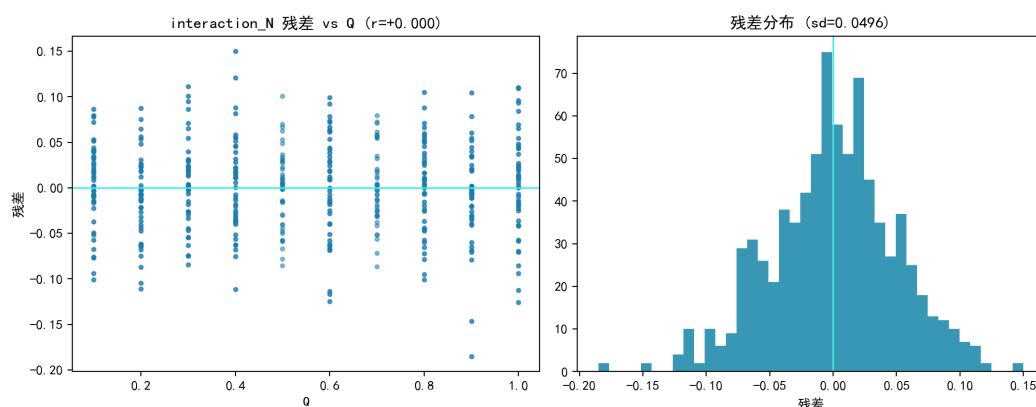
图 6.26 interaction_N 残差诊断：与 Q 无相关、分布近对称。
