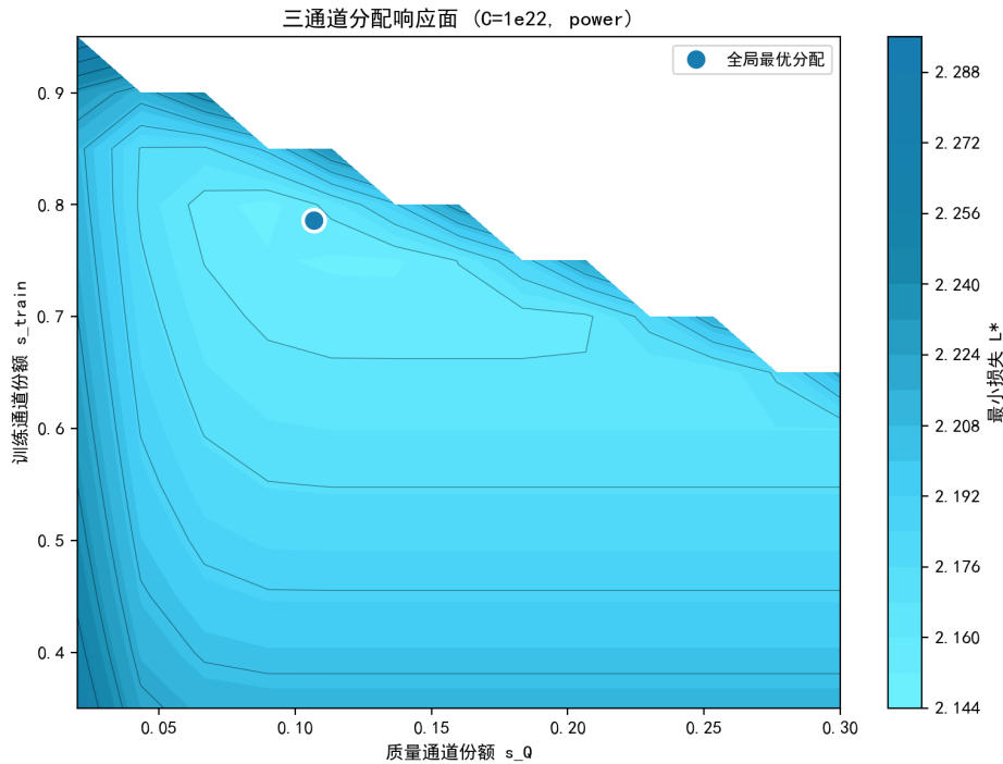
图 7.54 三通道分配响应面 ( C = 10^{22} , 幂成本; 蓝点为全局最优分配)。
