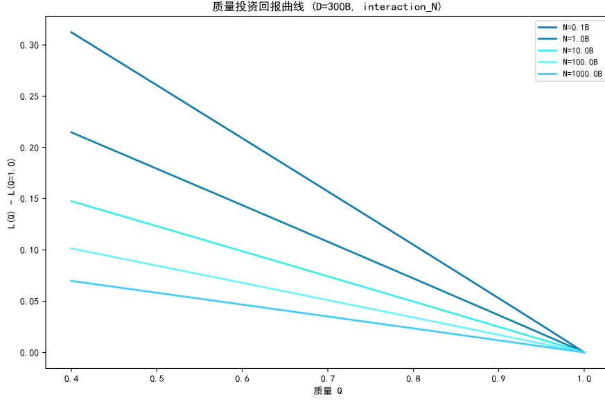
图 6.33 质量投资回报曲线 ( D = 300B ): L(Q) 相对 L(Q = 1) 随 N 变化。
