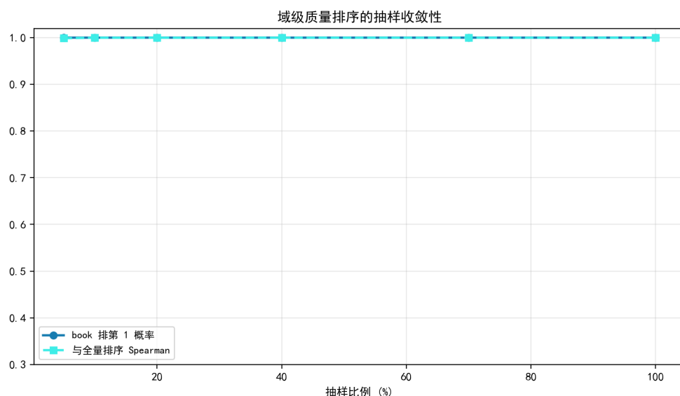
图 5.15 域级质量排序的抽样收敛性：book 在 5% 抽样下仍 100% 保持第 1。
