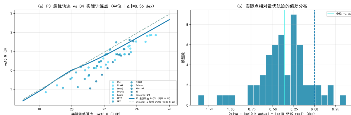
图 7.55 闭环对照：P3 最优轨迹与 B4 实际训练点（左）；偏差分布（右）。中位偏差 0.36 dex，优于 Chinchilla 规则 30%。
