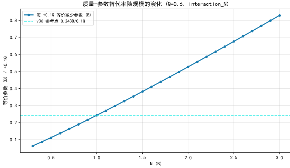
图 6.36 每 +0.1Q 等价减少的参数随规模的演化（近线性上升）。
