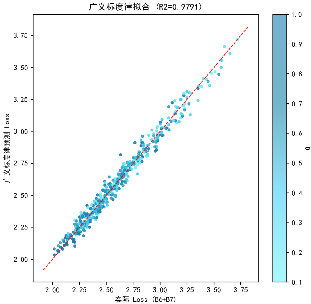
图 6.29 广义标度律在 B6+B7 数据上的拟合（质量-参数量交互形式， R^2 = 0.979 ）。
