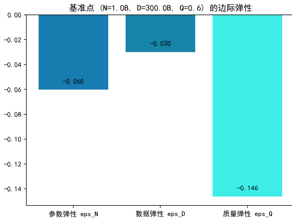
图 6.34 基准点处三个维度的损失弹性对比（质量弹性最高）。
