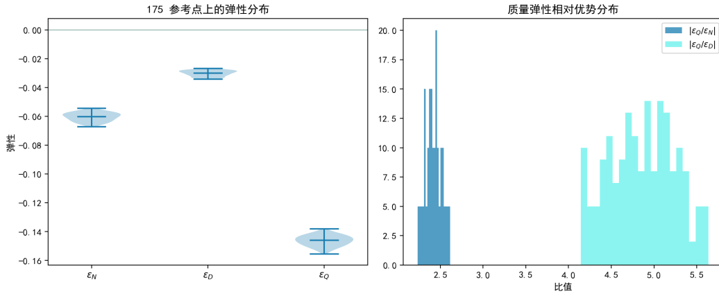
图 6.37 175 个参考点上弹性分布与质量弹性相对优势比值。
