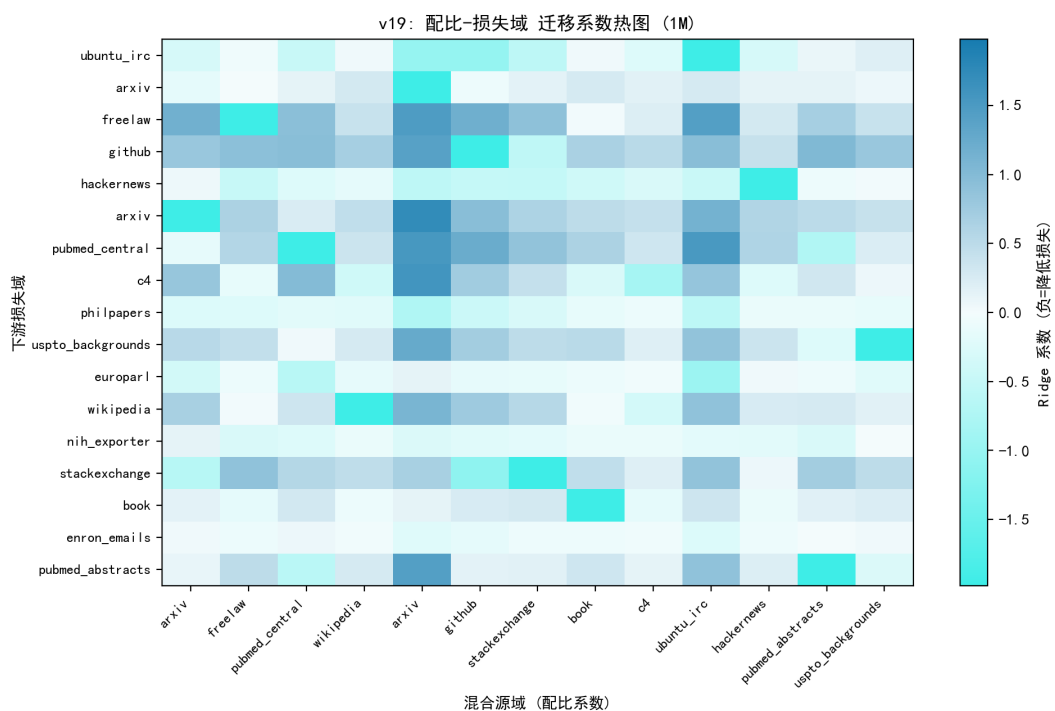
图 5.10 配比源域 \times 损失域迁移系数热图 (1M 尺度, 负值 = 压低损失)。
