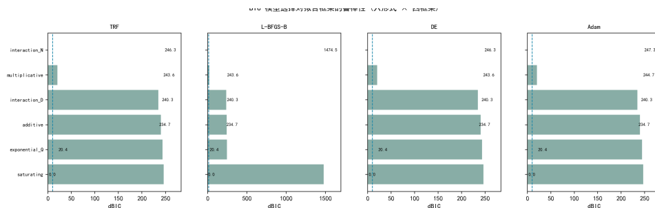
图 6.23 拟合框架鲁棒性：四种独立拟合框架 (TRF/L-BFGS-B/DE/Adam) 下的 BIC 排序完全一致 (虚线为 \Delta BIC = 10 决定性阈值)。
