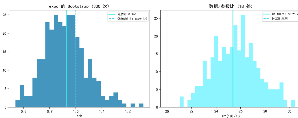
图 7.44 D^*(N) 参数 Bootstrap: 指数 CI 含 1.0, 常数 CI 高于 D = 20N 。
