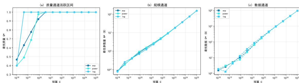
图 7.47 最优解族随预算轨迹：质量通道活跃区间由成本形式决定。
