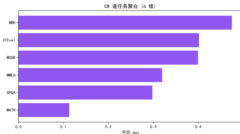
图 8.15 C8 逐任务聚合得分（6 维）。
