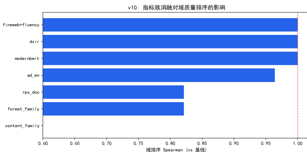
图 9.16 指标族消融对域质量排序的影响（红虚线为完全一致）。
