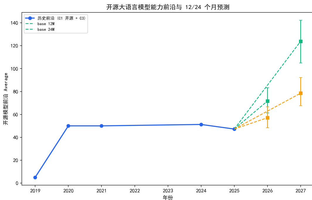
图 8.12 开源模型能力前沿（历史点）与 12/24 个月预测（基础/放缓情景，90% 区间）。
