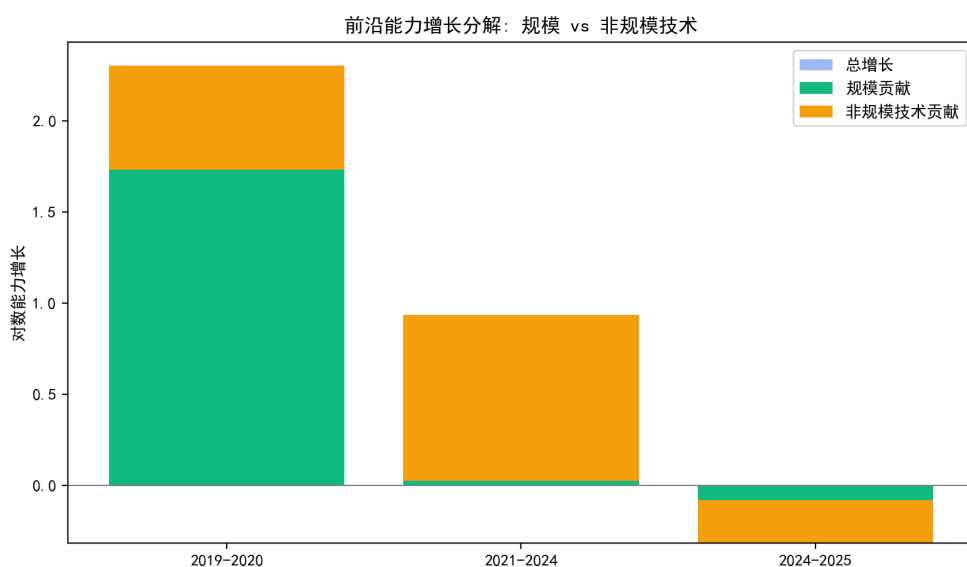
图 8.13 前沿能力增长分解：规模贡献与非规模技术贡献。
