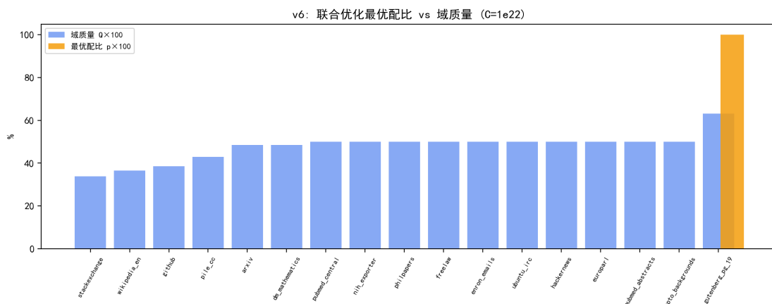
图 7.10 联合优化最优配比与域质量对比 ( C = 10^{22} ): 配比向最高质量域（小说）集中。
