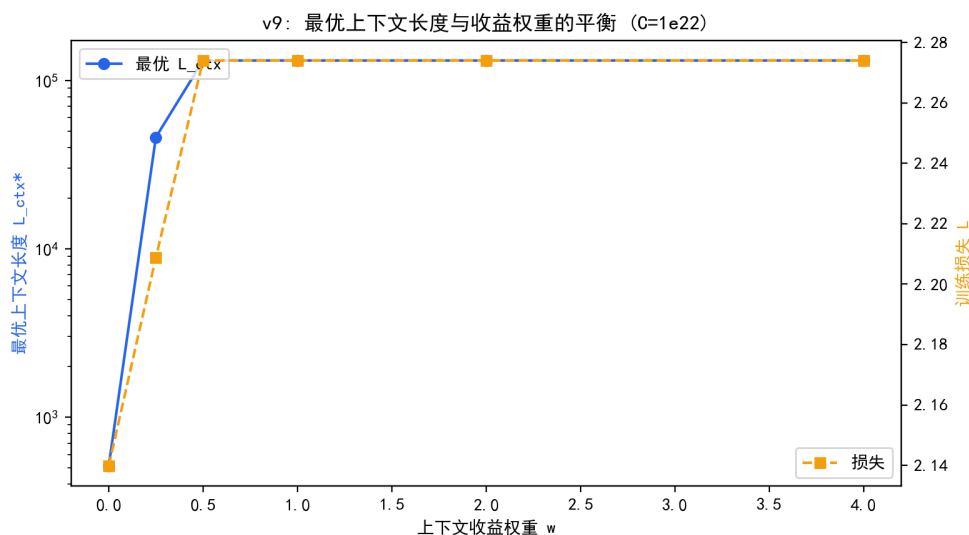
图 7.11 最优上下文长度与收益权重 w 的平衡 ( C = 10^{22} )。
