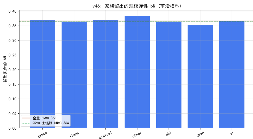
图 8.46 家族留下的规模弹性 b_N ：全家族稳定在 0.36 附近。
