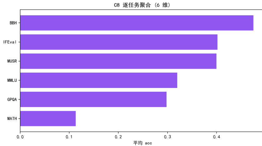
图 8.49 C8 逐任务聚合得分（6 维）。
