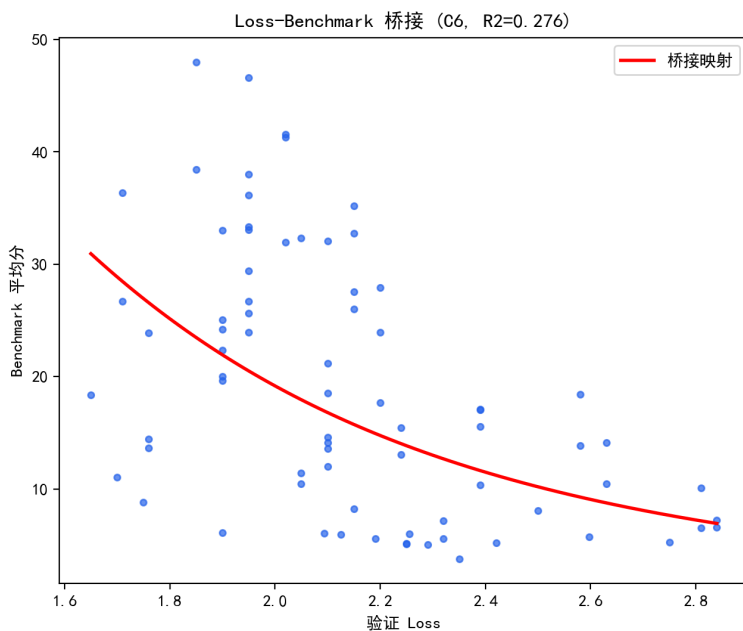
图 8.48 Loss-Benchmark 桥接映射（C6，75 个模型）。
