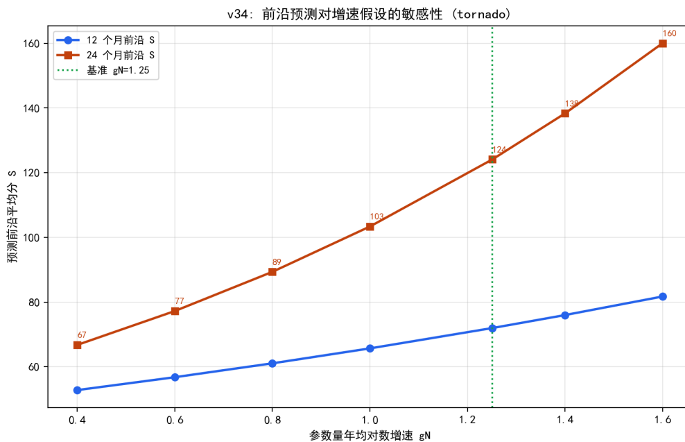
图 8.41 前沿预测对参数量增速假设 g_N 的敏感性（12/24 个月）。
