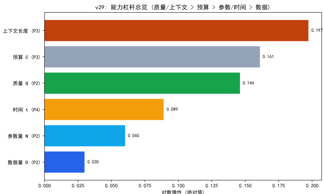
图 10.53 能力杠杆总览：各投入的对数弹性排序（质量/上下文 > 预算 > 参数/时间 > 数据）。
