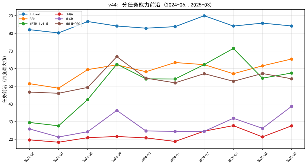
图 8.42 分任务能力前沿：推理类（MATH/GPQA/MUSR）增长快于知识/指令类。
