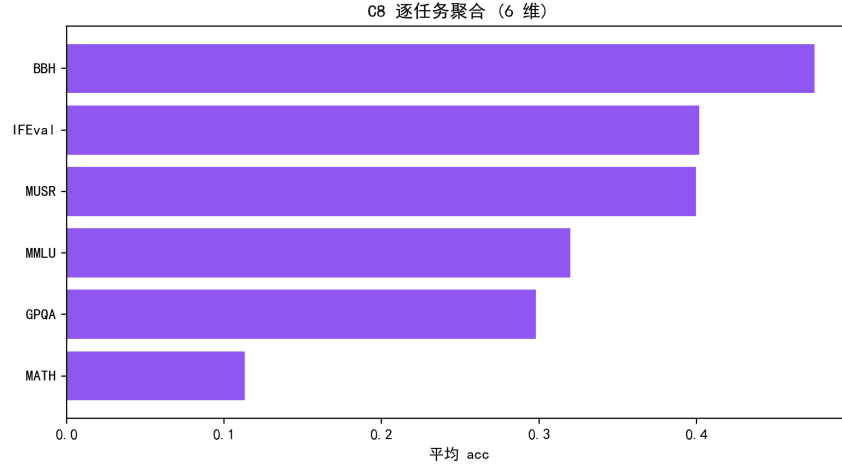
图 8.23 C8 逐任务聚合得分（6 维）。
