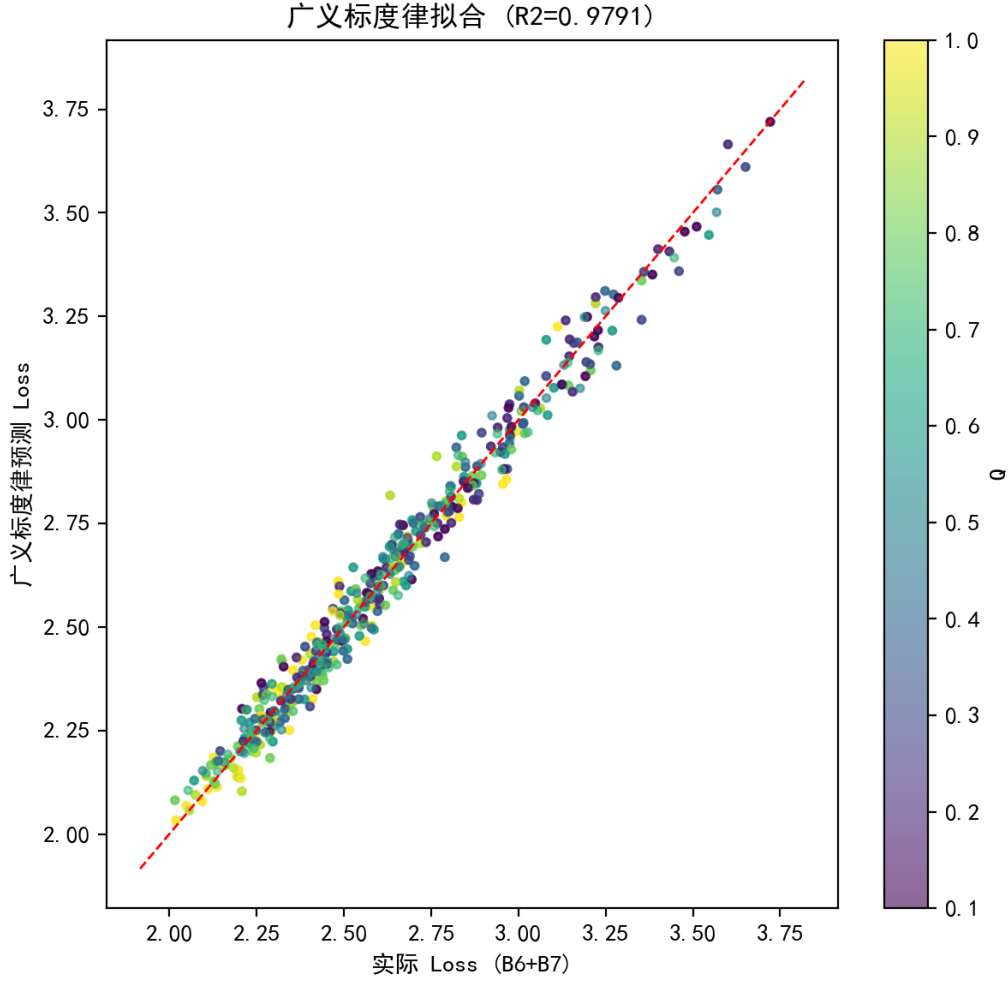
图 6.7 广义标度律在 B6+B7 数据上的拟合（质量-参数量交互形式， R^2 = 0.979 ）。
