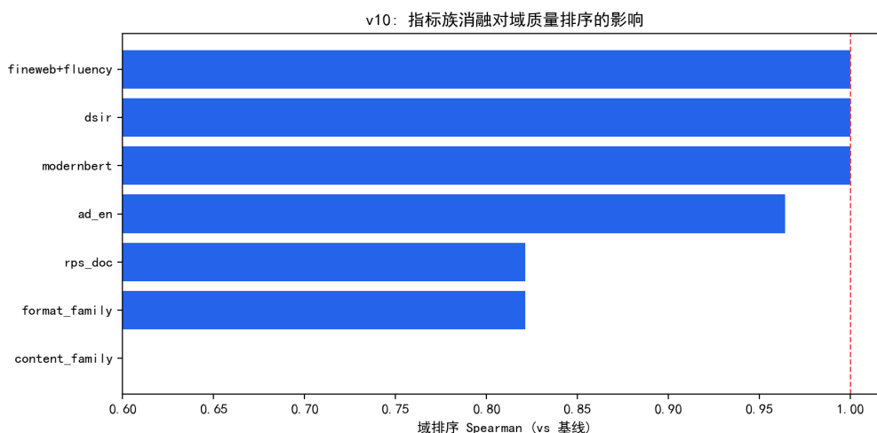
图 9.24 指标族消融对域质量排序的影响（红虚线为完全一致）。
