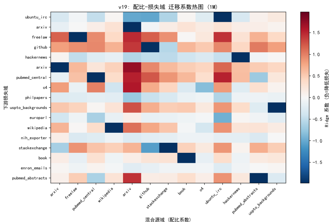
图 5.5 配比源域 × 损失域迁移系数热图 (1M 尺度，负值 = 压低损失)。
