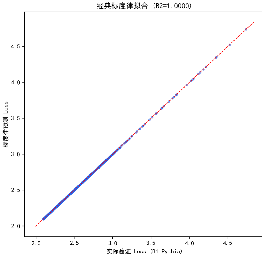
图 6.8 经典标度律在 B1 轨迹上的拟合与跨家族验证。
