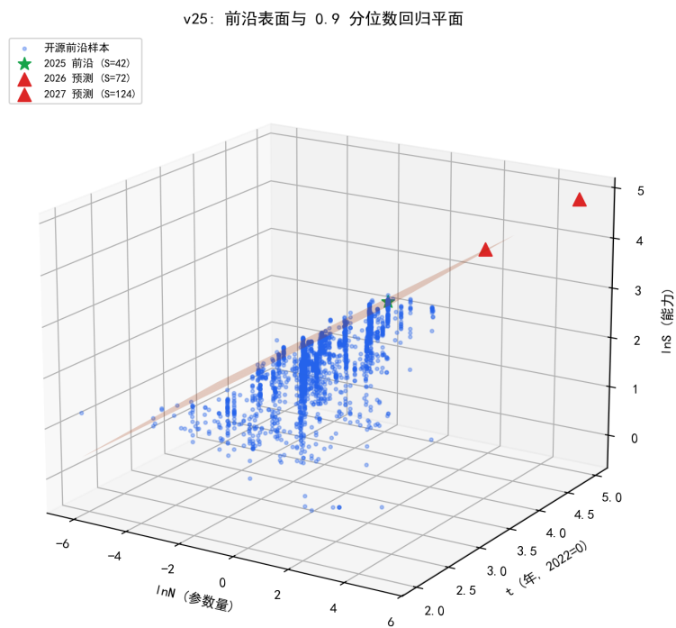
图 8.26 能力前沿 3D 表面与 0.9 分位数回归平面（星标 =2025 前沿，三角 = 预测点）。
