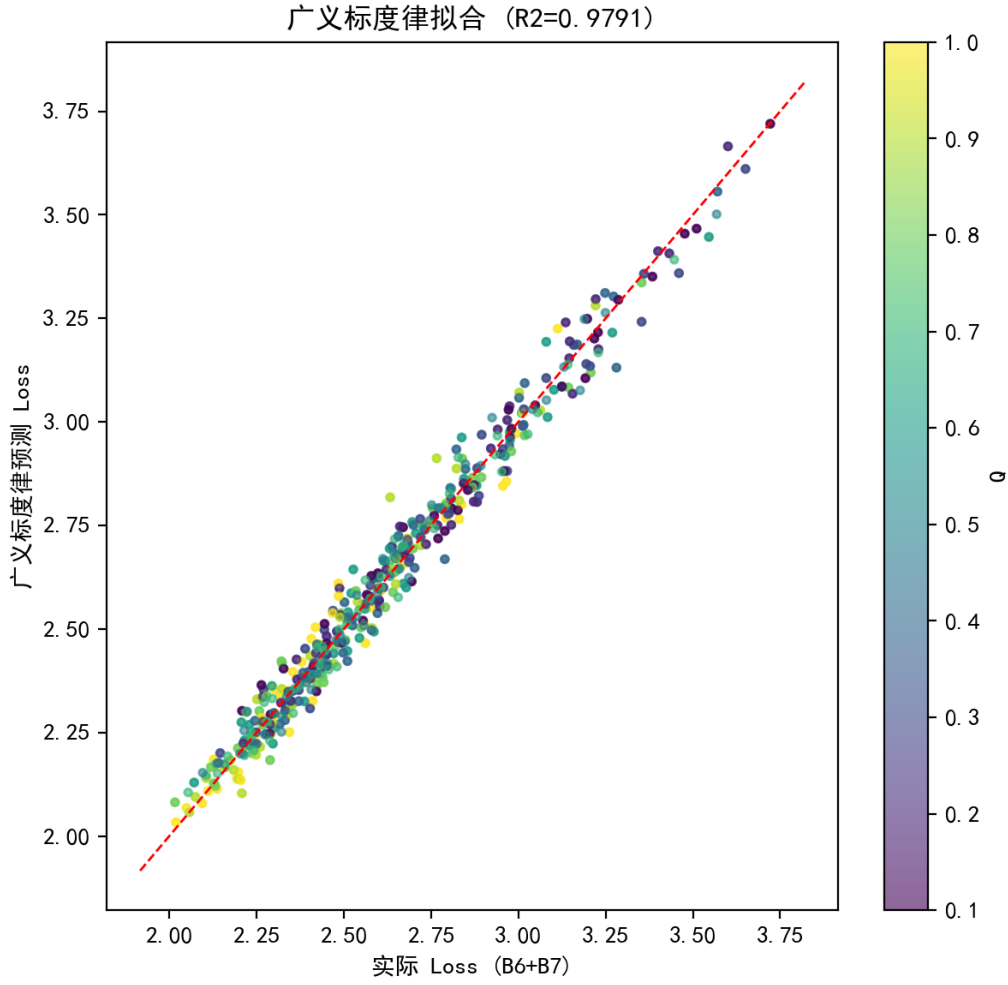
图 6.10 广义标度律在 B6+B7 数据上的拟合（质量-参数量交互形式， R^2 = 0.979 ）。
