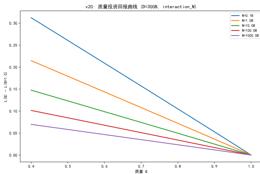
图 6.12 质量投资回报曲线（ D = 300B ）： L(Q) 相对 L(Q = 1) 随 N 变化。
