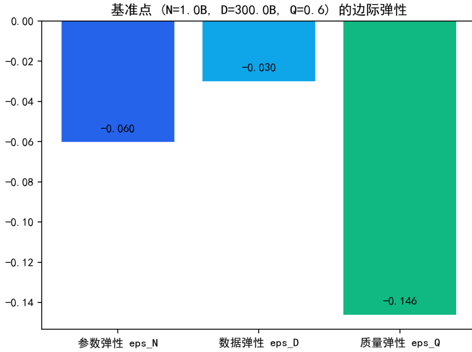
图 6.13 基准点处三个维度的损失弹性对比（质量弹性最高）。
