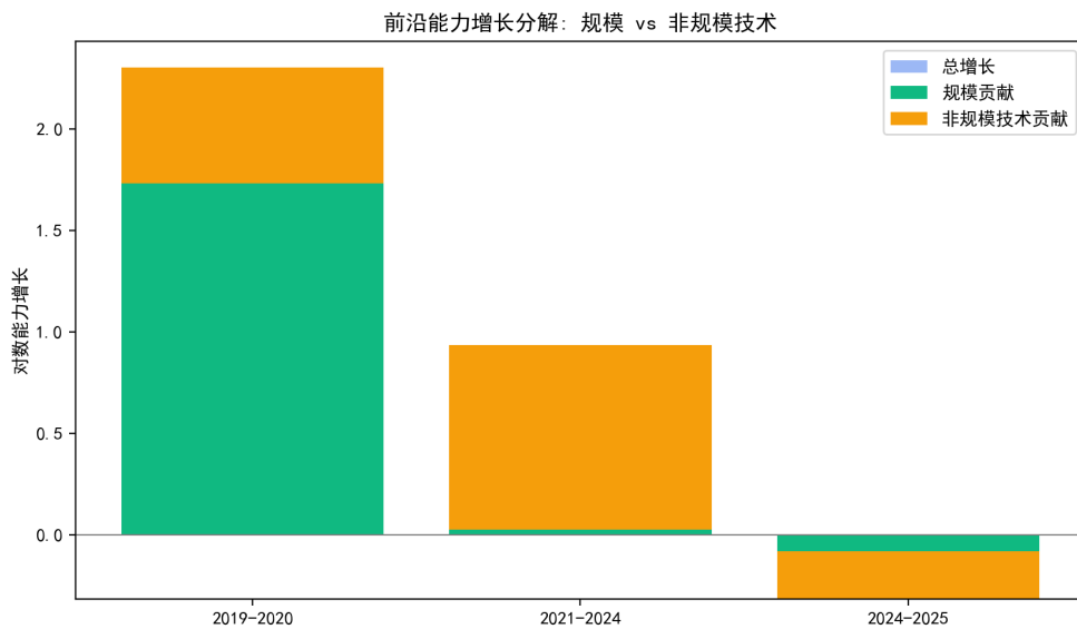
图 8.27 前沿能力增长分解：规模贡献与非规模技术贡献。
