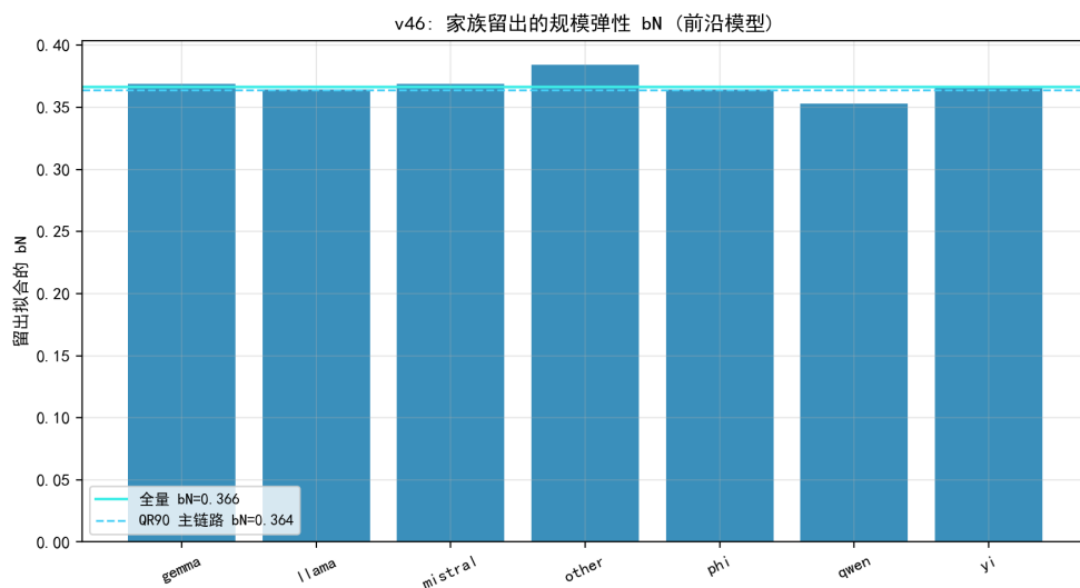
图 8.69 家族留下的规模弹性 b_N ：全家族稳定在 0.36 附近。
