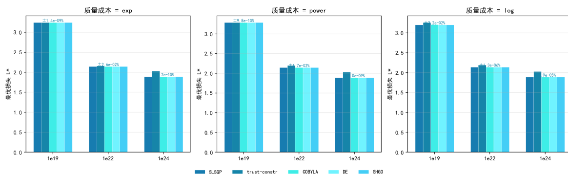
图 7.35 五框架求解对比：SLSQP/COBYLA/DE/SHGO 在 9 实例上一致到 10^{-6} 量级（括号为四框架最大相对偏差），trust-constr 内点法在边界角点最优处失稳。
