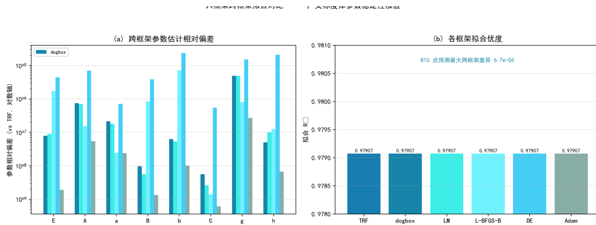
图 6.26 六框架跨框架拟合对比：参数最大相对极差 2.4 \times 10^{-3}\% ，预测差异 6.7 \times 10^{-6} ， R^2 全部为 0.979073。
