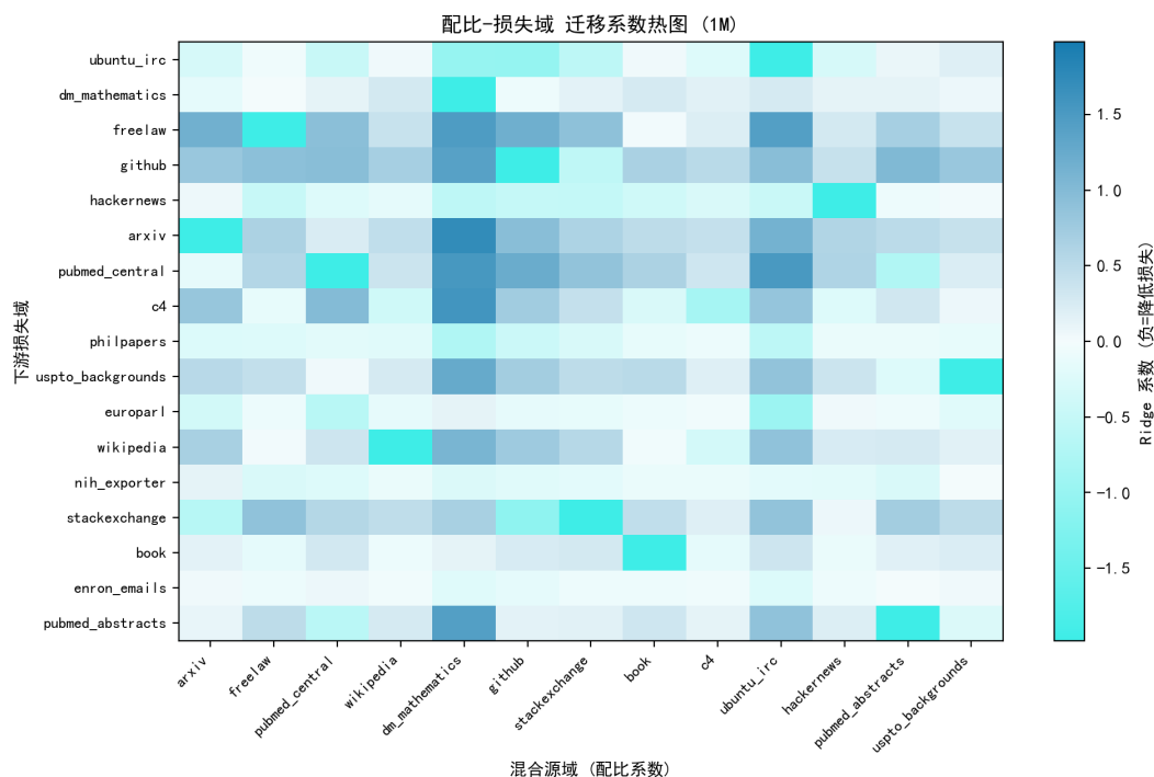
图 5.11 配比源域 \times 损失域迁移系数热图（1M 尺度，负值 = 压低损失）。
