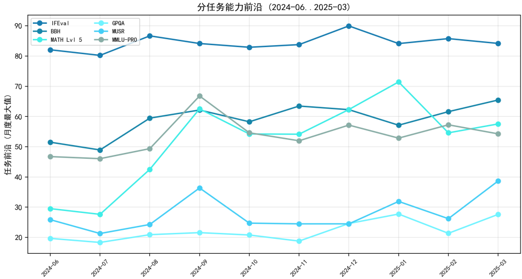
图 8.65 分任务能力前沿：推理类（MATH/GPQA/MUSR）增长快于知识/指令类。
