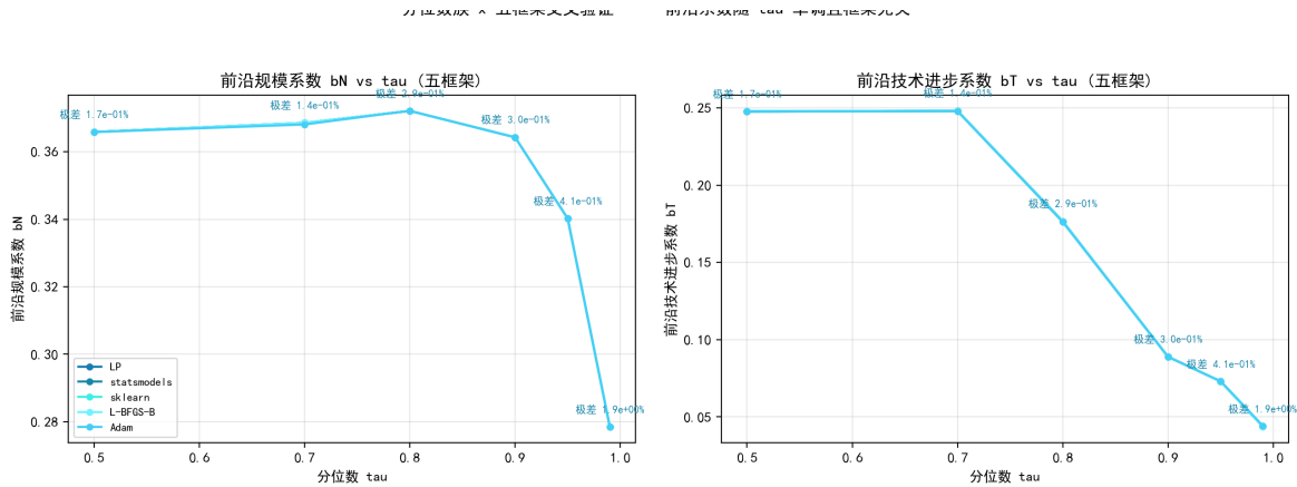
图 8.60 分位数族 \times 五框架: 每个 \tau 上五框架一致; b_T 随 \tau 单调递减、 b_N 峰后回落。
