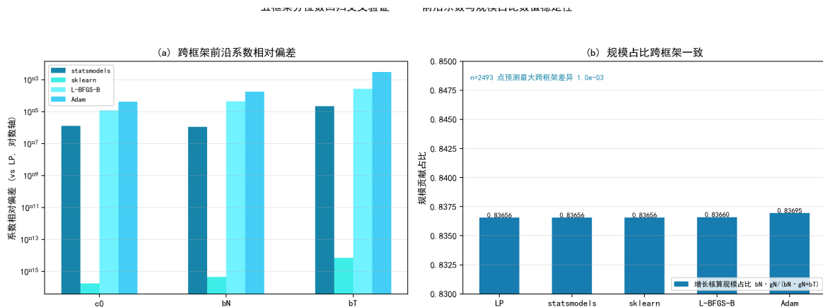
图 8.59 五框架分位数回归交叉验证：系数与规模贡献占比（83.7%）跨框架一致。
