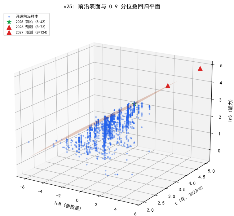
图 8.48 能力前沿 3D 表面与 0.9 分位数回归平面（星标 = 2025 前沿，三角 = 预测点）。
