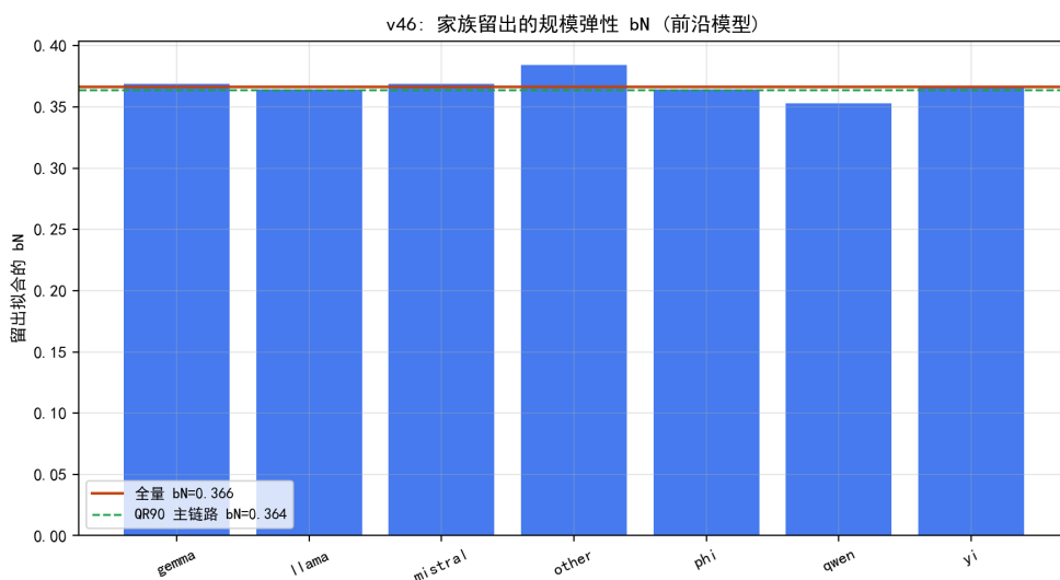
图 8.49 家族留出的规模弹性 b_N ：全家族稳定在 0.36 附近。
