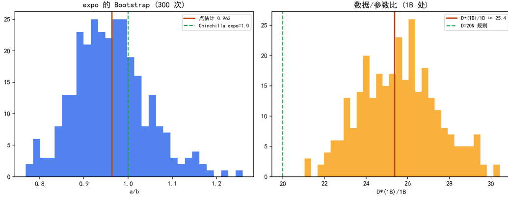
图 7.31 D^*(N) 参数 Bootstrap: 指数 CI 含 1.0, 常数 CI 高于 D = 20N 。
