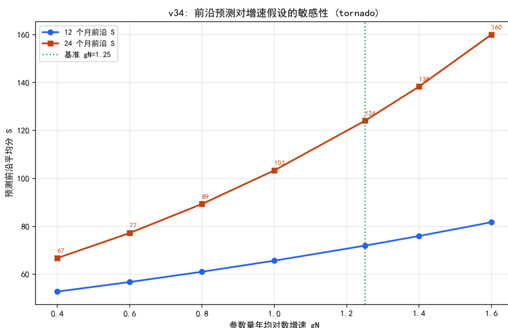
图 8.43 前沿预测对参数量增速假设 g_N 的敏感性（12/24 个月）。
