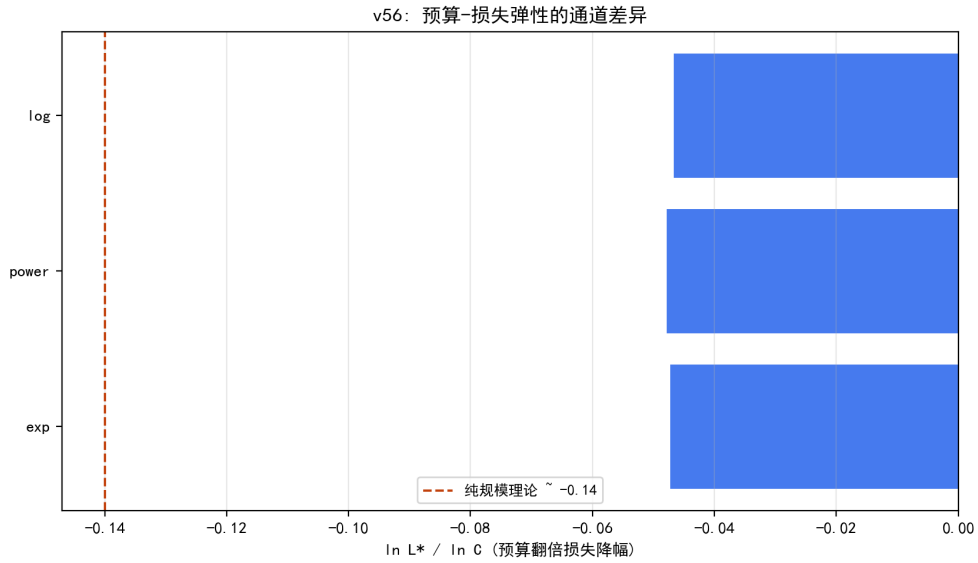
图 7.29 总损失口径的预算弹性：三形式几乎重合，低于超额口径斜率。
