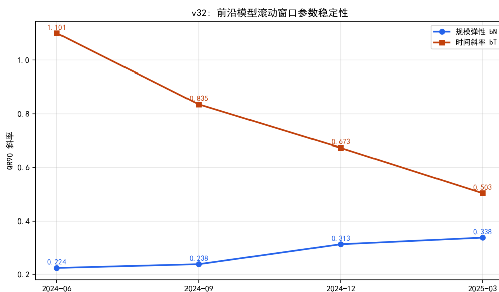
图 8.46 前沿 QR90 滚动窗口参数：规模弹性上升、时间斜率持续下降。
