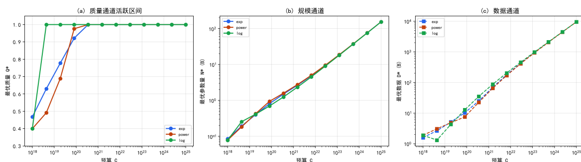
图 7.34 最优解族随预算轨迹：质量通道活跃区间由成本形式决定。
