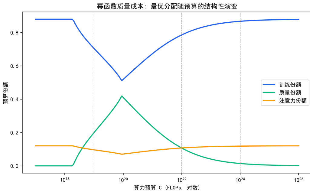
图 7.33 幂函数质量成本下最优成本份额随预算的结构性演变（竖线为三档预算）。
