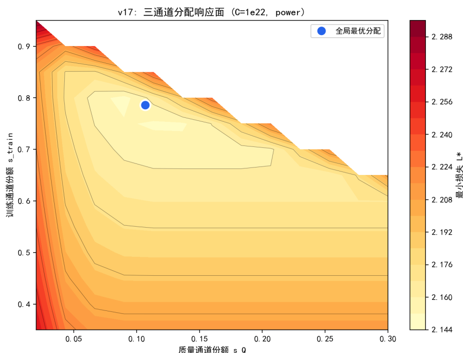
图 7.39 三通道分配响应面（ C = 10^{22} ，幂成本；蓝点为全局最优分配）。
