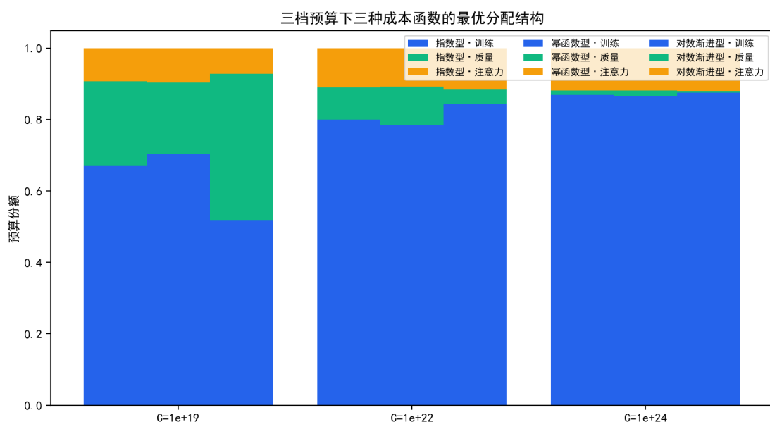
图 7.20 三档预算下三种质量成本函数的最优成本份额结构。
