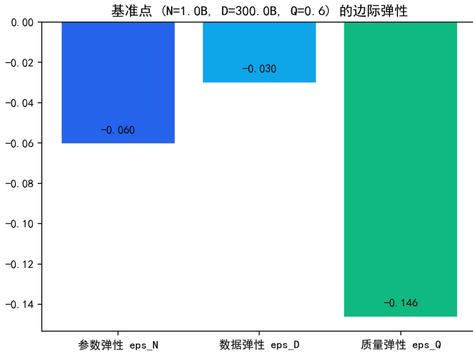
图 6.17 基准点处三个维度的损失弹性对比（质量弹性最高）。
