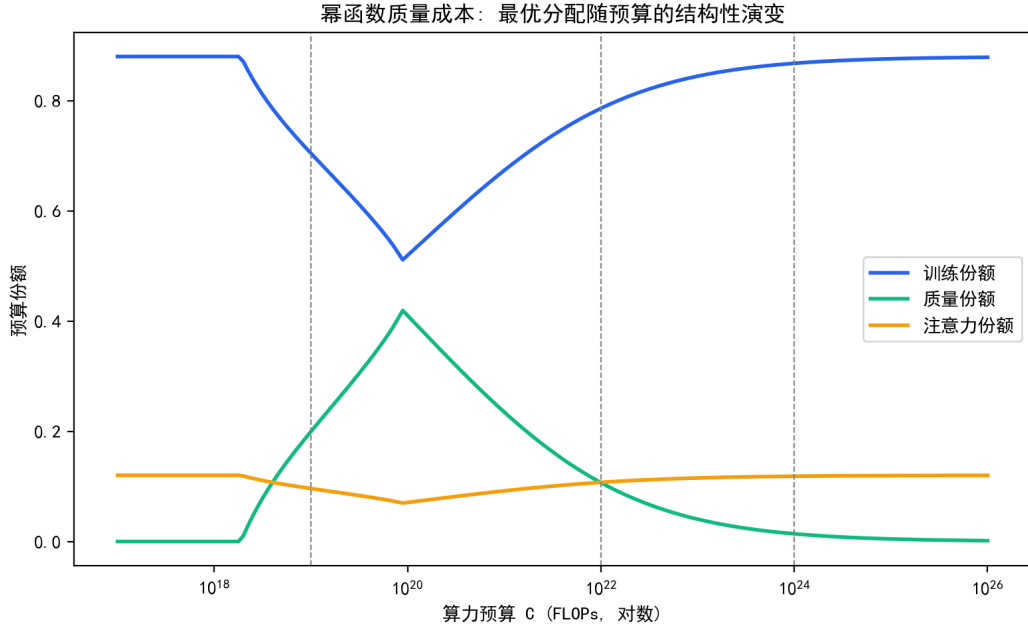
图 7.23 幂函数质量成本下最优成本份额随预算的结构性演变（竖线为三档预算）。
