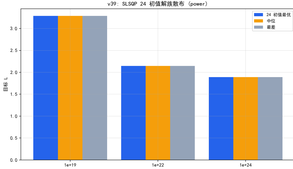
图 7.19 SLSQP 24 初值解族散布：三档预算全部初值收敛到同一最优。
