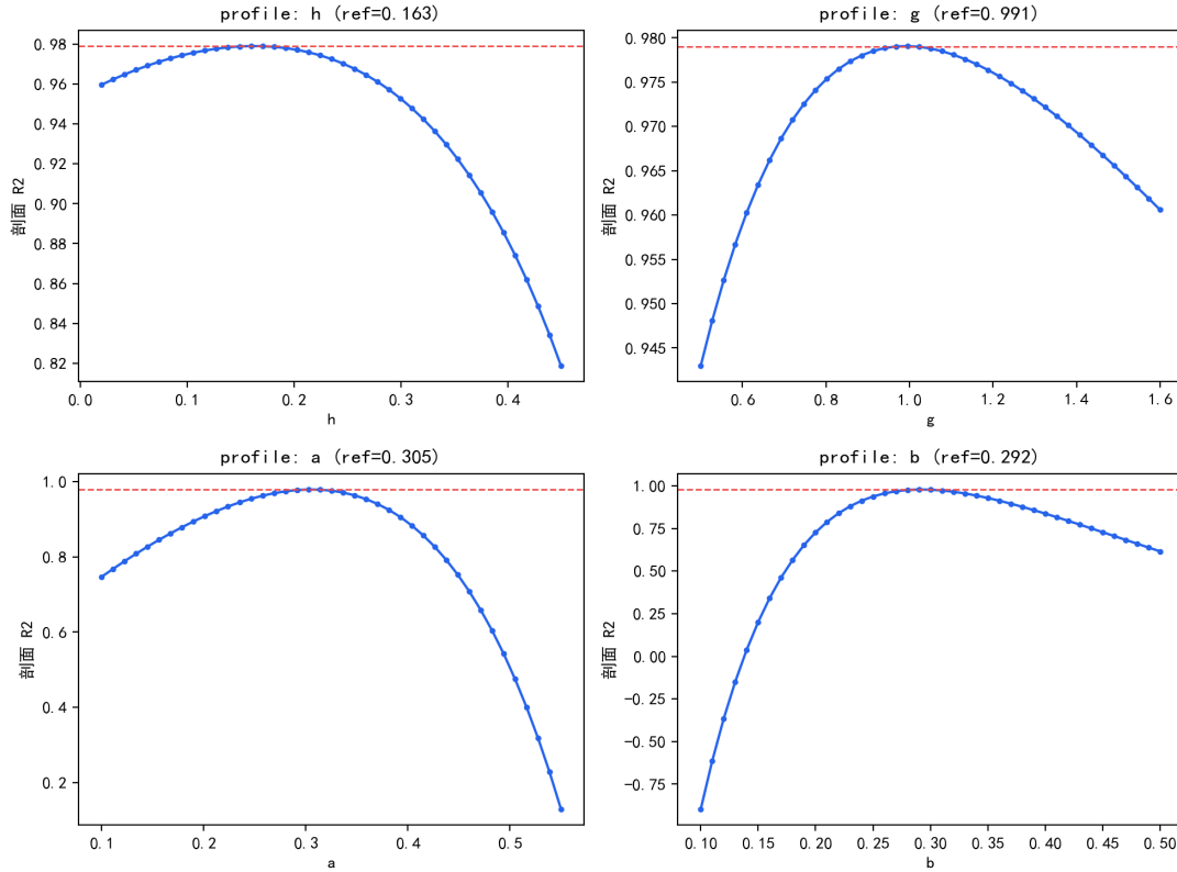
图 6.15 关键参数的剖面似然曲线（红色虚线为 90% 似然比阈值）。
