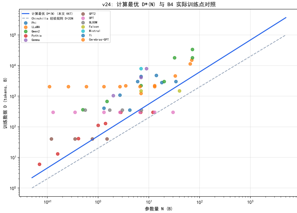
图 7.22 计算最优数据曲线 D^*(N) 、Chinchilla 经验规则与 B4 实际训练点。
