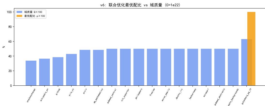
图 7.26 联合优化最优配比与域质量对比 ( C = 10^{22} )：配比向最高质量域（小说）集中。
