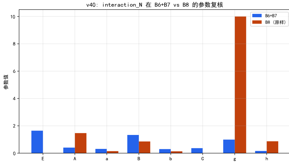
图 6.14 B8 原样 vs B6+B7 的参数对比：B8 质量项退化 ( E = C = 0 , g 撞界)。
