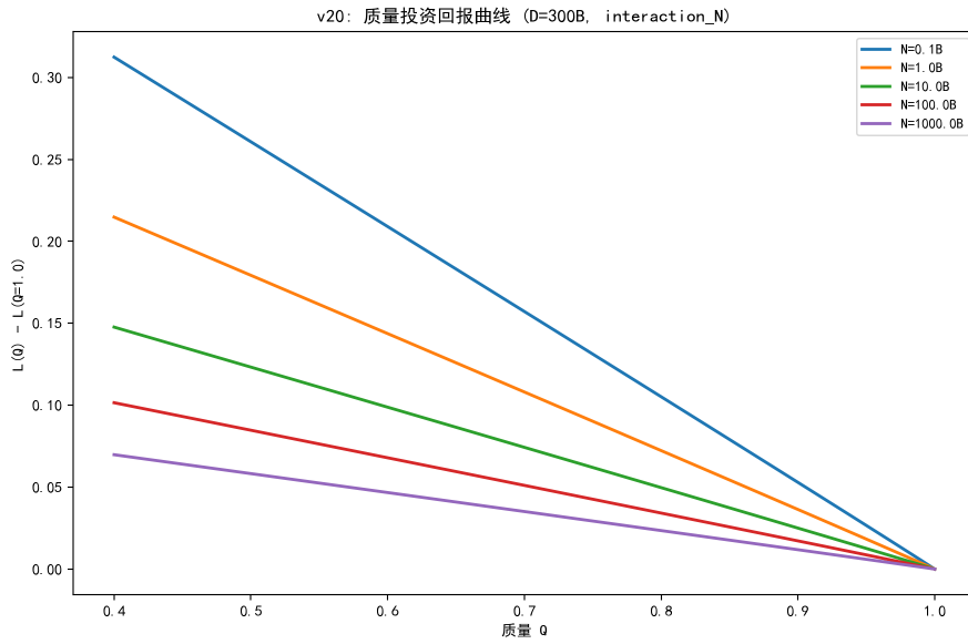
图 6.16 质量投资回报曲线 ( D = 300B ): L(Q) 相对 L(Q = 1) 随 N 变化。
