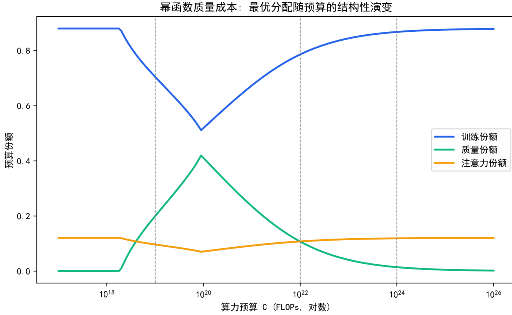
图 7.40 幂函数质量成本下最优成本份额随预算的结构性演变（竖线为三档预算）。
