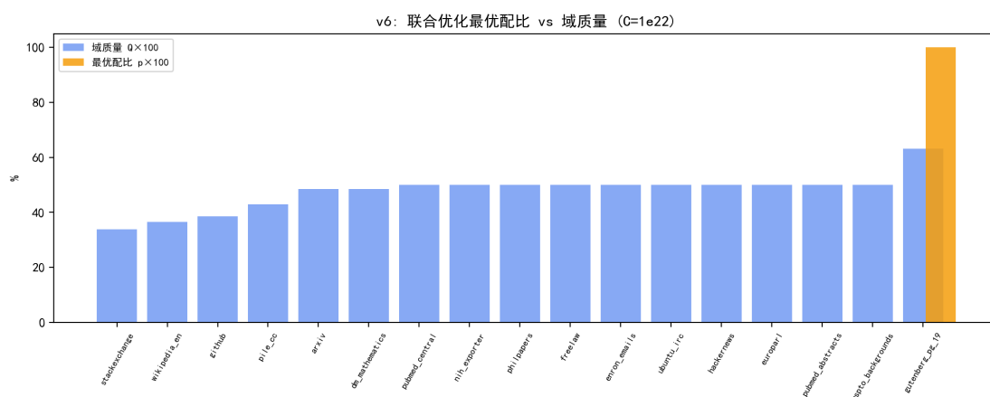
图 7.43 联合优化最优配比与域质量对比 ( C = 10^{22} )：配比向最高质量域（小说）集中。
