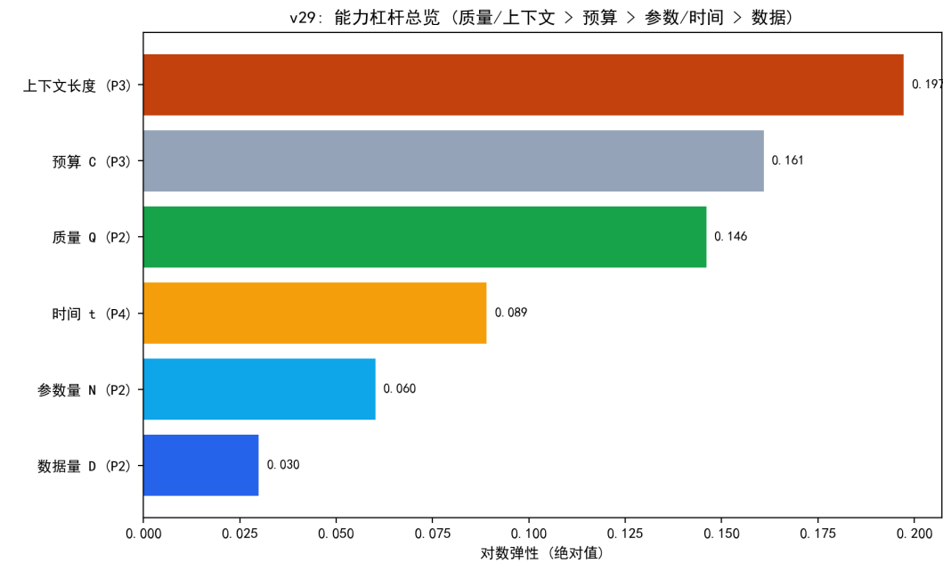
图 10.66 能力杠杆总览：各投入的对数弹性排序（质量/上下文 > 预算 > 参数/时间 > 数据）。
