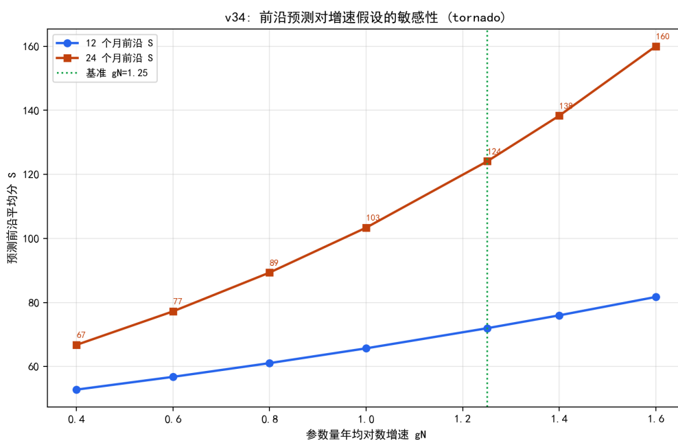
图 8.51 前沿预测对参数量增速假设 g_N 的敏感性（12/24 个月）。
