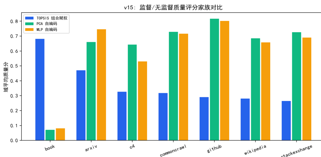
图 9.65 TOPSIS 组合赋权与自编码典型性评分的域级对照（方向相反）。
