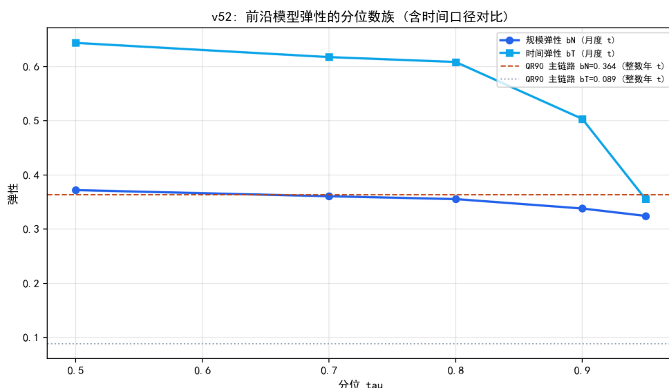
图 9.63 前沿弹性的分位数族与时间口径对比（ b_N 稳健， b_T 对口径敏感）。
