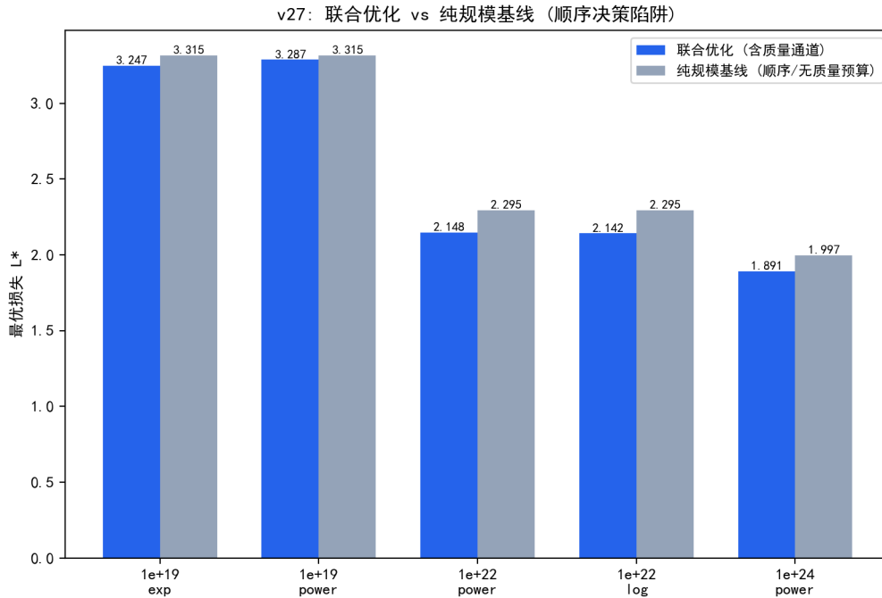
图 7.44 联合优化 vs 纯规模基线的最优损失（顺序决策陷阱：质量需预算预留）。
