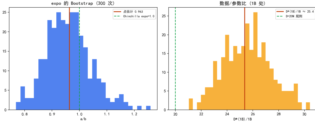
图 7.38 D^*(N) 参数 Bootstrap: 指数 CI 含 1.0, 常数 CI 高于 D = 20N 。
