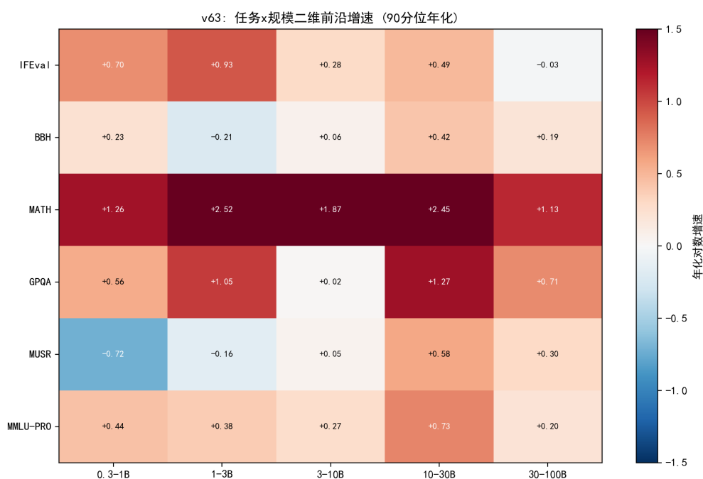
图 8.54 任务 × 规模二维前沿增速：MATH/GPQA 在 1–3B 与 10–30B 双峰。
