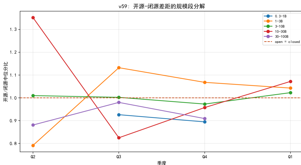
图 8.48 开源-闭源差距的规模段分解：中段持平、两端滞后约 10%。
