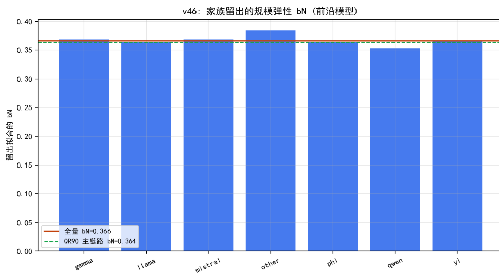
图 8.48 家族留下的规模弹性 b_N ：全家族稳定在 0.36 附近。
