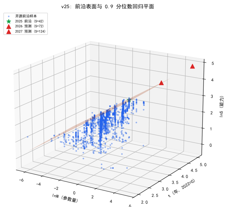
图 8.47 能力前沿 3D 表面与 0.9 分位数回归平面（星标 = 2025 前沿，三角 = 预测点）。
