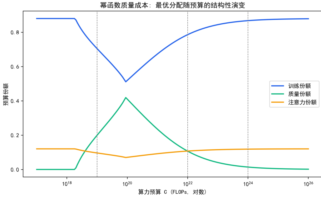
图 7.32 幂函数质量成本下最优成本份额随预算的结构性演变（竖线为三档预算）。
