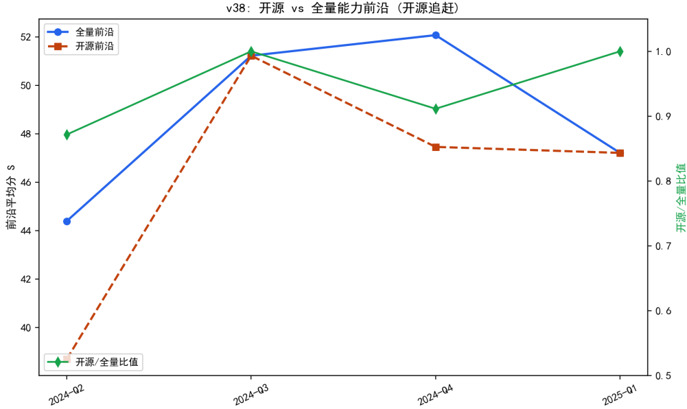
图 8.39 开源 vs 全量能力前沿：开源在 2024Q3/2025Q1 追平全量领跑。
