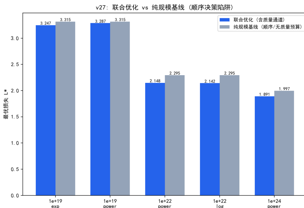
图 7.36 联合优化 vs 纯规模基线的最优损失 (顺序决策陷阱: 质量需预算预留)。
