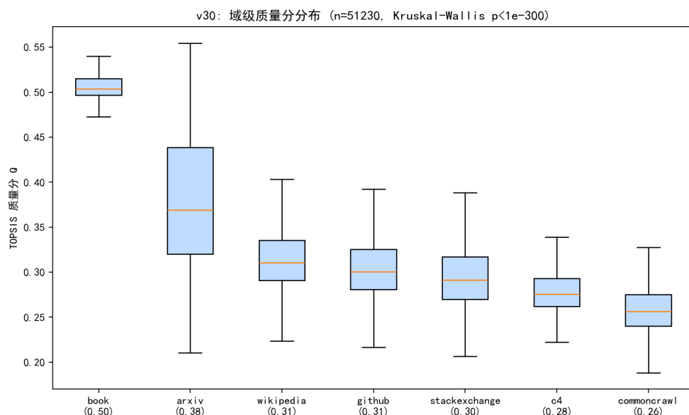
图 5.10 七域样本级质量分布（箱线图，Kruskal-Wallis p < 10^{-300} ）。
