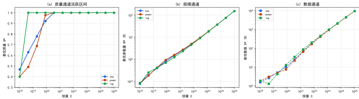
图 7.33 最优解族随预算轨迹：质量通道活跃区间由成本形式决定。
