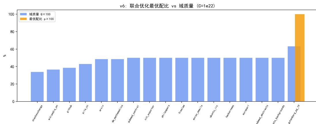
图 7.35 联合优化最优配比与域质量对比 ( C = 10^{22} ): 配比向最高质量域 (小说) 集中。
