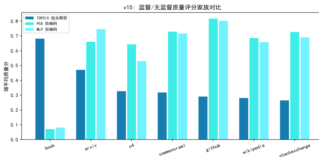
图 9.71 TOPSIS 组合赋权与自编码典型性评分的域级对照（方向相反）。
