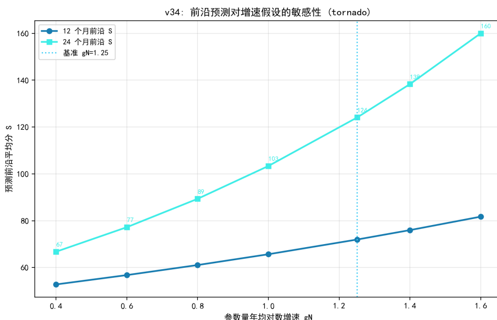
图 8.57 前沿预测对参数量增速假设 g_N 的敏感性（12/24 个月）。
