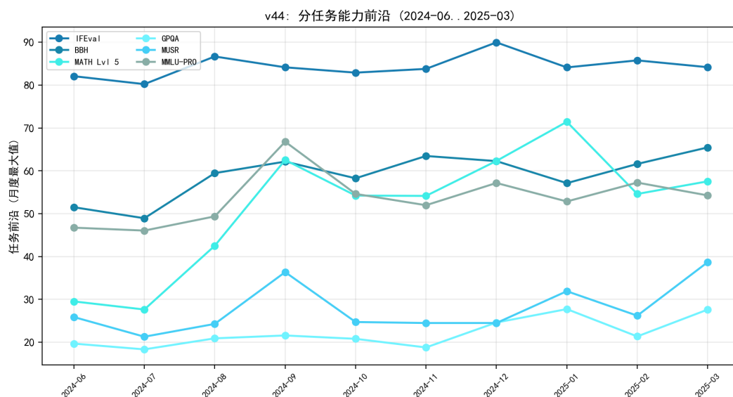
图 8.58 分任务能力前沿：推理类（MATH/GPQA/MUSR）增长快于知识/指令类。
