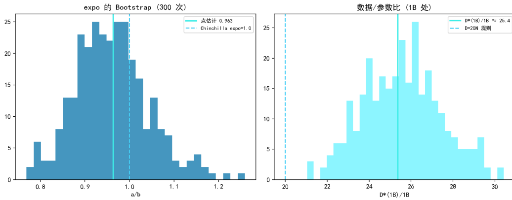
图 7.41 D^*(N) 参数 Bootstrap: 指数 CI 含 1.0, 常数 CI 高于 D = 20N 。
