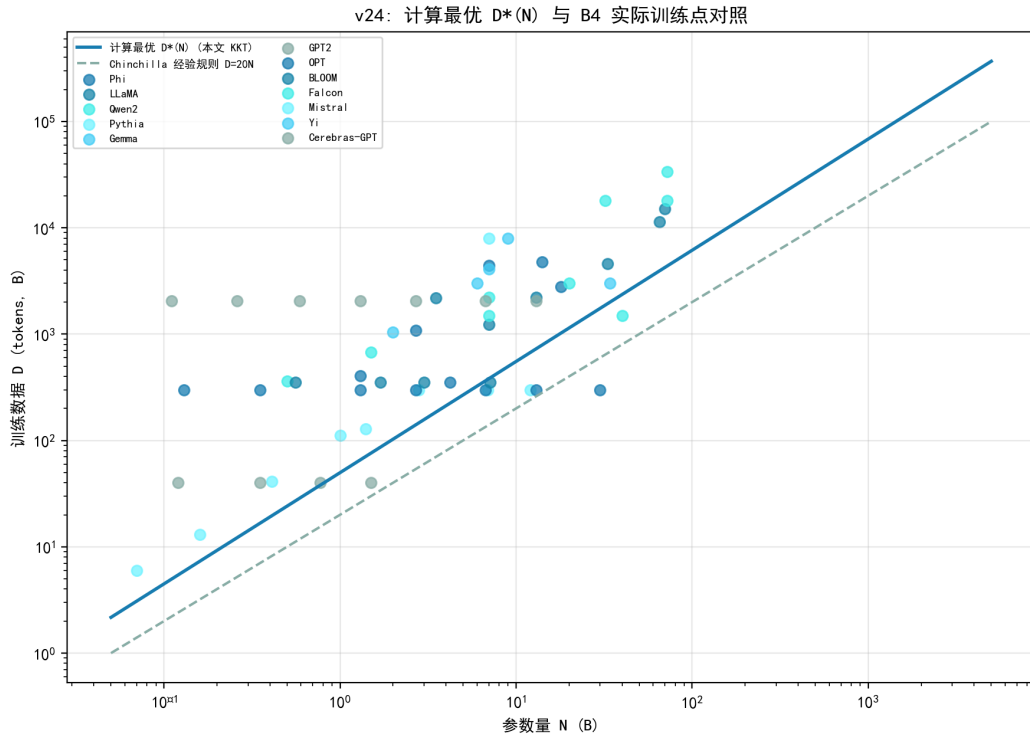
图 7.40 计算最优数据曲线 D^*(N) 、Chinchilla 经验规则与 B4 实际训练点。
