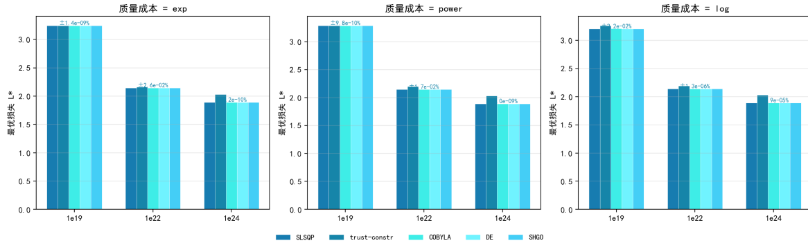
图 7.34 五框架求解对比：SLSQP/COBYLA/DE/SHGO 在 9 实例上一致到 10^{-6} 量级（括号为四框架最大相对偏差），trust-constr 内点法在边界角点最优处失稳。
