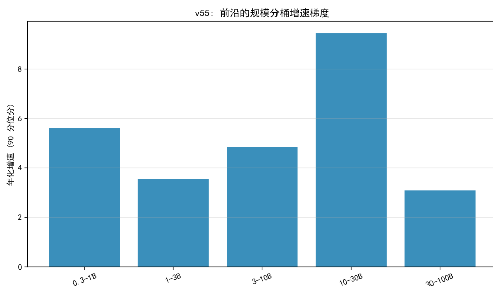
图 8.59 规模分桶的前沿年化增速：10-30B 甜点区最快，30-100B 最慢。
