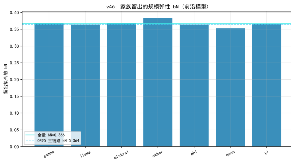
图 8.65 家族留出的规模弹性 b_N ：全家族稳定在 0.36 附近。
