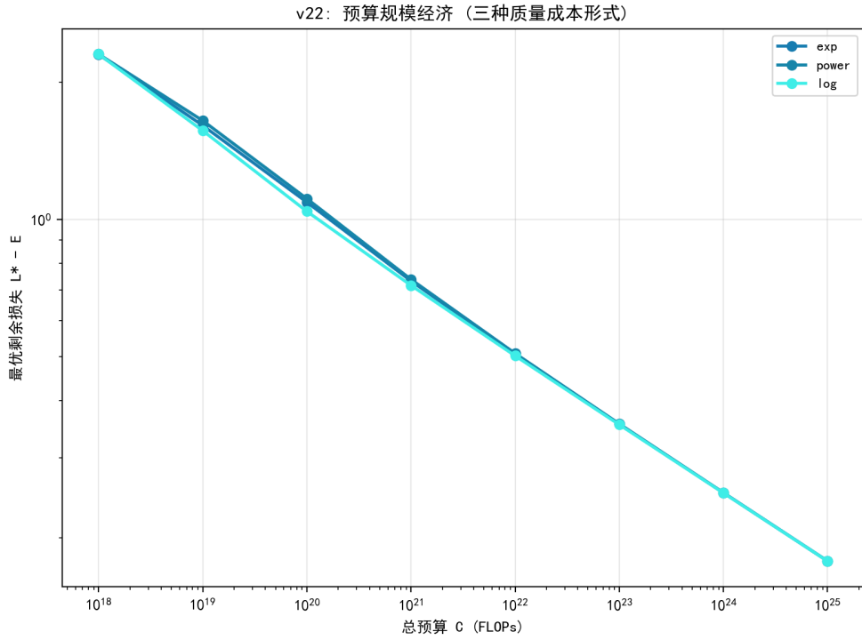
图 7.36 预算-最优损失的对数线性规律（三种质量成本形式）。
