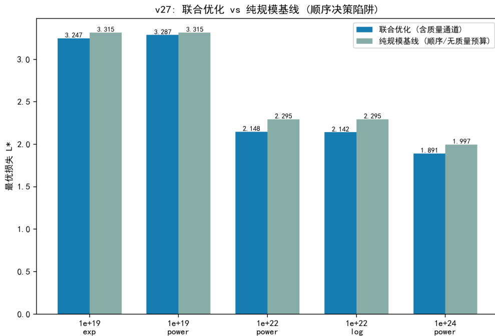
图 7.47 联合优化 vs 纯规模基线的最优损失 (顺序决策陷阱: 质量需预算预留)。
