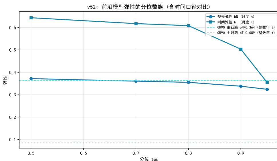
图 9.69 前沿弹性的分位数族与时间口径对比（bN 稳健，bT 对口径敏感）。
