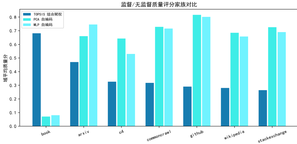
图 9.78 TOPSIS 组合赋权与自编码典型性评分的域级对照（方向相反）。
