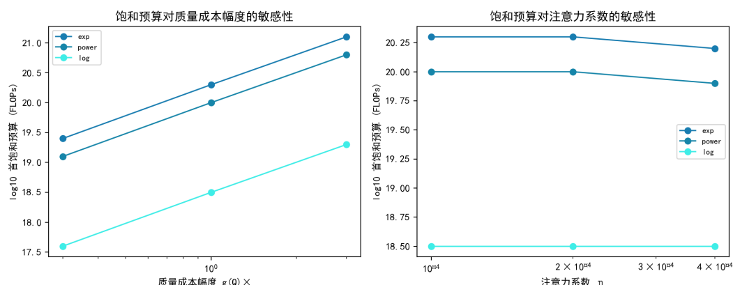
图 9.79 首饱和和预算对质量成本幅度（左）与注意力系数（右）的敏感性。
