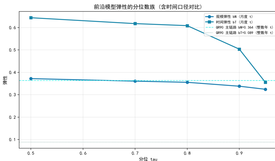
图 9.80 前沿弹性的分位数族与时间口径对比（bN 稳健，bT 对口径敏感）。
