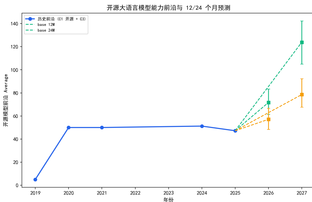
图 8.50 开源模型能力前沿（历史点）与 12/24 个月预测（基础/放缓情景，90% 区间）。
