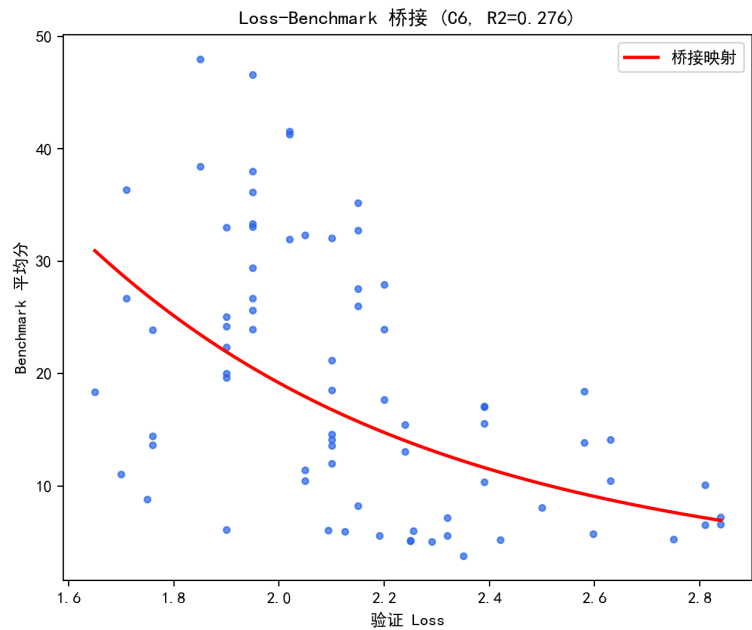
图 8.20 Loss-Benchmark 桥接映射（C6，75 个模型）。
