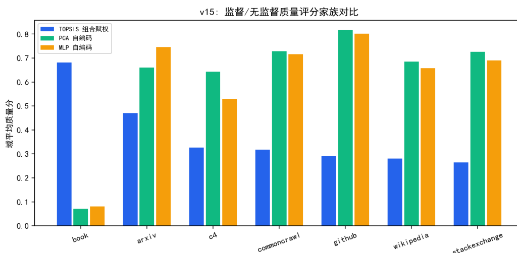
图 9.23 Topsis 组合赋权与自编码典型性评分的域级对照（方向相反）。
