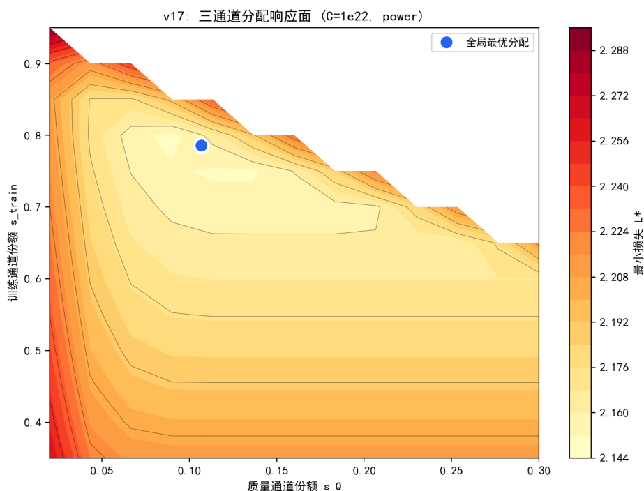
图 7.17 三通道分配响应面（ C = 10^{22} ，幂成本；蓝点为全局最优分配）。
