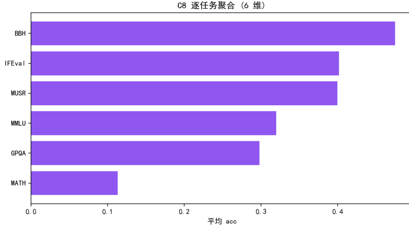
图 8.21 C8 逐任务聚合得分 (6 维)。
