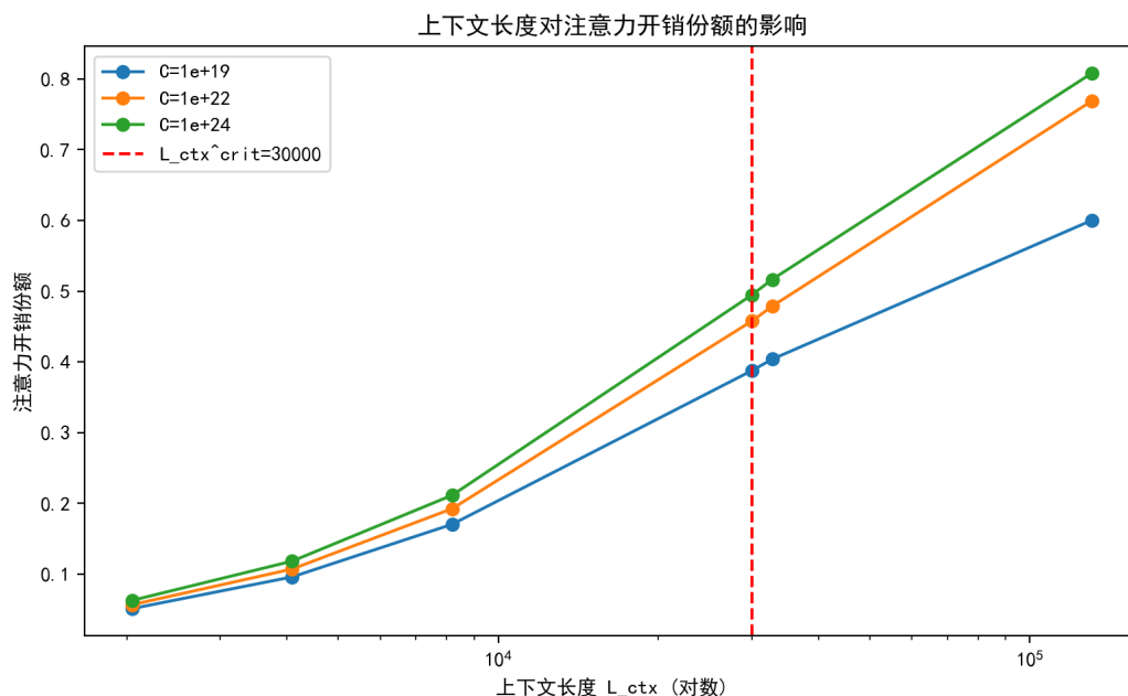
图 7.14 注意力开销份额随上下文长度的变化（红色虚线为临界点 30000）。
