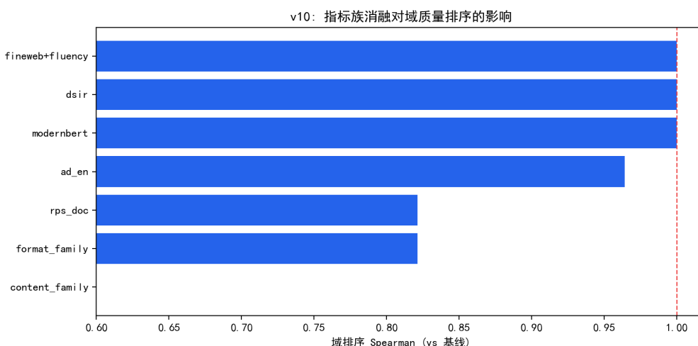
图 9.22 指标族消融对域质量排序的影响（红虚线为完全一致）。
