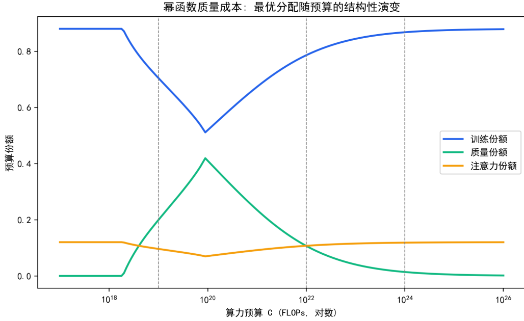
图 7.13 幂函数质量成本下最优成本份额随预算的结构性演变（竖线为三档预算）。
