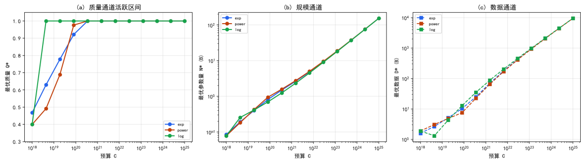
图 7.32 最优解族随预算轨迹：质量通道活跃区间由成本形式决定。
