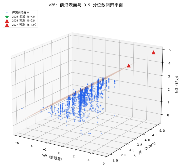
图 8.44 能力前沿 3D 表面与 0.9 分位数回归平面（星标 = 2025 前沿，三角 = 预测点）。
