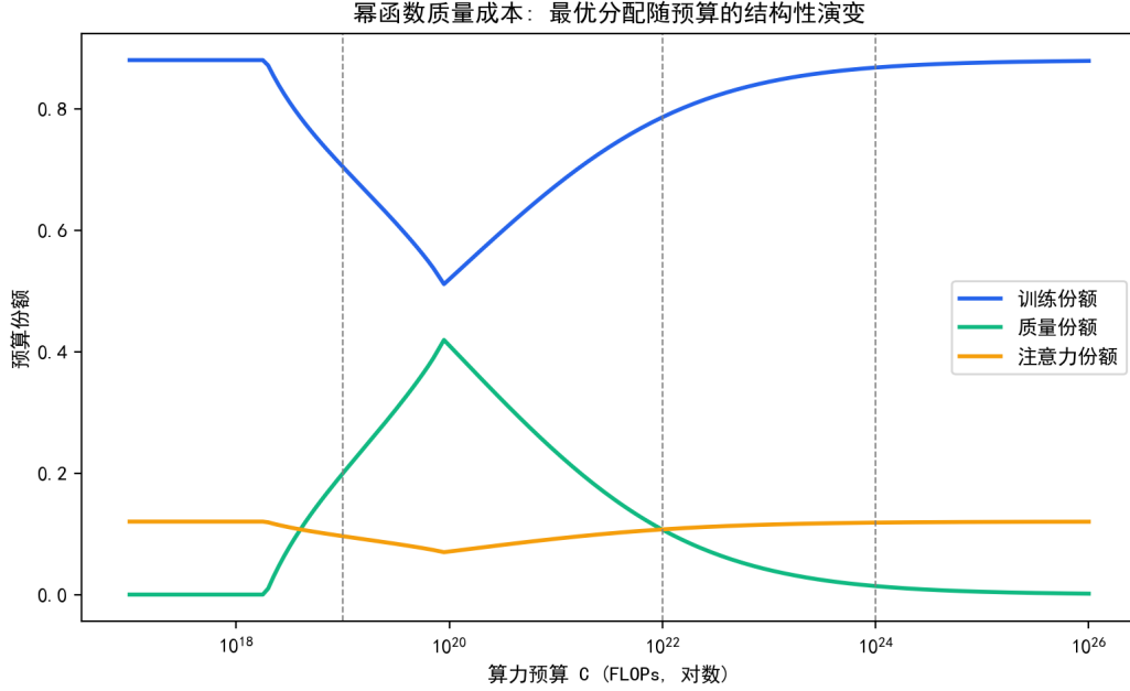
图 7.31 幂函数质量成本下最优成本份额随预算的结构性演变（竖线为三档预算）。
