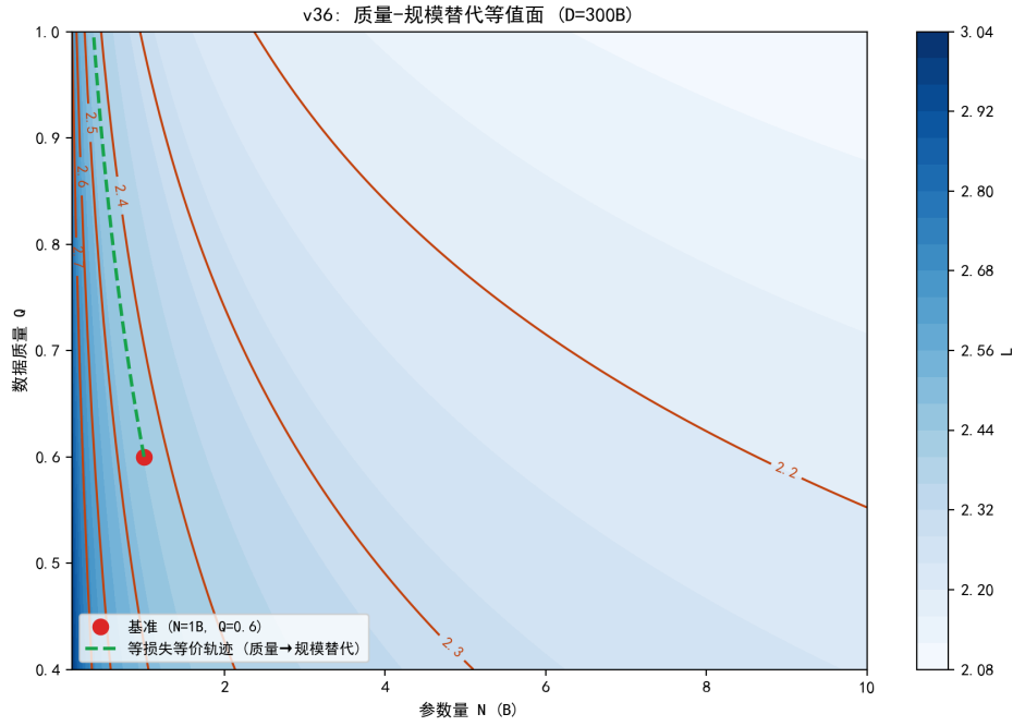
图 6.23 质量-规模替代等值面：等损失轨迹显示质量对参数的替代关系。
