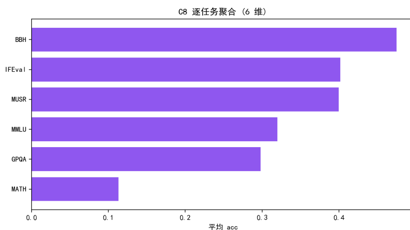
图 8.48 C8 逐任务聚合得分 (6 维)。
