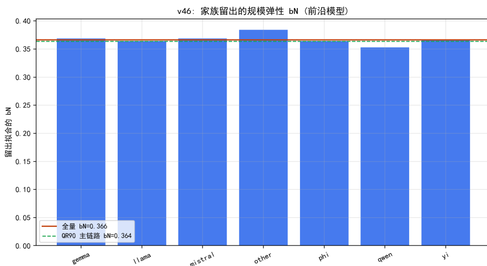
图 8.45 家族留出的规模弹性 b_N ：全家族稳定在 0.36 附近。
