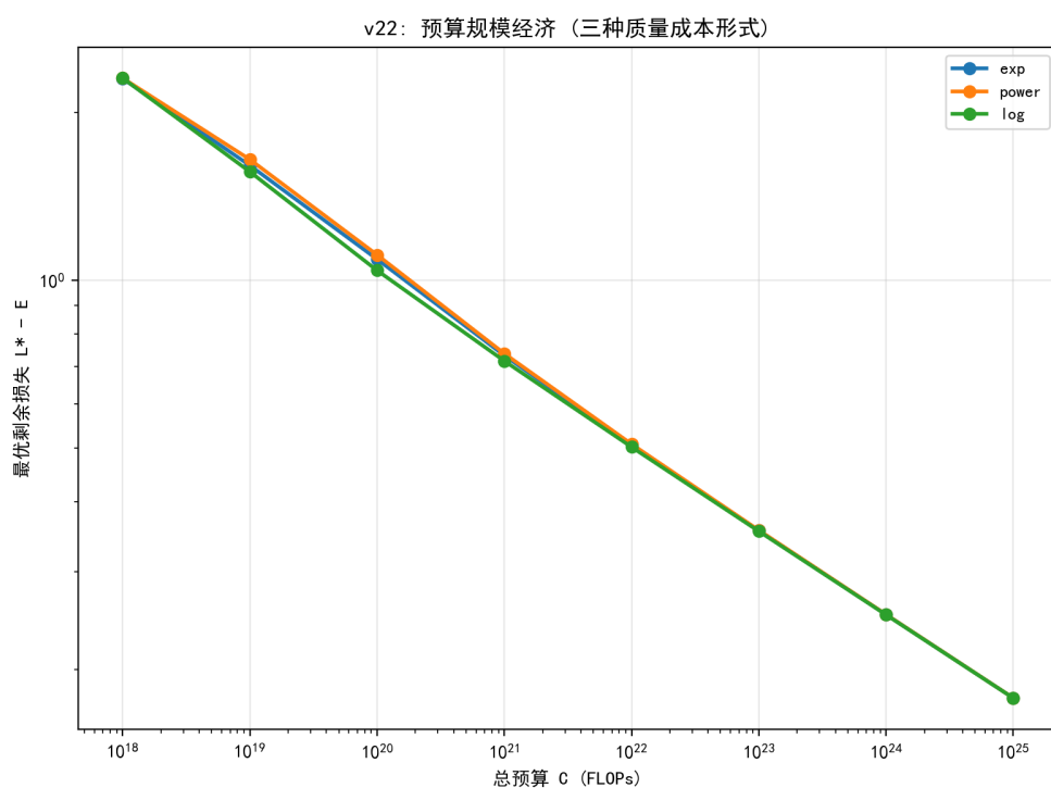
图 7.28 预算-最优损失的对数线性规律（三种质量成本形式）。
