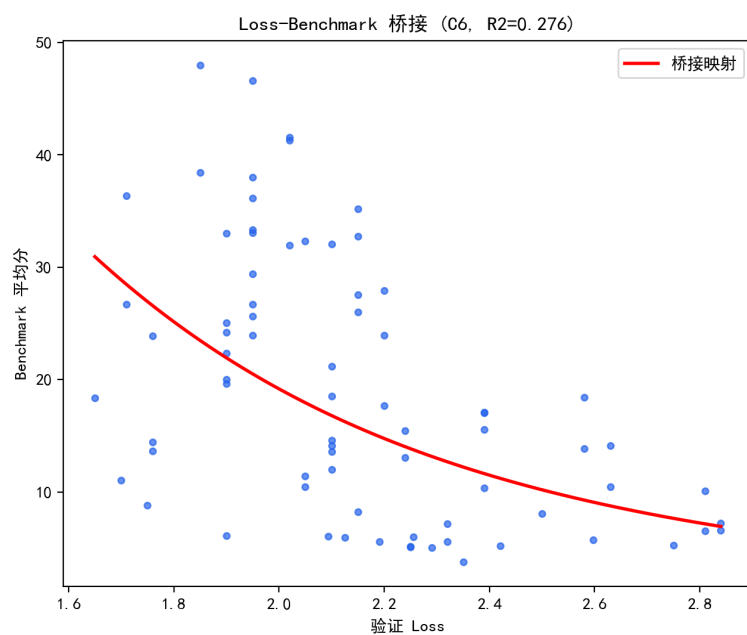
图 8.47 Loss-Benchmark 桥接映射 (C6, 75 个模型)。
