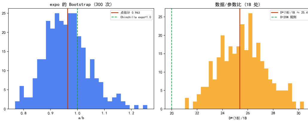
图 7.30 D^*(N) 参数 Bootstrap: 指数 CI 含 1.0, 常数 CI 高于 D = 20N 。
