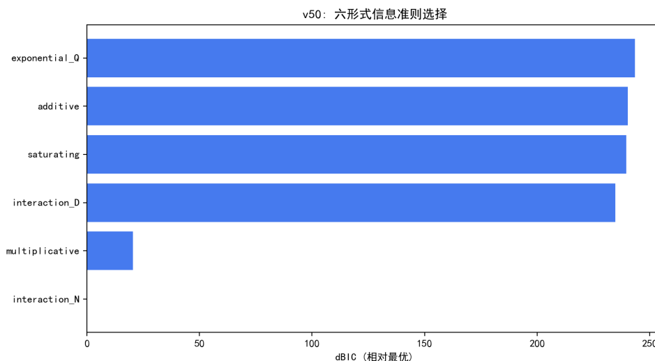
图 6.16 六种形式的 BIC/AIC 选择：interaction_N 决定性胜出。
