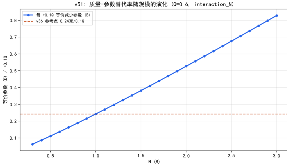
图 6.24 每 +0.1Q 等价减少的参数随规模的演化（近线性上升）。
