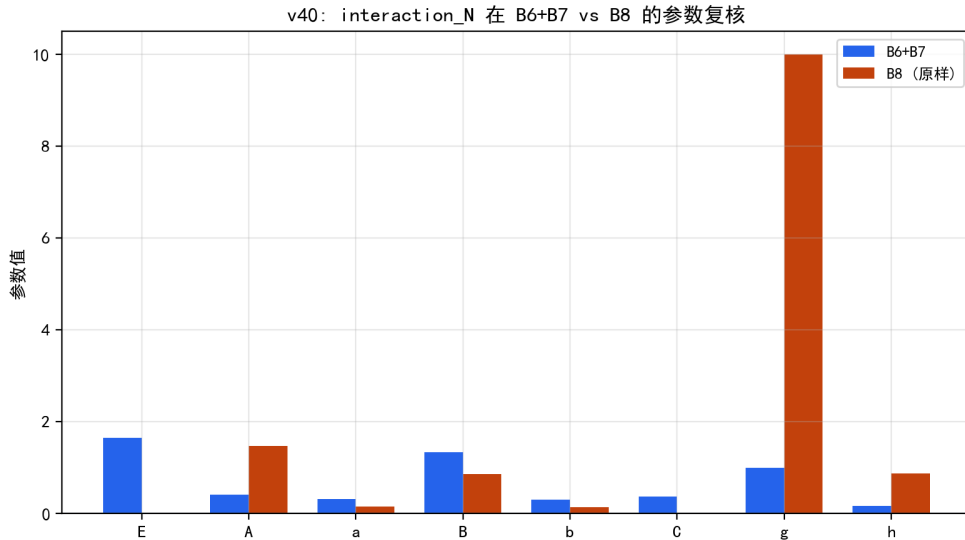
图 6.19 B8 原样 vs B6+B7 的参数对比：B8 质量项退化（ E = C = 0 ， g 撞界）。
