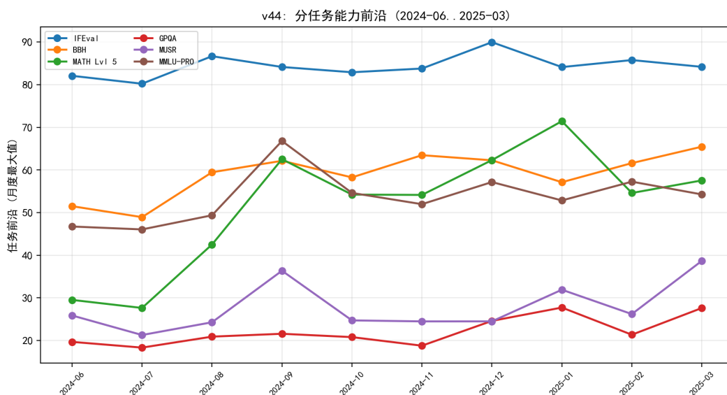
图 8.41 分任务能力前沿：推理类（MATH/GPQA/MUSR）增长快于知识/指令类。
