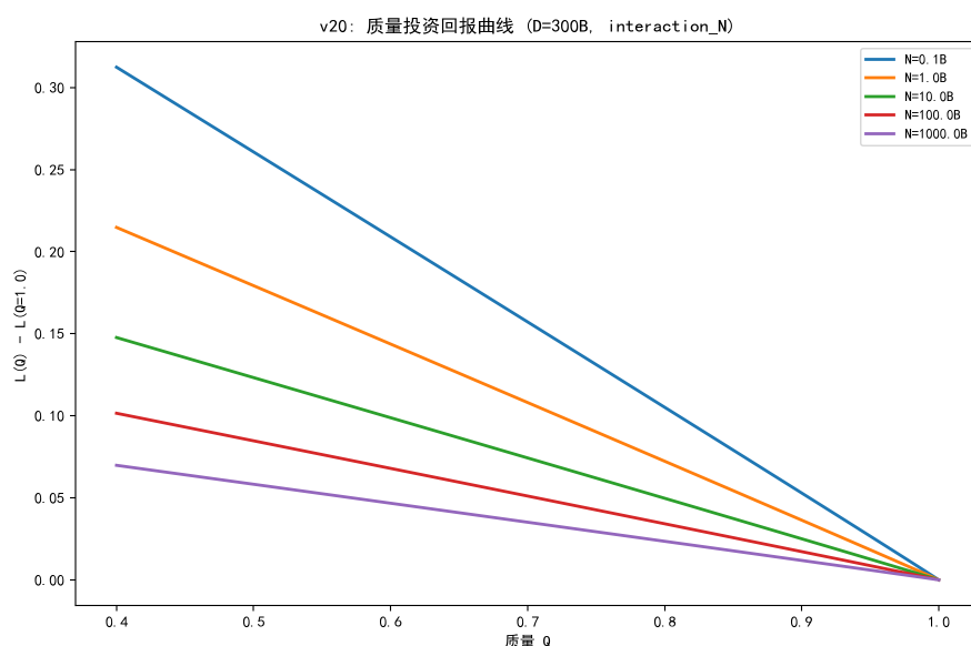
图 6.21 质量投资回报曲线（ D = 300B ）： L(Q) 相对 L(Q = 1) 随 N 变化。
