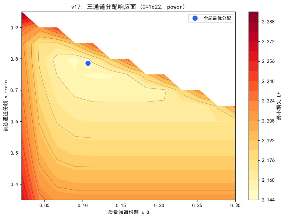
图 7.37 三通道分配响应面（ C = 10^{22} ，幂成本；蓝点为全局最优分配）。
