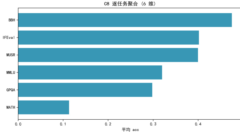
图 8.67 C8 逐任务聚合得分 (6 维)。
