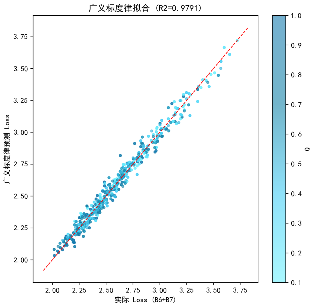
图 6.24 广义标度律在 B6+B7 数据上的拟合（质量-参数数量交互形式， R^2 = 0.979 ）。
