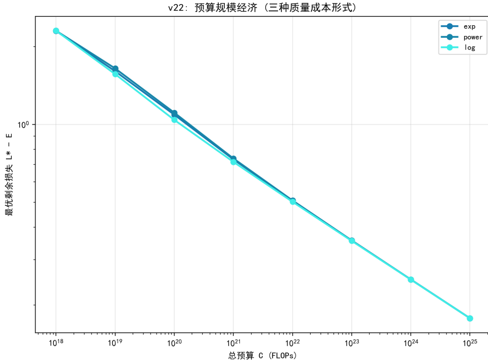
图 7.35 预算-最优损失的对数线性规律（三种质量成本形式）。
