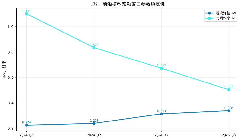
图 8.61 前沿 QR90 滚动窗口参数：规模弹性上升、时间斜率持续下降。
