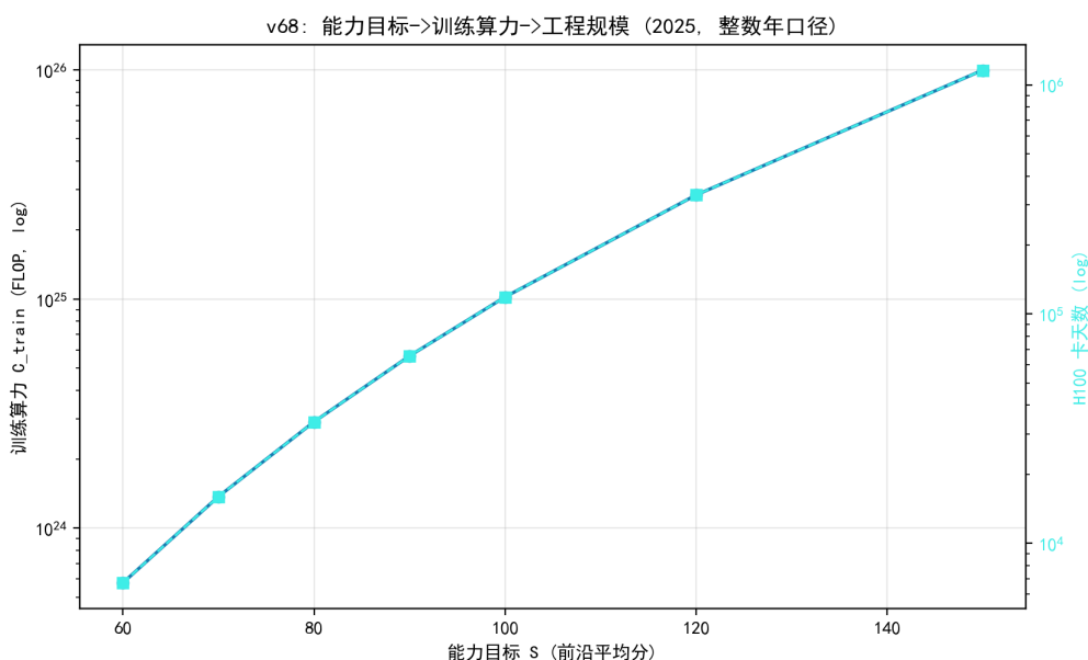
图 8.54 能力目标 → 训练算力 (对数轴)：S=90 约需 6.6 万卡天。
