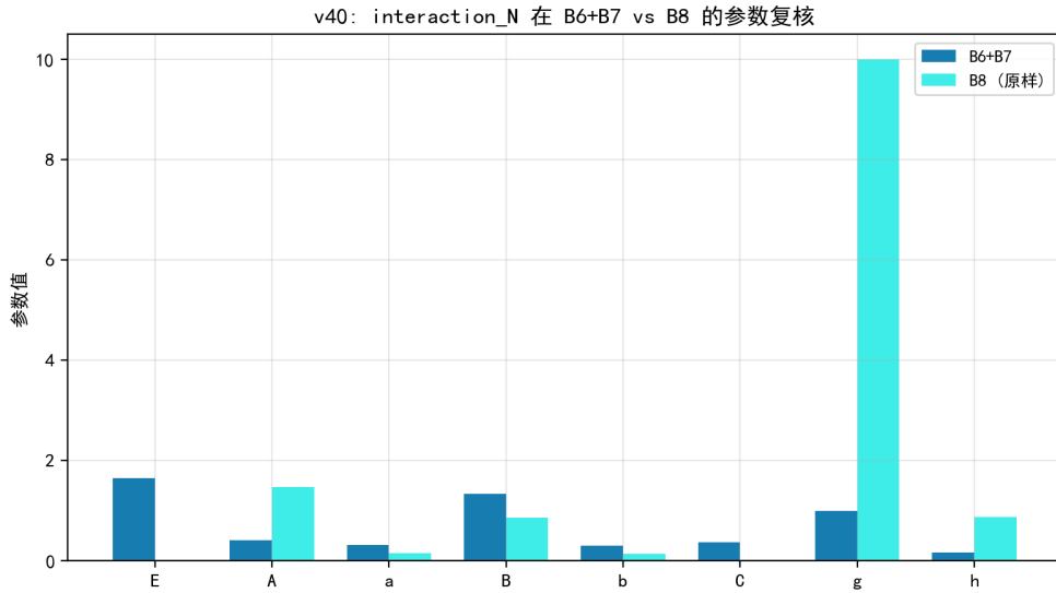
图 6.26 B8 原样 vs B6+B7 的参数对比：B8 质量项退化（ E = C = 0 ， g 撞界）。
