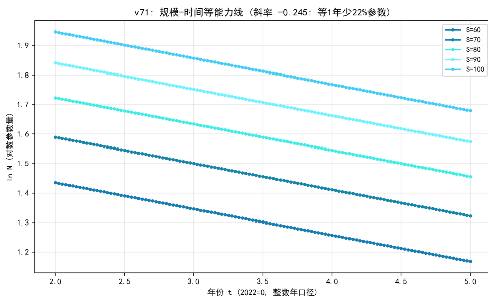
图 8.55 规模-时间等能力线：等 1 年少用 22% 参数（斜率 -0.245）。
