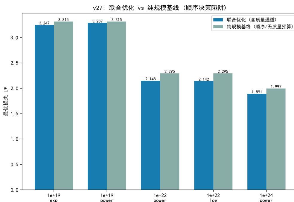
图 7.46 联合优化 vs 纯规模基线的最优损失（顺序决策陷阱：质量需预算预留）。
