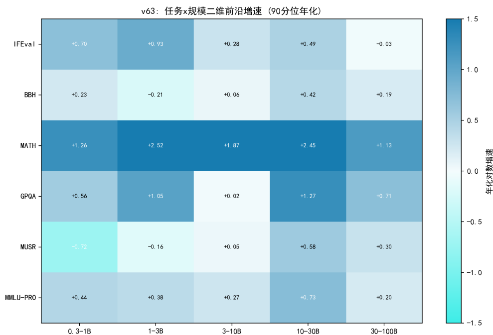
图 8.59 任务 × 规模二维前沿增速：MATH/GPQA 在 1–3B 与 10–30B 双峰。
