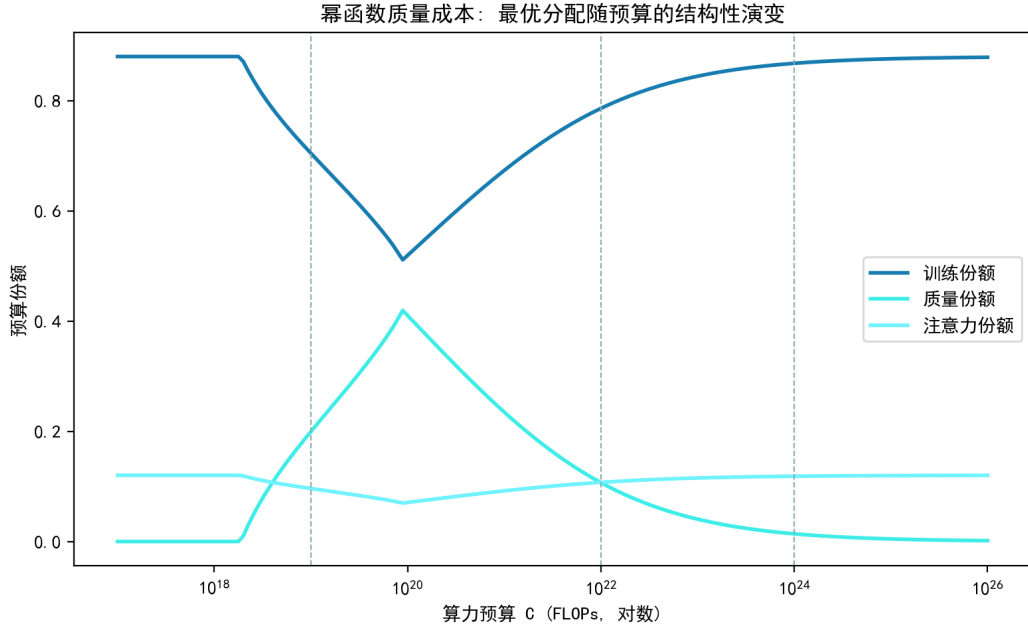
图 7.42 幂函数质量成本下最优成本份额随预算的结构性演变（竖线为三档预算）。
