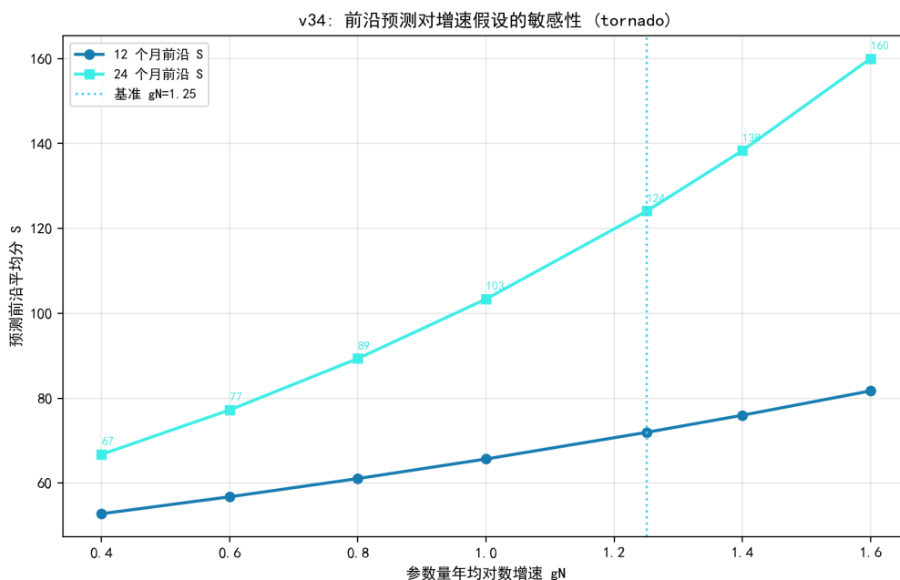
图 8.56 前沿预测对参数量增速假设 g_N 的敏感性（12/24 个月）。
