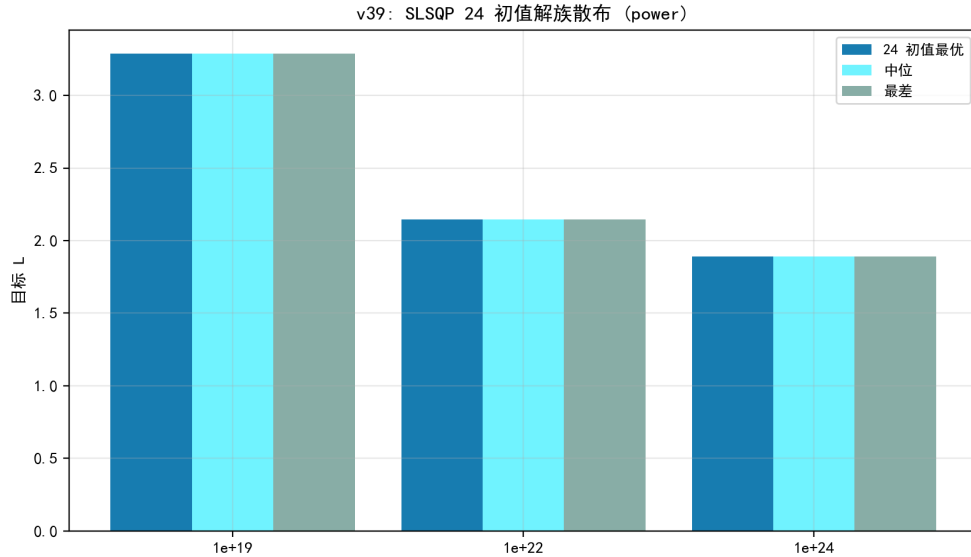
图 7.33 SLSQP 24 初值解族散布：三档预算全部初值收敛到同一最优。
