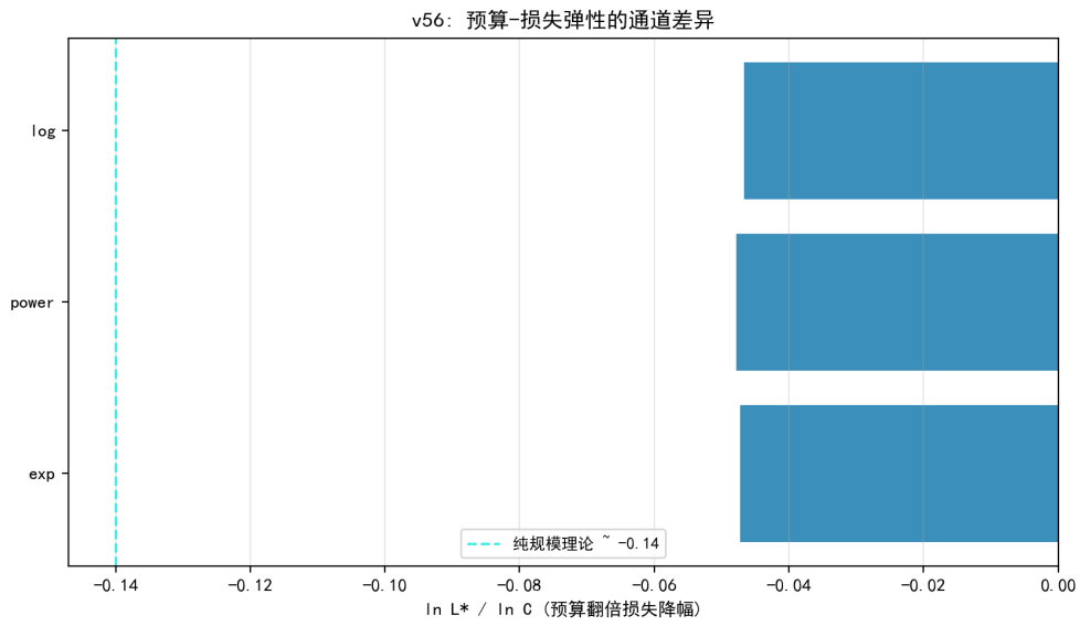
图 7.36 总损失口径的预算弹性：三形式几乎重合，低于超额口径斜率。
