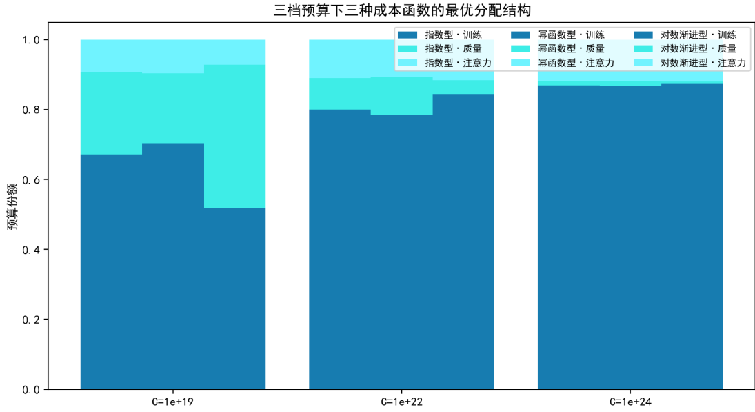
图 7.34 三档预算下三种质量成本函数的最优成本份额结构。
