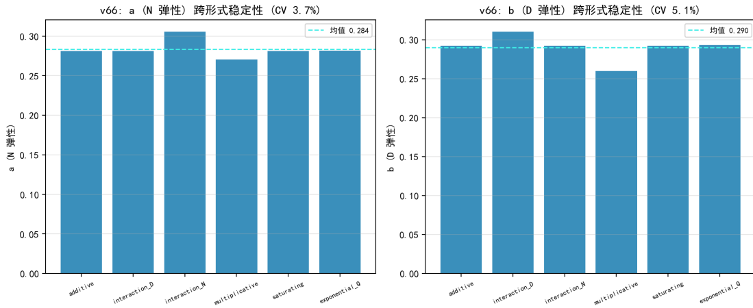
图 6.23 六形式共享参数：a/b 跨形式稳定（CV<6%）、 (1-Q)^g 族 g \approx 1 。
