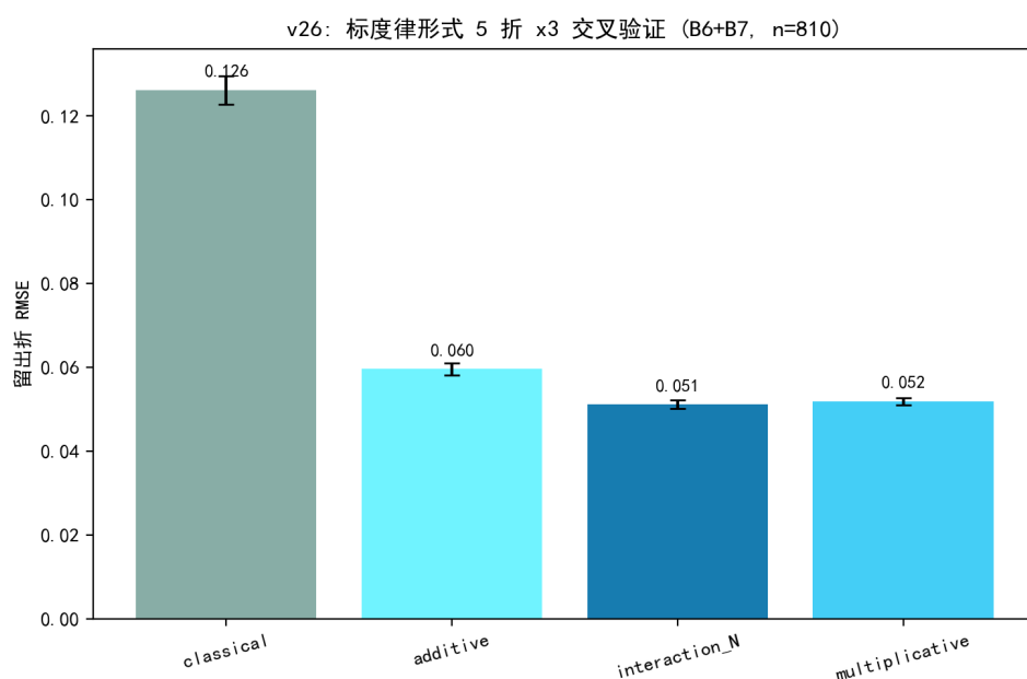
图 6.20 标度律形式 5 折交叉验证的留出 RMSE 对比。
