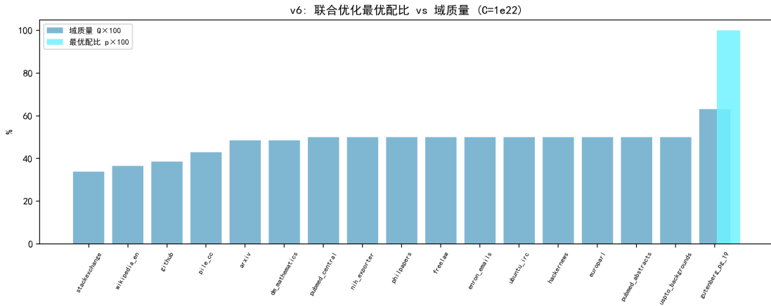
图 7.45 联合优化最优配比与域质量对比 ( C = 10^{22} )：配比向最高质量域 (小说) 集中。
