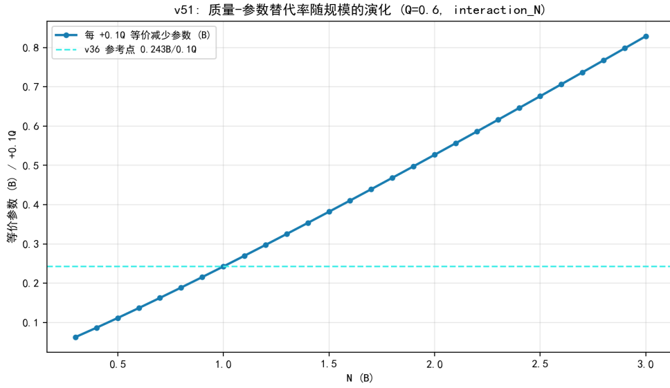
图 6.31 每 +0.1Q 等价减少的参数随规模的演化（近线性上升）。
