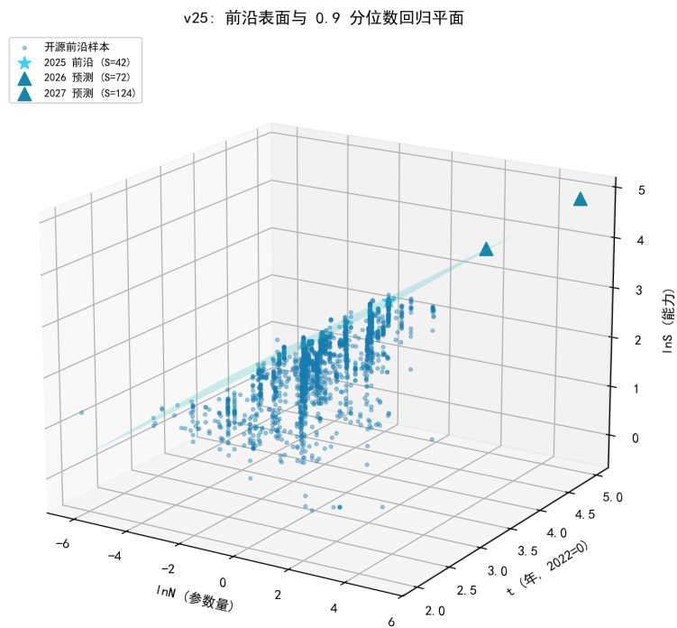
图 8.63 能力前沿 3D 表面与 0.9 分位数回归平面（星标 =2025 前沿，三角 = 预测点）。
