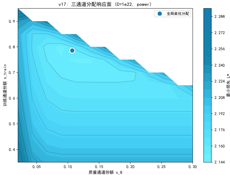
图 7.48 三通道分配响应面（ C = 10^{22} ，幂成本；蓝点为全局最优分配）。
