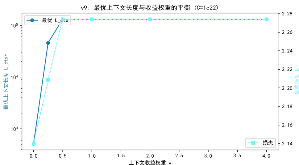
图 7.47 最优上下文长度与收益权重 w 的平衡 ( C = 10^{22} )。
