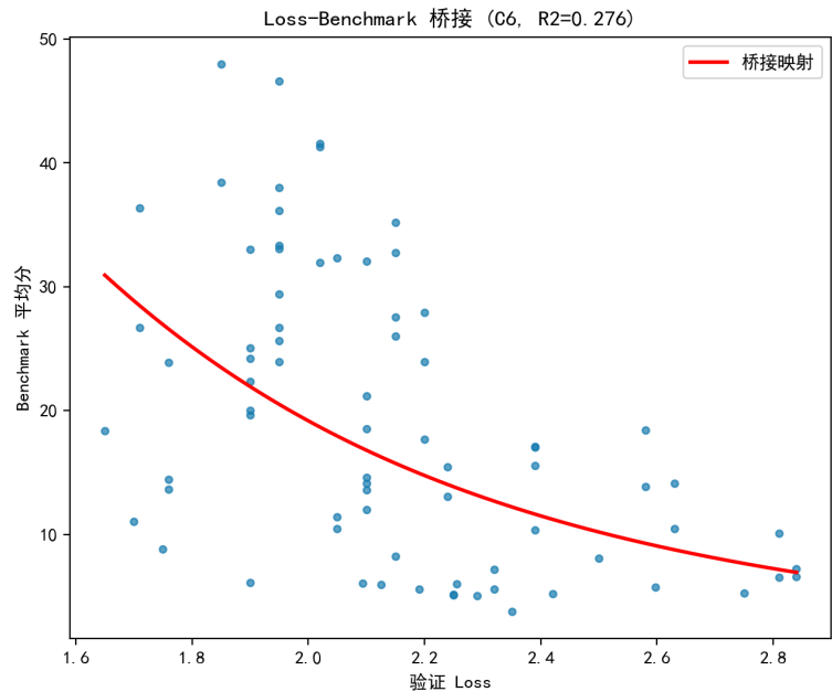
图 8.66 Loss-Benchmark 桥接映射（C6，75 个模型）。
