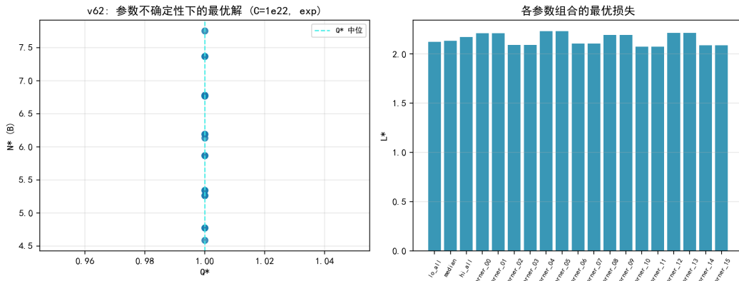
图 7.37 参数角点下的最优解： Q^*=1 稳定、 L^* 带宽 \pm 3.5\% 、 N^* \pm 28\% 。
