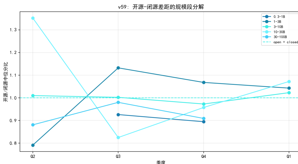
图 8.50 开源-闭源差距的规模段分解：中段持平、两端滞后约 10%。
