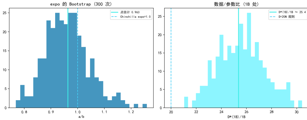
图 7.40 D^*(N) 参数 Bootstrap: 指数 CI 含 1.0, 常数 CI 高于 D = 20N 。
