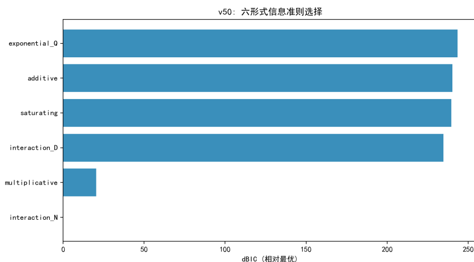
图 6.21 六种形式的 BIC/AIC 选择：interaction_N 决定性胜出。
