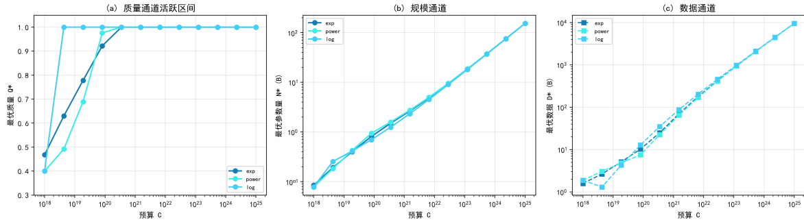
图 7.43 最优解族随预算轨迹：质量通道活跃区间由成本形式决定。
