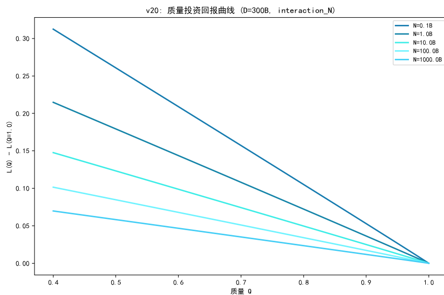
图 6.28 质量投资回报曲线（ D = 300B ）： L(Q) 相对 L(Q = 1) 随 N 变化。
