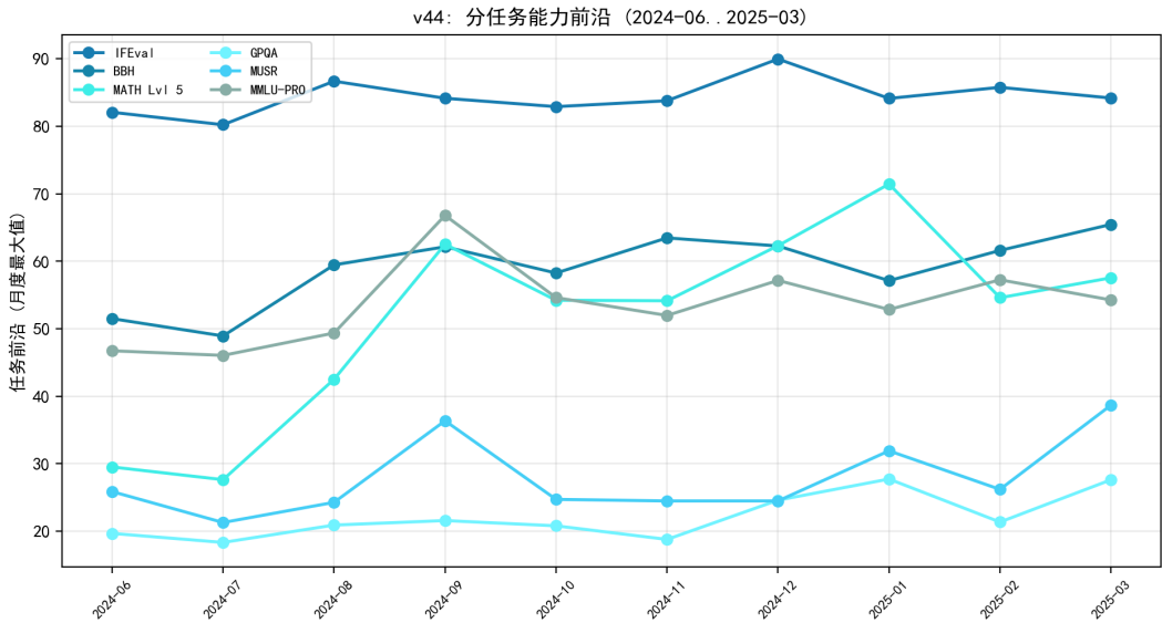
图 8.57 分任务能力前沿：推理类（MATH/GPQA/MUSR）增长快于知识/指令类。
