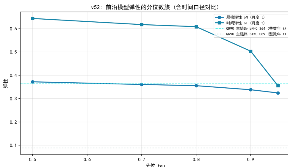
图 9.68 前沿弹性的分位数族与时间口径对比（ b_N 稳健， b_T 对口径敏感）。
