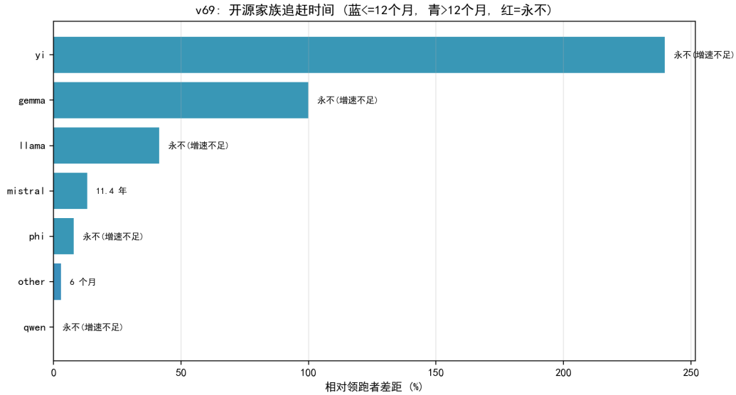
图 8.52 家族追赶时间：仅 other 可短期追平，Llama 近乎停滞。
