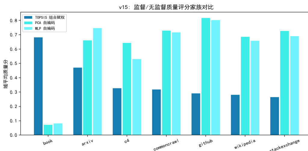
图 9.70 TOPSIS 组合赋权与自编码典型性评分的域级对照（方向相反）。
