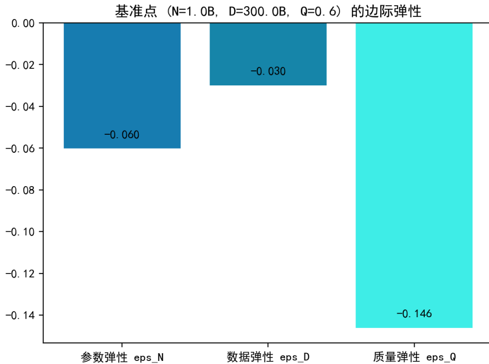
图 6.29 基准点处三个维度的损失弹性对比（质量弹性最高）。
