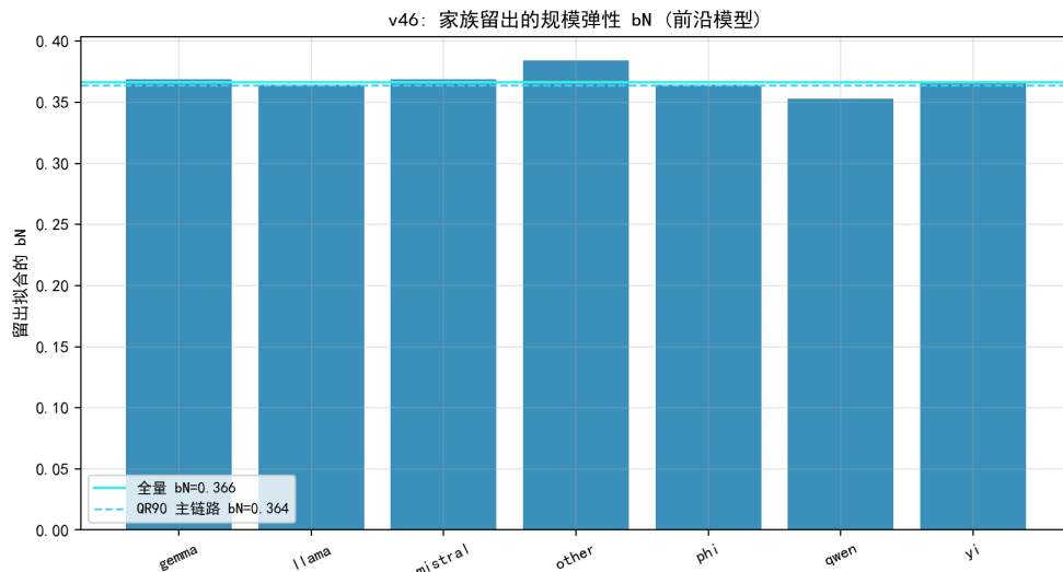
图 8.64 家族留出的规模弹性 b_N ：全家族稳定在 0.36 附近。
