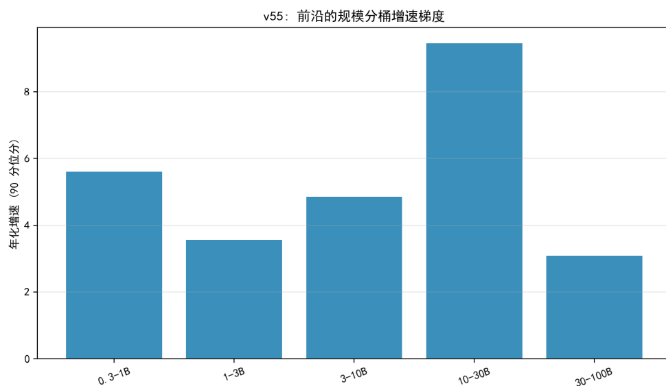
图 8.58 规模分桶的前沿年化增速：10–30B 甜点区最快，30–100B 最慢。
