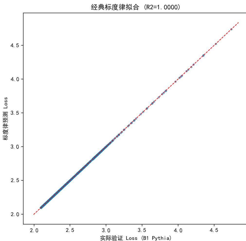
图 6.19 经典标度律在 B1 轨迹上的拟合与跨家族验证。
