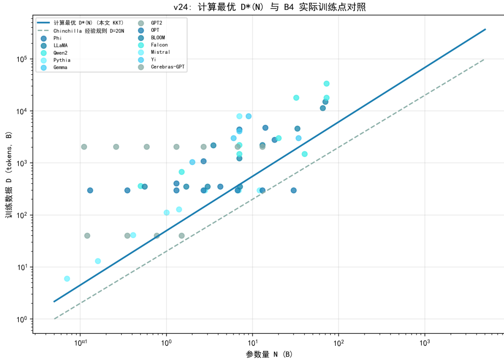
图 7.39 计算最优数据曲线 D^*(N) 、Chinchilla 经验规则与 B4 实际训练点。
