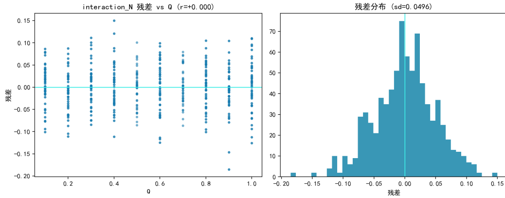
图 6.22 interaction_N 残差诊断：与 Q 无相关、分布近对称。
