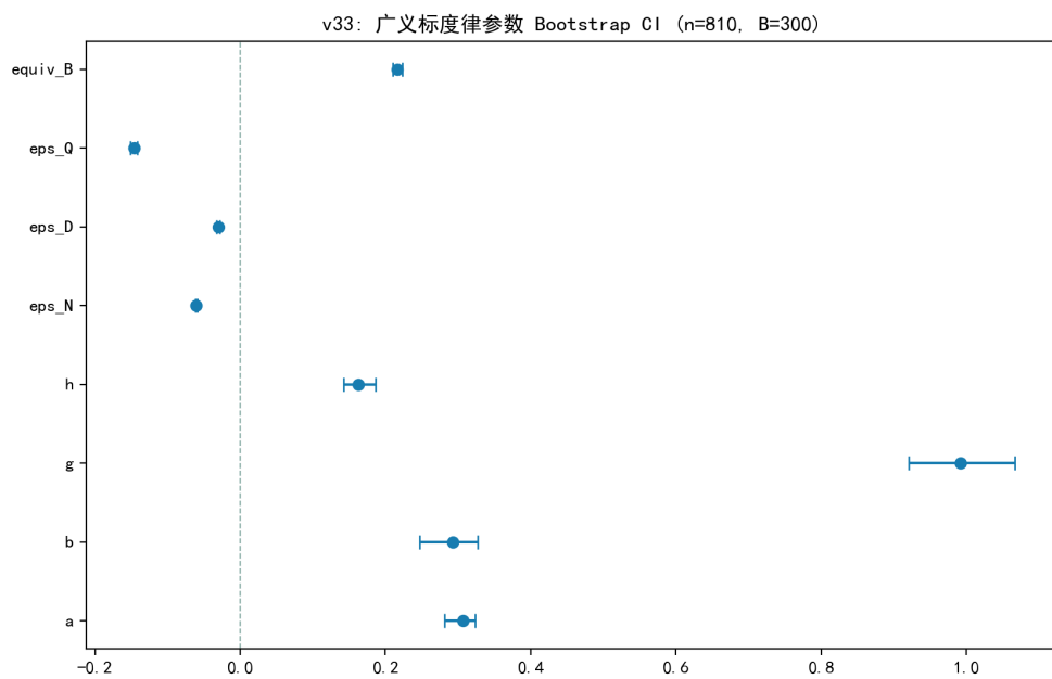
图 6.25 广义标度律参数与弹性的 Bootstrap 置信区间。
