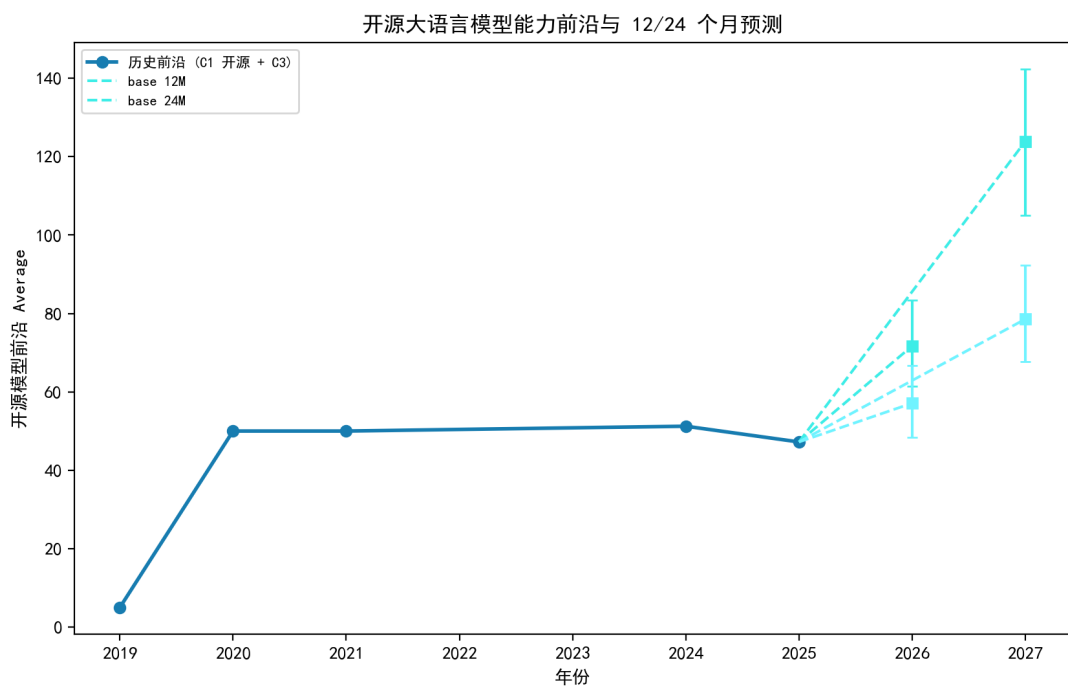
图 8.62 开源模型能力前沿（历史点）与 12/24 个月预测（基础/放缓情景，90% 区间）。
