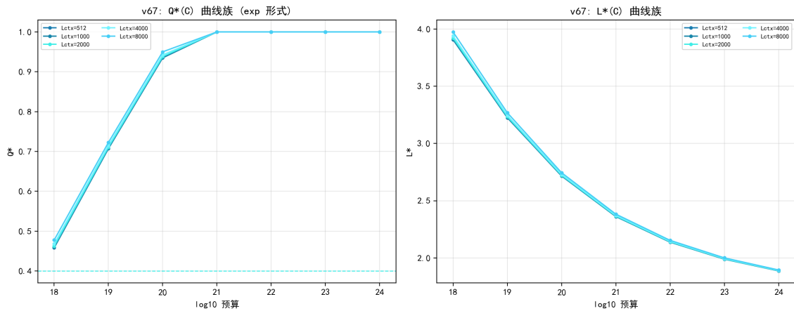
图 7.38 上下文长度 \times 预算响应面： L^* 路径几乎不随 L_{ctx} 移动。
