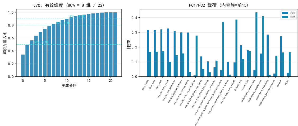
图 5.18 22 指标的有效维度 (80%=8 维) 与 PC1/PC2 载荷：两族互补。
