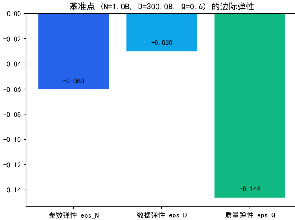
图 6.8 基准点处三个维度的损失弹性对比（质量弹性最高）。
