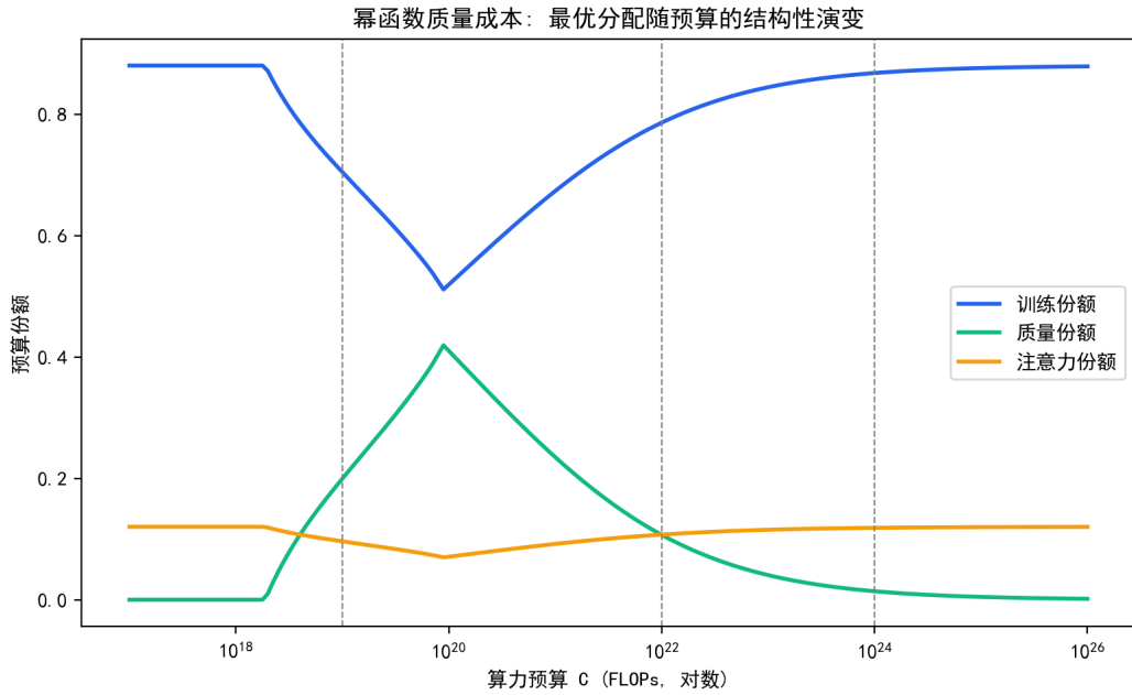
图 7.10 幂函数质量成本下最优成本份额随预算的结构性演变（竖线为三档预算）。
