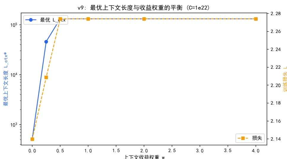
图 7.13 最优上下文长度与收益权重 w 的平衡 ( C = 10^{22} )。
