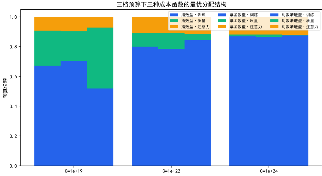
图 7.9 三档预算下三种质量成本函数的最优成本份额结构。
