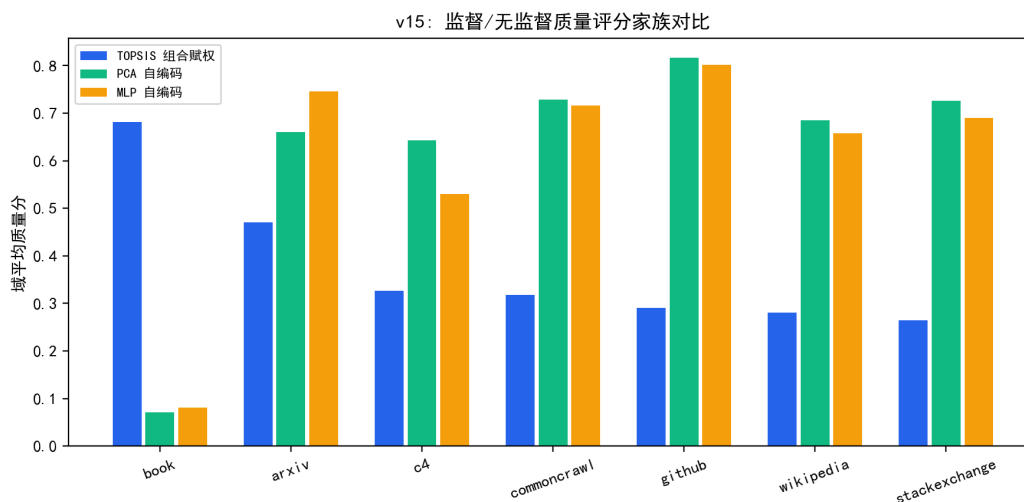
图 9.20 TOPSIS 组合赋权与自编码典型性评分的域级对照（方向相反）。
