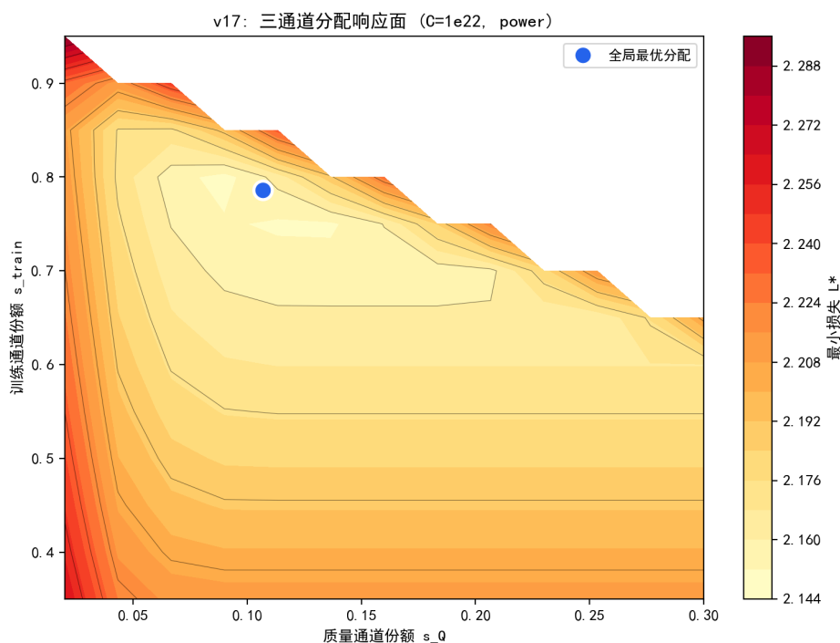
图 7.14 三通道分配响应面 ( C = 10^{22} , 幂成本; 蓝点为全局最优分配)。
