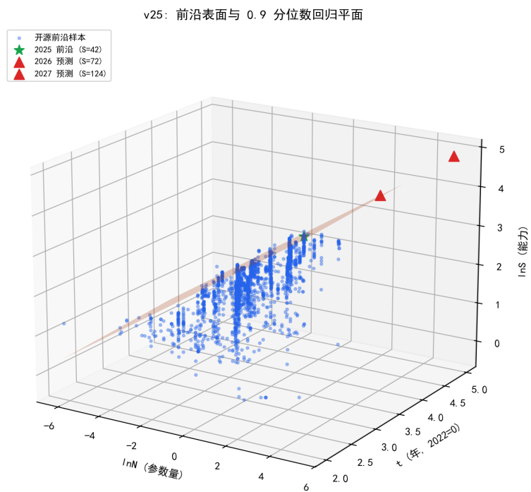
图 8.31 能力前沿 3D 表面与 0.9 分位数回归平面（星标 =2025 前沿，三角 = 预测点）。
