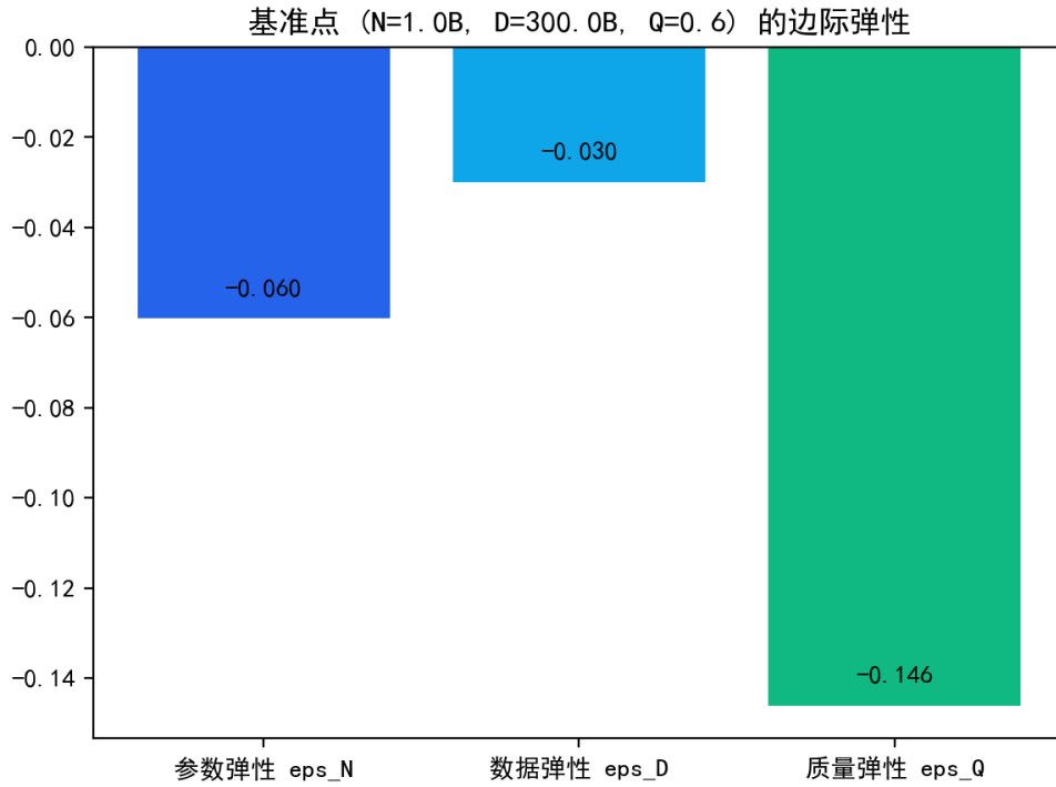
图 6.16 基准点处三个维度的损失弹性对比（质量弹性最高）。
