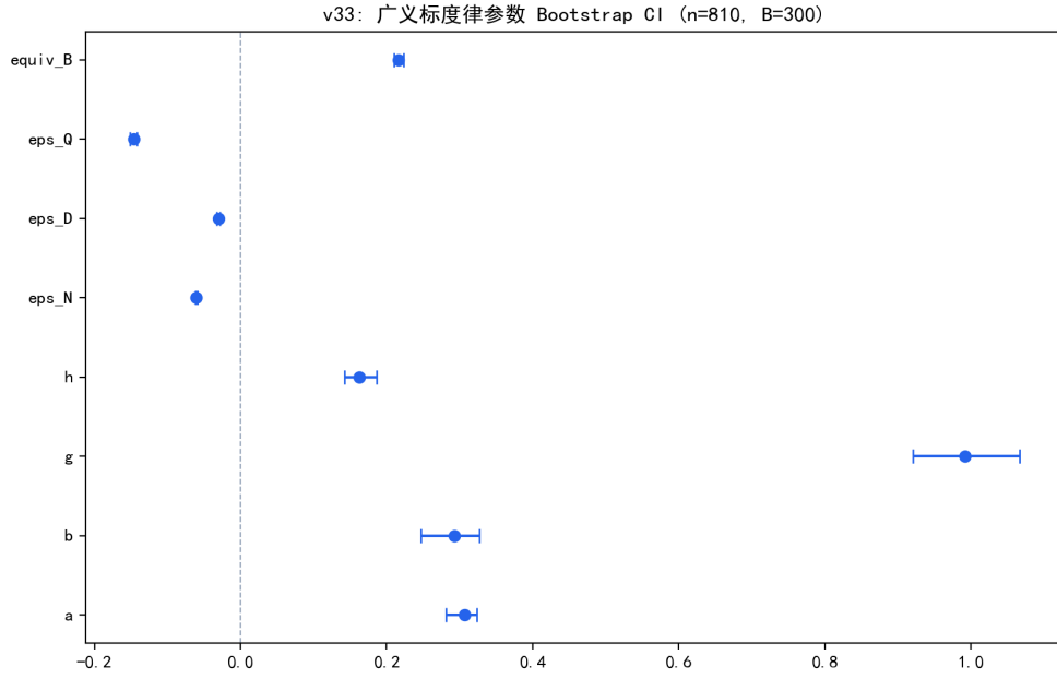
图 6.13 广义标度律参数与弹性的 Bootstrap 置信区间。
