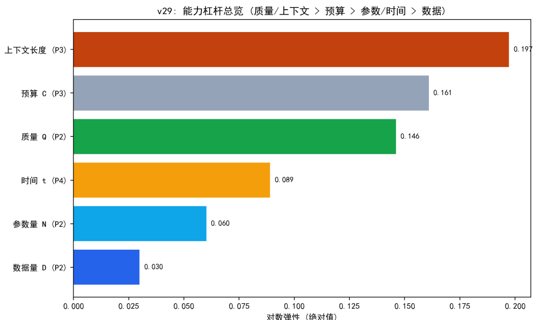
图 10.37 能力杠杆总览：各投入的对数弹性排序（质量/上下文 > 预算 > 参数/时间 > 数据）。
