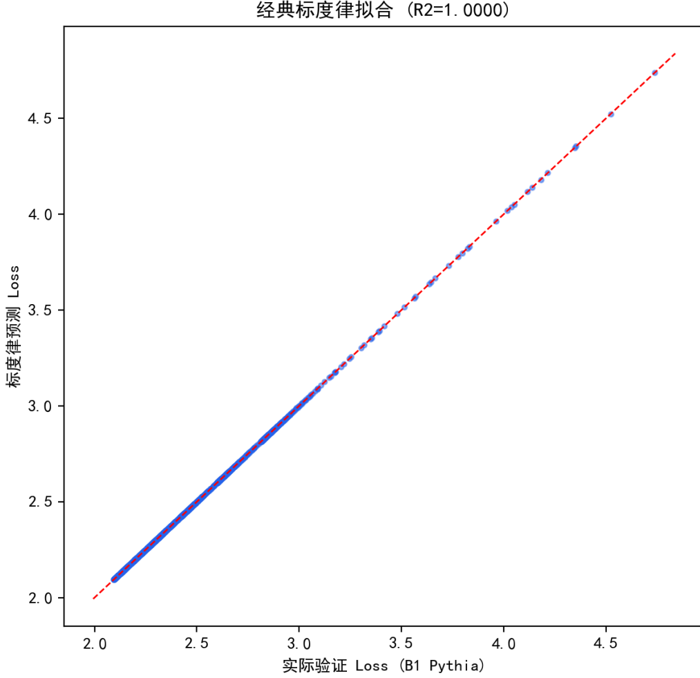
图 6.10 经典标度律在 B1 轨迹上的拟合与跨家族验证。
