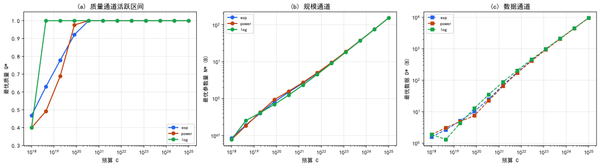
图 7.22 最优解族随预算轨迹：质量通道活跃区间由成本形式决定。
