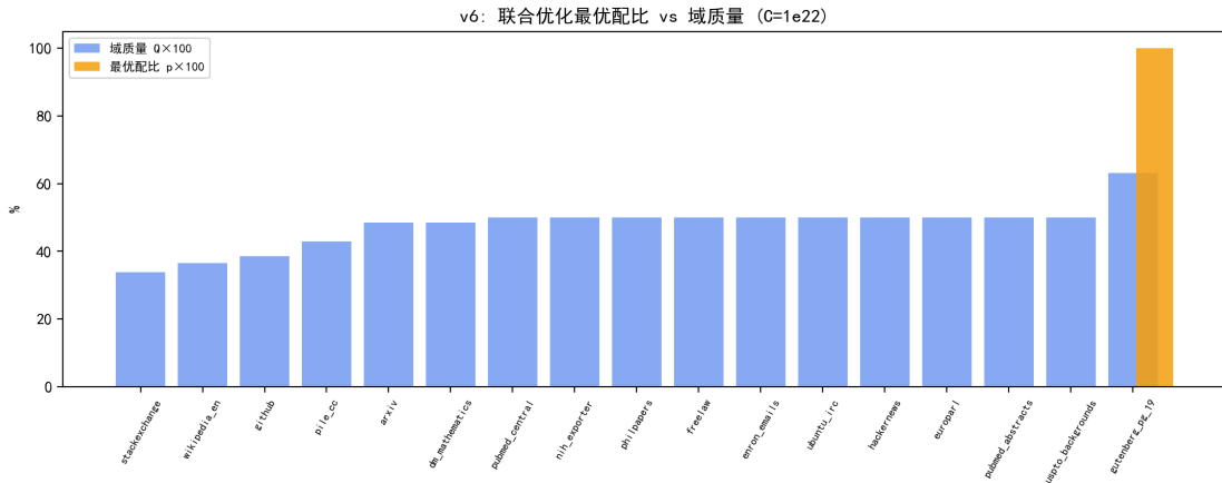
图 7.24 联合优化最优配比与域质量对比（ C = 10^{22} ）：配比向最高质量域（小说）集中。
