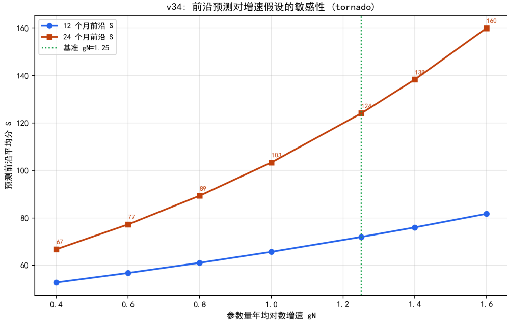
图 8.28 前沿预测对参数量增速假设 g_N 的敏感性（12/24 个月）。
