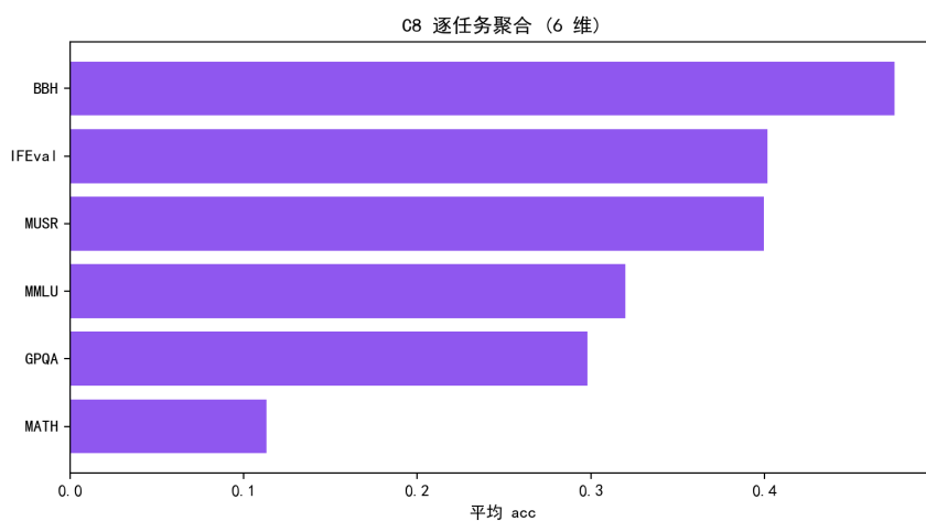
图 8.34 C8 逐任务聚合得分 (6 维)。
