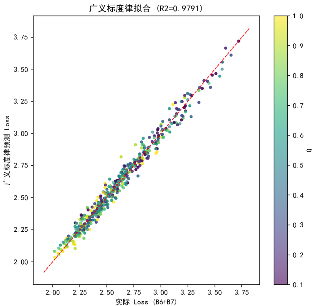
图 6.12 广义标度律在 B6+B7 数据上的拟合（质量-参数数量交互形式， R^2 = 0.979 ）。
