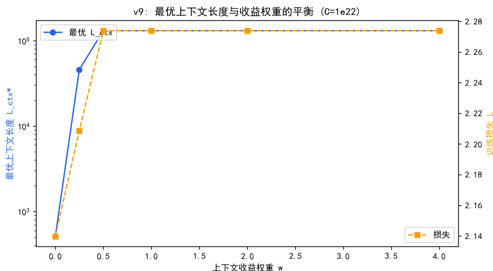
图 7.26 最优上下文长度与收益权重 w 的平衡 ( C = 10^{22} )。
