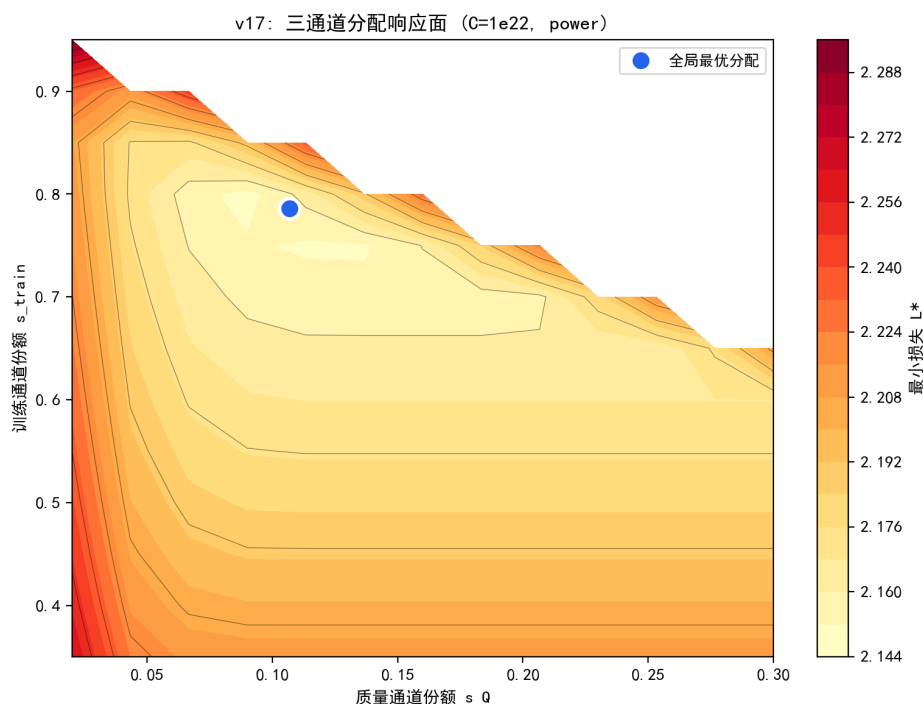
图 7.27 三通道分配响应面（ C = 10^{22} ，幂成本；蓝点为全局最优分配）。
