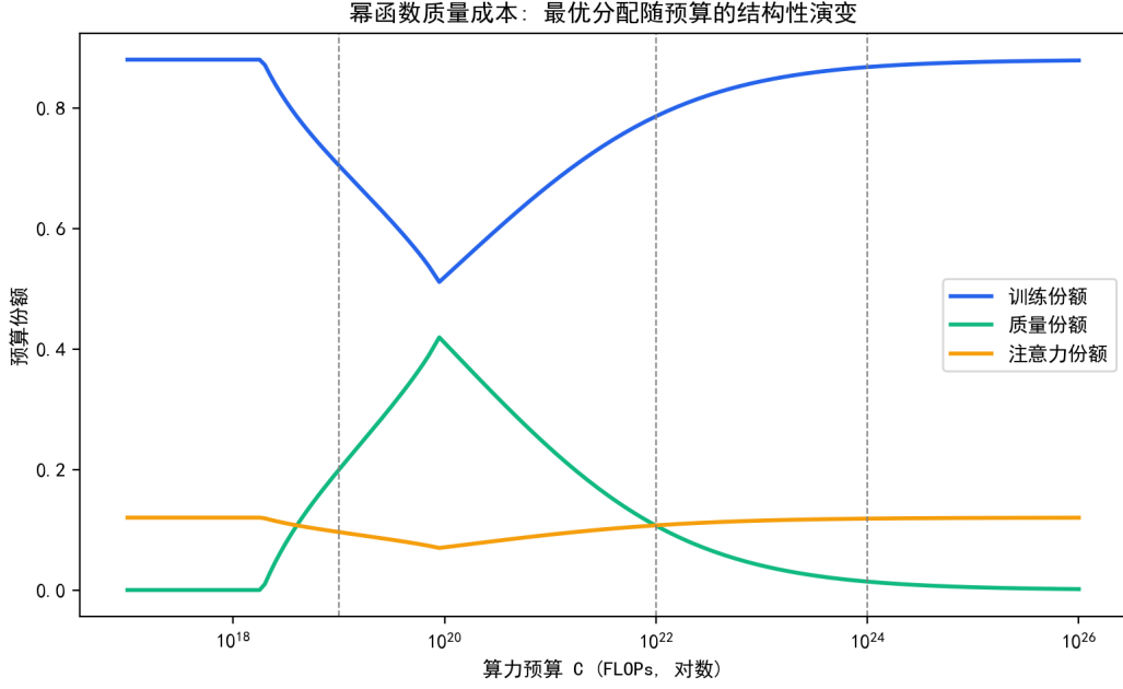
图 7.21 幂函数质量成本下最优成本份额随预算的结构性演变（竖线为三档预算）。
