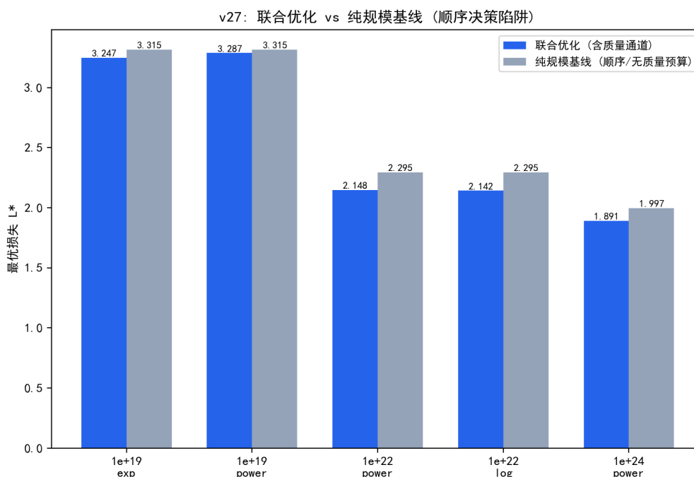
图 7.25 联合优化 vs 纯规模基线的最优损失（顺序决策陷阱：质量需预算预留）。
