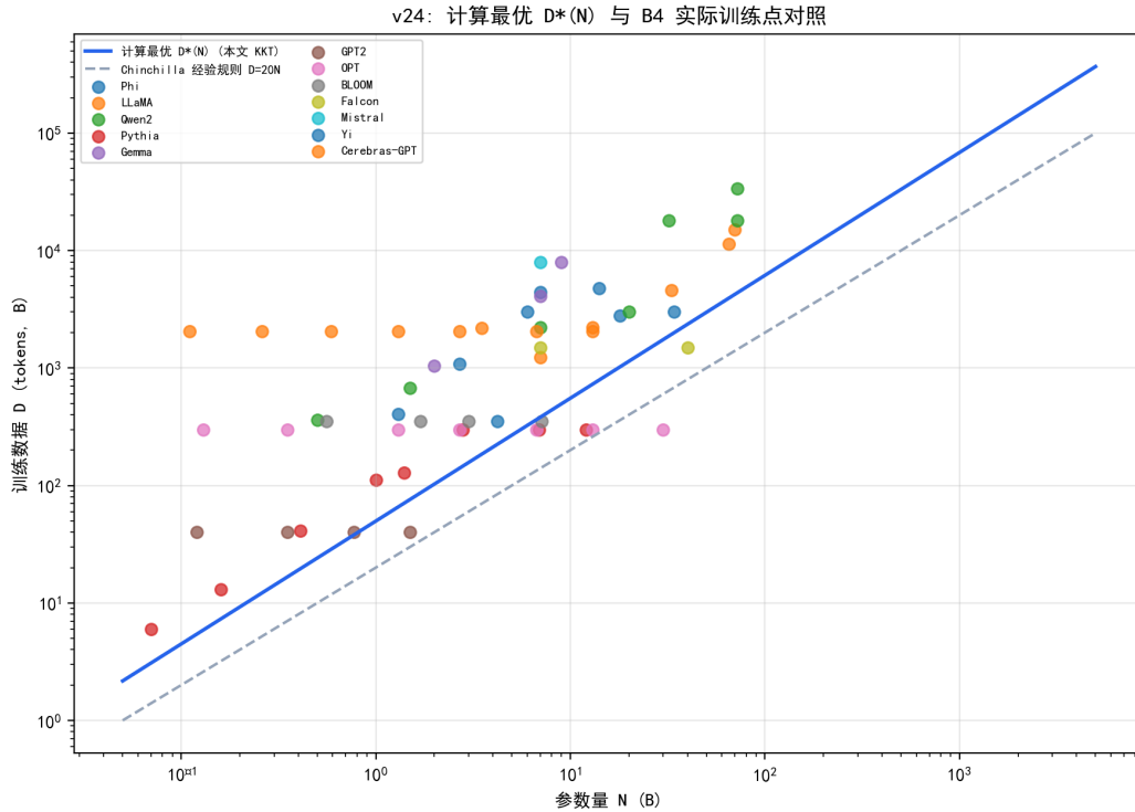
图 7.20 计算最优数据曲线 D^*(N) 、Chinchilla 经验规则与 B4 实际训练点。
