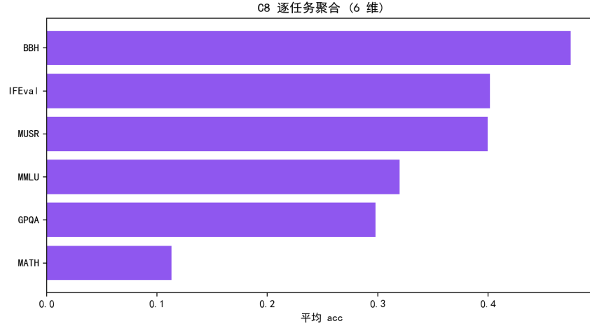
图 8.16 C8 逐任务聚合得分（6 维）。
