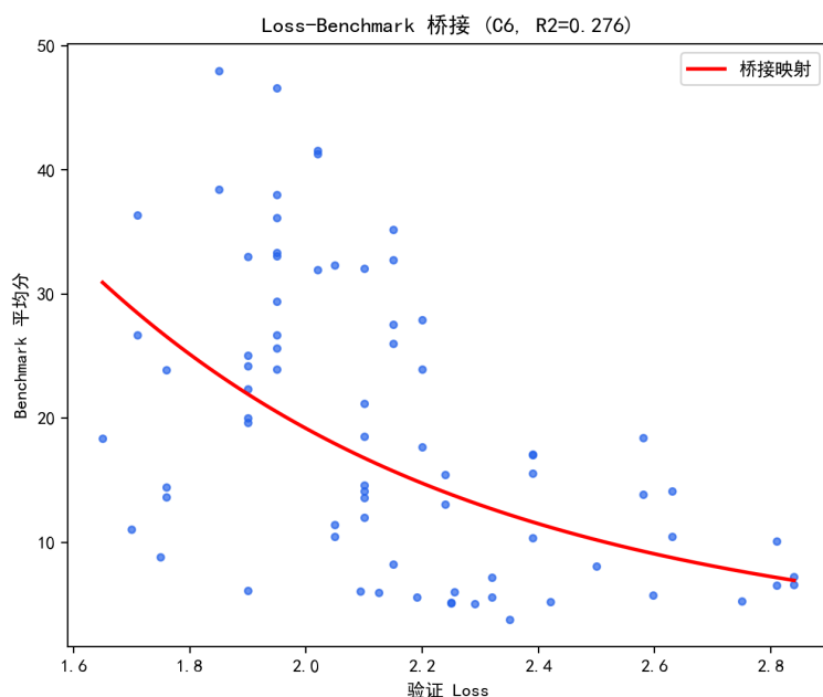
图 8.15 Loss-Benchmark 桥接映射（C6，75 个模型）。
