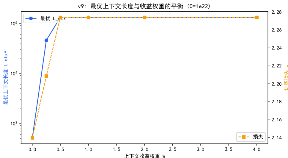
图 7.12 最优上下文长度与收益权重 w 的平衡（ C = 10^{22} ）。
