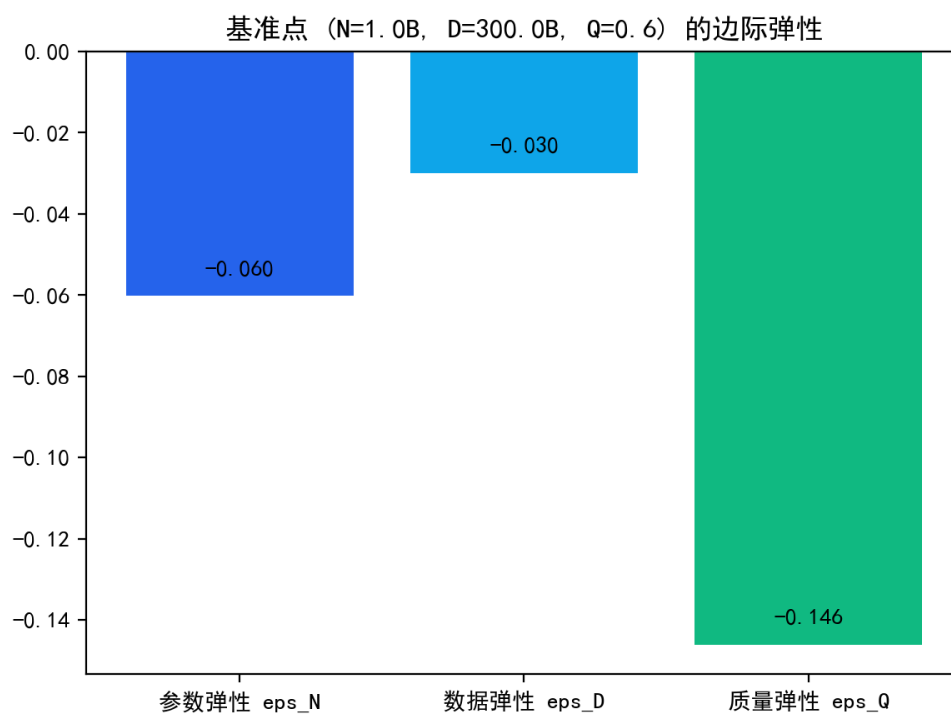
图 6.7 基准点处三个维度的损失弹性对比（质量弹性最高）。
