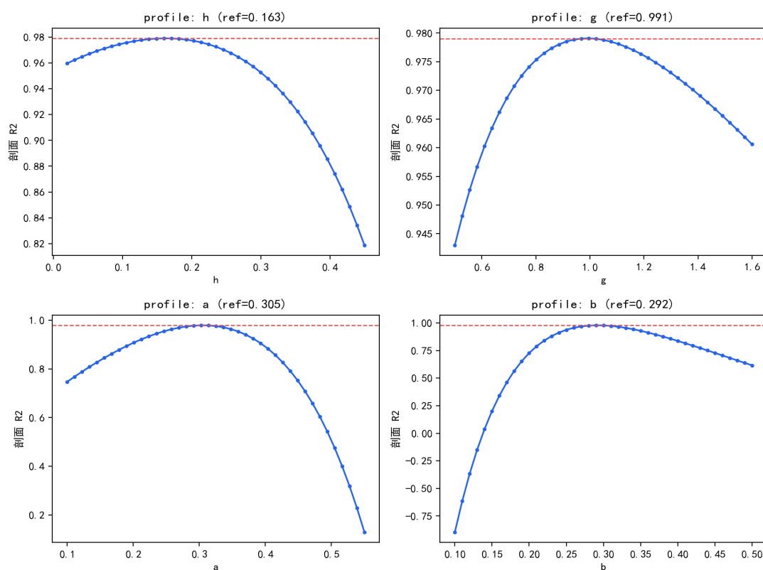
图 6.6 关键参数的剖面似然曲线（红色虚线为 90% 似然比阈值）。
