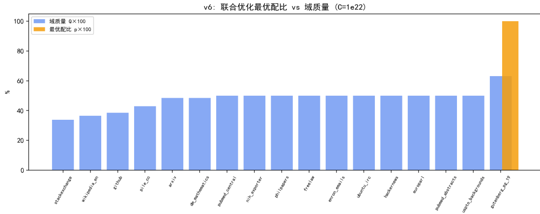
图 7.11 联合优化最优配比与域质量对比（ C = 10^{22} ）：配比向最高质量域（小说）集中。
