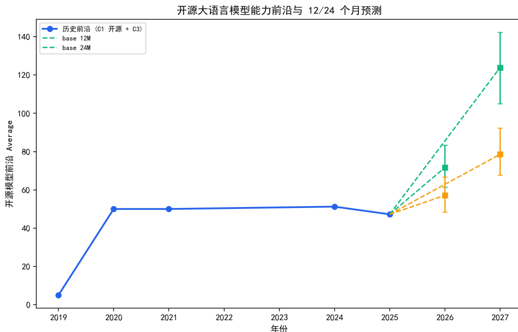
图 8.13 开源模型能力前沿（历史点）与 12/24 个月预测（基础/放缓情景，90% 区间）。
