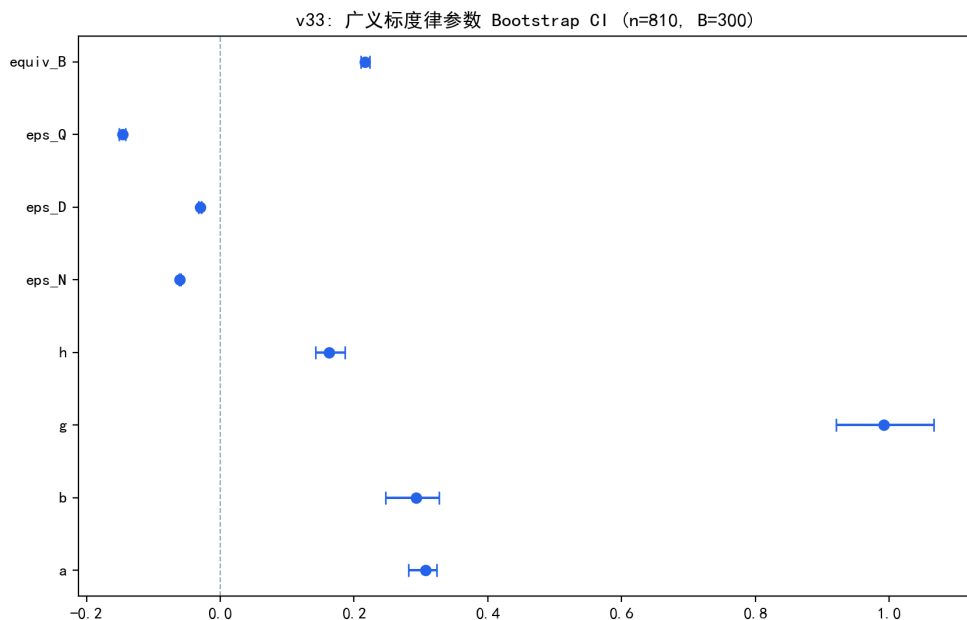
图 6.22 广义标度律参数与弹性的 Bootstrap 置信区间。
