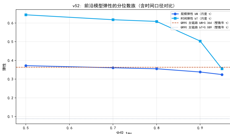
图 9.60 前沿弹性的分位数族与时间口径对比 (bN 稳健, bT 对口径敏感)。
