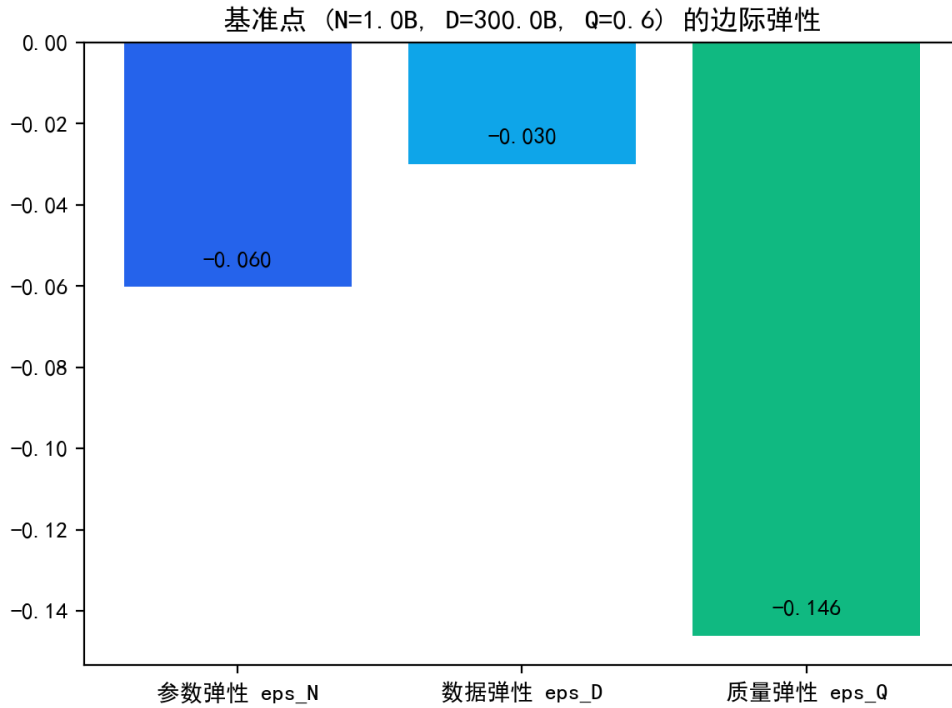
图 6.26 基准点处三个维度的损失弹性对比（质量弹性最高）。
