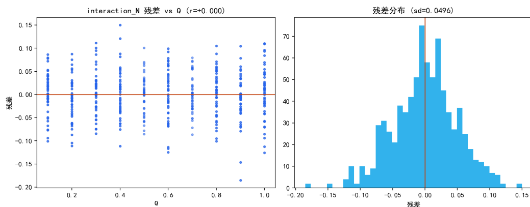
图 6.20 interaction_N 残差诊断：与 Q 无相关、分布近对称。
