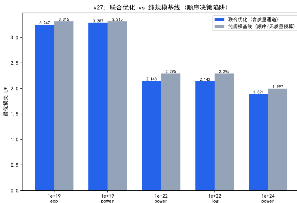
图 7.42 联合优化 vs 纯规模基线的最优损失（顺序决策陷阱：质量需预算预留）。
