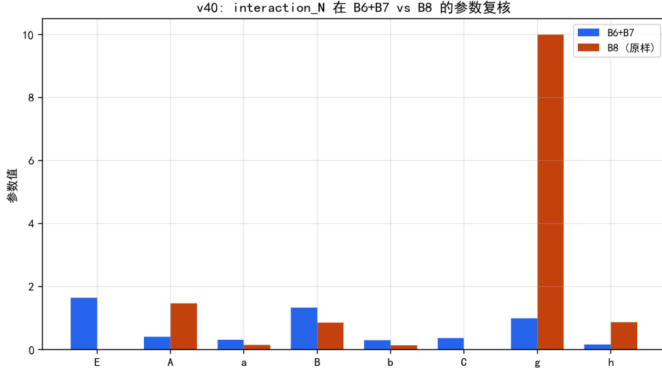
图 6.23 B8 原样 vs B6+B7 的参数对比：B8 质量项退化（ E = C = 0 ， g 撞界）。
