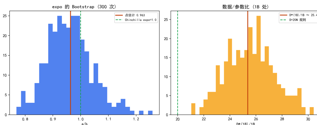
图 7.36 D^*(N) 参数 Bootstrap: 指数 CI 含 1.0, 常数 CI 高于 D = 20N 。
