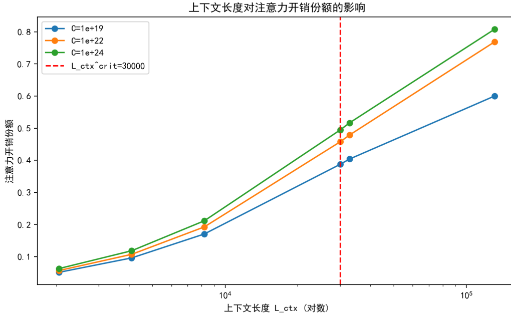
图 7.40 注意力开销份额随上下文长度的变化（红色虚线为临界点 30000）。
