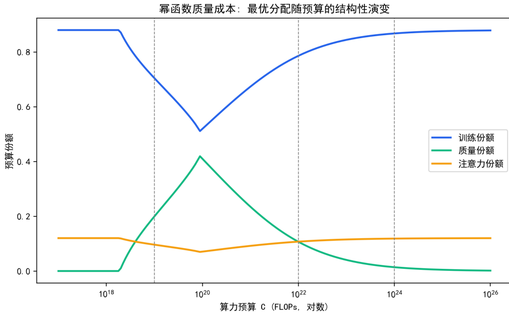
图 7.38 幂函数质量成本下最优成本份额随预算的结构性演变（竖线为三档预算）。
