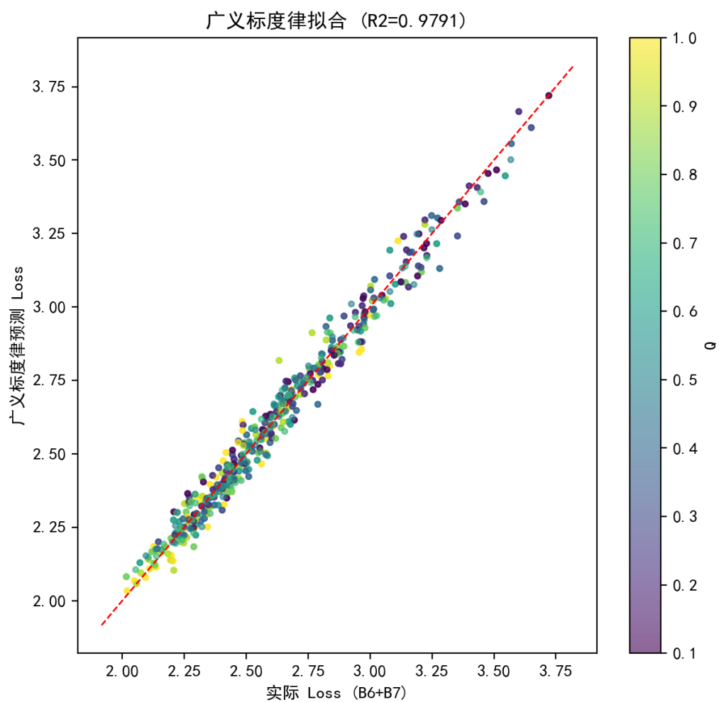
图 6.21 广义标度律在 B6+B7 数据上的拟合（质量-参数量交互形式， R^2 = 0.979 ）。
