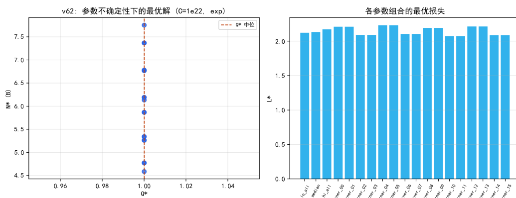
图 7.34 参数角点下的最优解： Q^*=1 稳定、 L^* 带宽 \pm 3.5\% 、 N^* \pm 28\% 。
