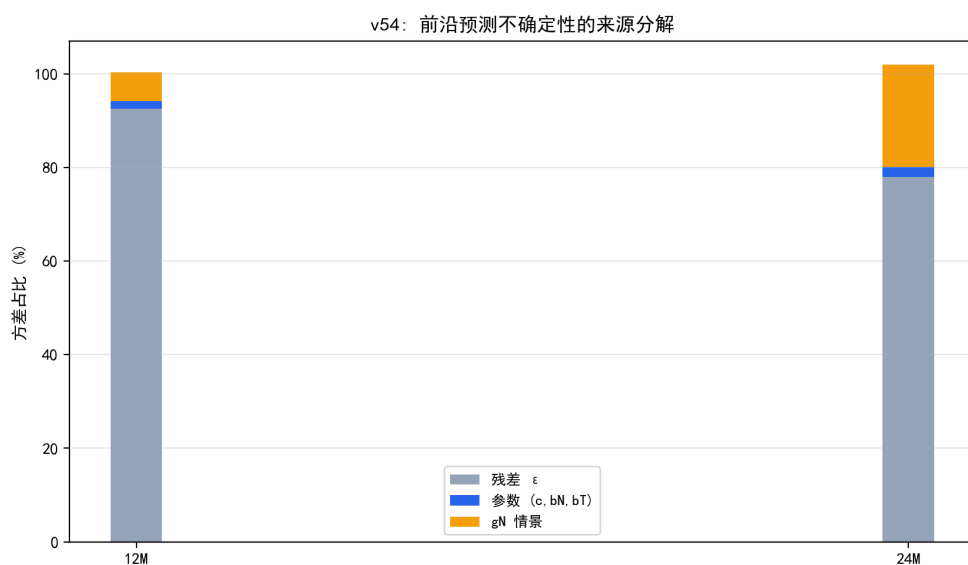
图 8.48 前沿预测不确定性的来源分解（12M/24M）。
