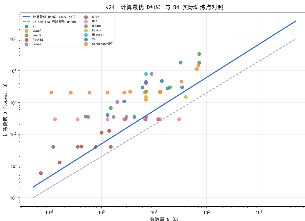
图 7.35 计算最优数据曲线 D^*(N) 、Chinchilla 经验规则与 B4 实际训练点。
