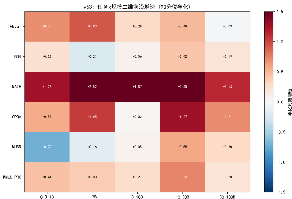
图 8.52 任务 × 规模二维前沿增速：MATH/GPQA 在 1–3B 与 10–30B 双峰。
