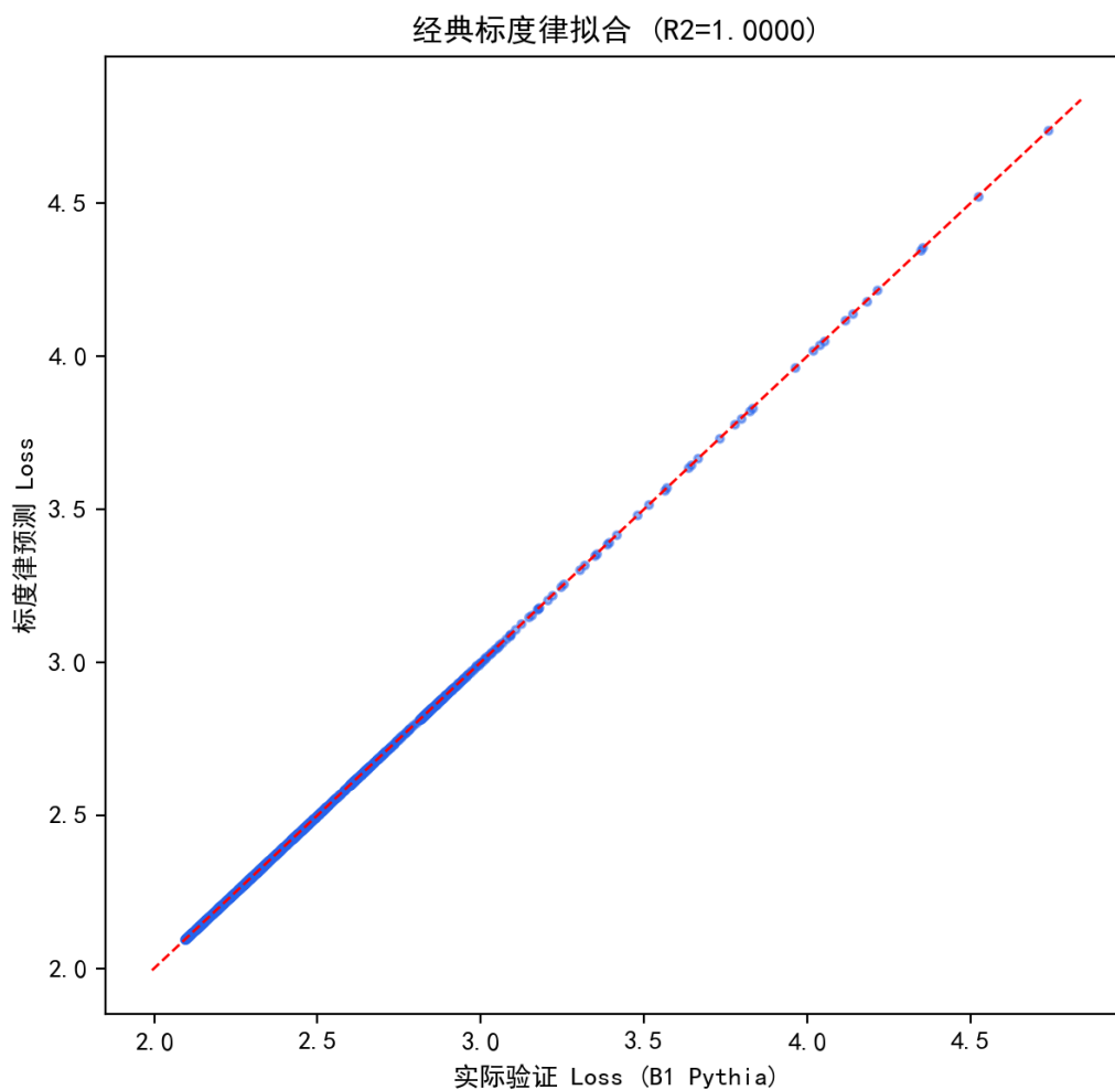
图 6.17 经典标度律在 B1 轨迹上的拟合与跨家族验证。
