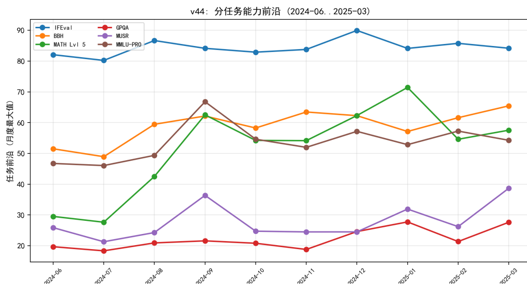
图 8.50 分任务能力前沿：推理类（MATH/GPQA/MUSR）增长快于知识/指令类。
