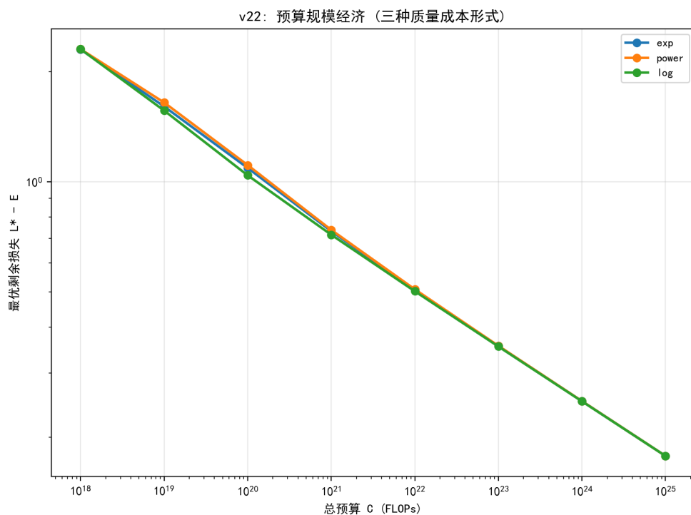
图 7.32 预算-最优损失的对数线性规律（三种质量成本形式）。
