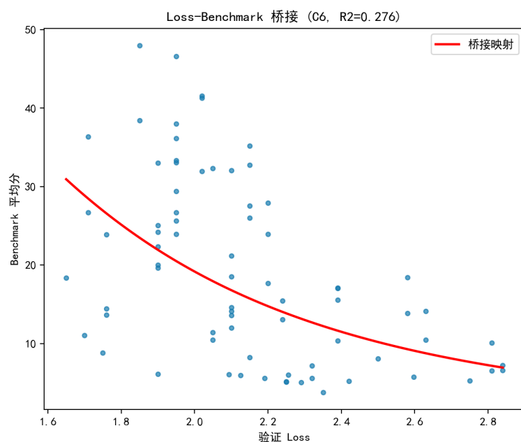
图 8.70 Loss-Benchmark 桥接映射 (C6, 75 个模型)。
