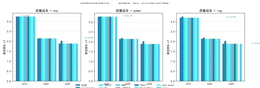
图 7.37 九框架求解对比：SLSQP/COBYLA/DE/SHGO/L-BFGS-B/Powell/Nelder-Mead/ 双退火/网格在 9 实例上一致到 10^{-6} 量级（括号为九路径最大相对偏差）， trust-constr 内点法在边界角点最优处失稳。
