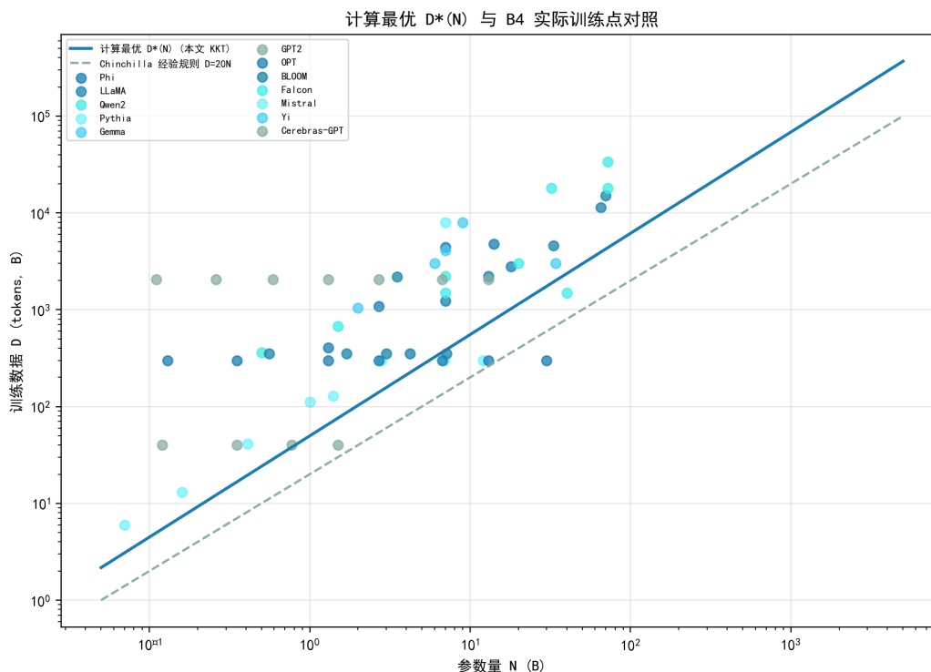
图 7.43 计算最优数据曲线 D^*(N) 、Chinchilla 经验规则与 B4 实际训练点。
