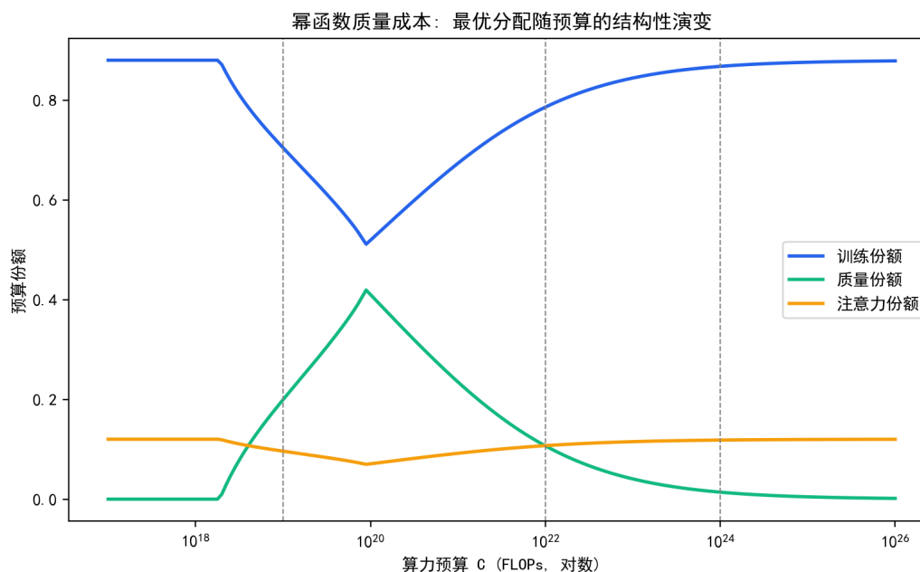
图 7.27 幂函数质量成本下最优成本份额随预算的结构性演变（竖线为三档预算）。
