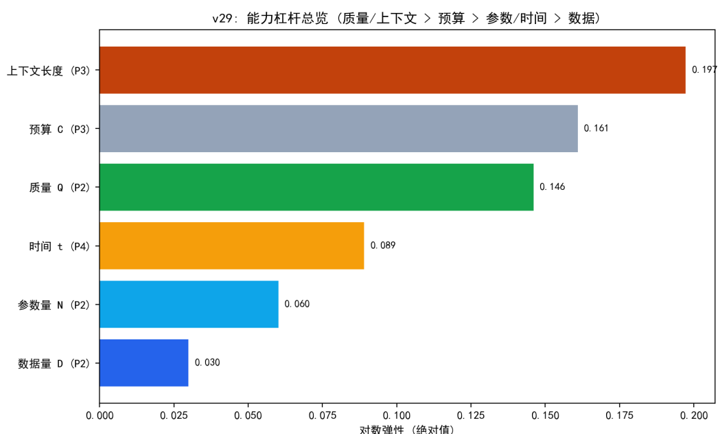
图 10.47 能力杠杆总览：各投入的对数弹性排序（质量/上下文 > 预算 > 参数/时间 > 数据）。
