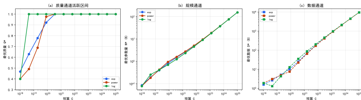
图 7.28 最优解族随预算轨迹：质量通道活跃区间由成本形式决定。
