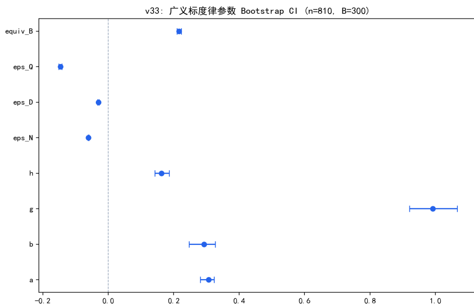
图 6.16 广义标度律参数与弹性的 Bootstrap 置信区间。
