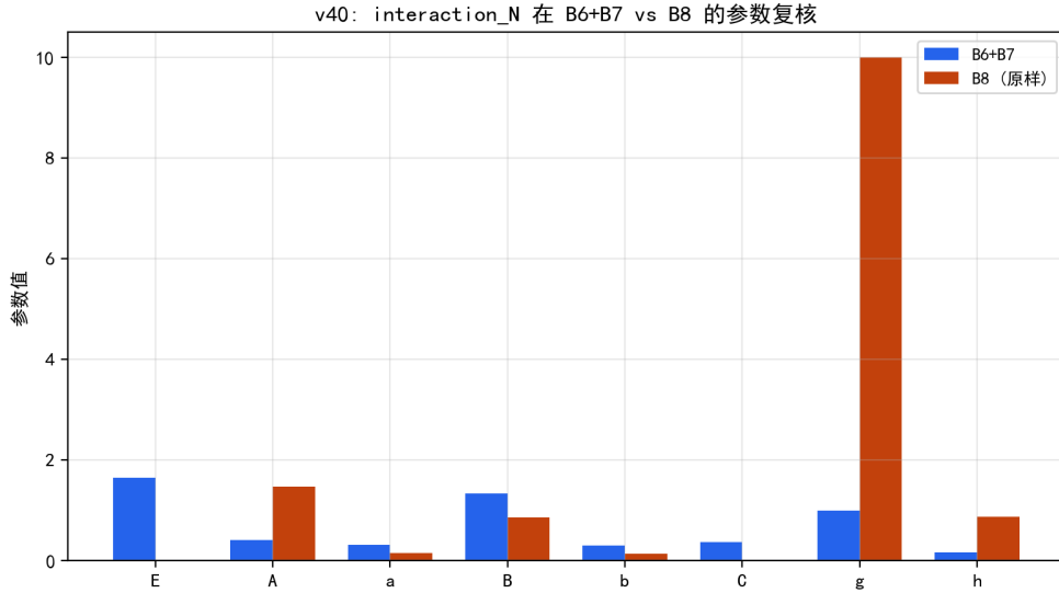
图 6.17 B8 原样 vs B6+B7 的参数对比：B8 质量项退化（ E = C = 0 ， g 撞界）。
