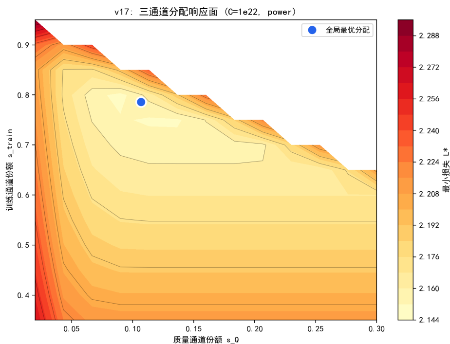
图 7.33 三通道分配响应面 ( C = 10^{22} ，幂成本；蓝点为全局最优分配)。
