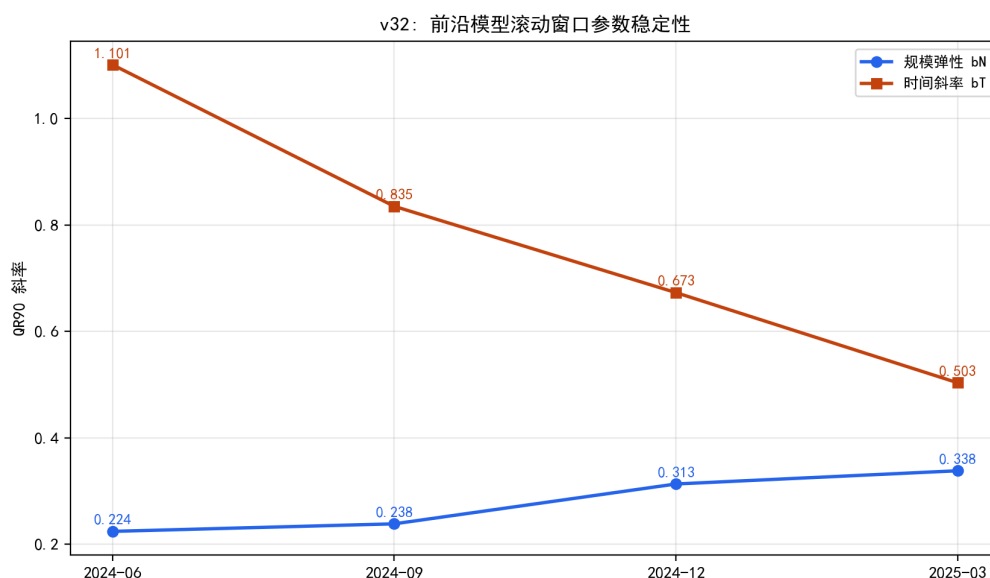
图 8.38 前沿 QR90 滚动窗口参数：规模弹性上升、时间斜率持续下降。
