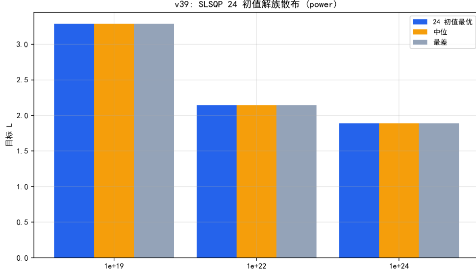
图 7.23 SLSQP 24 初值解族散布：三档预算全部初值收敛到同一最优。
