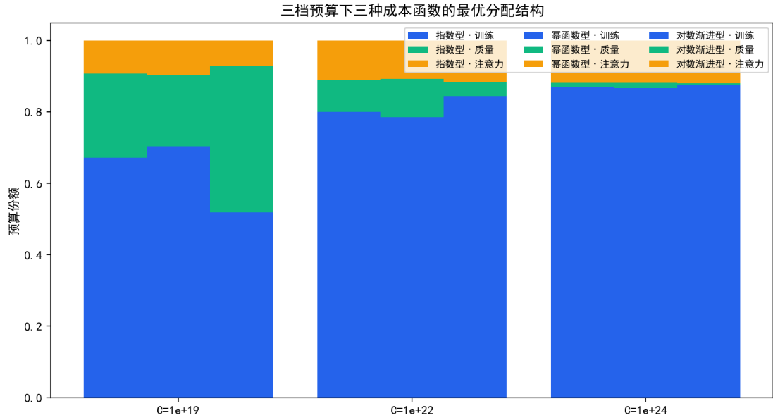
图 7.24 三档预算下三种质量成本函数的最优成本份额结构。
