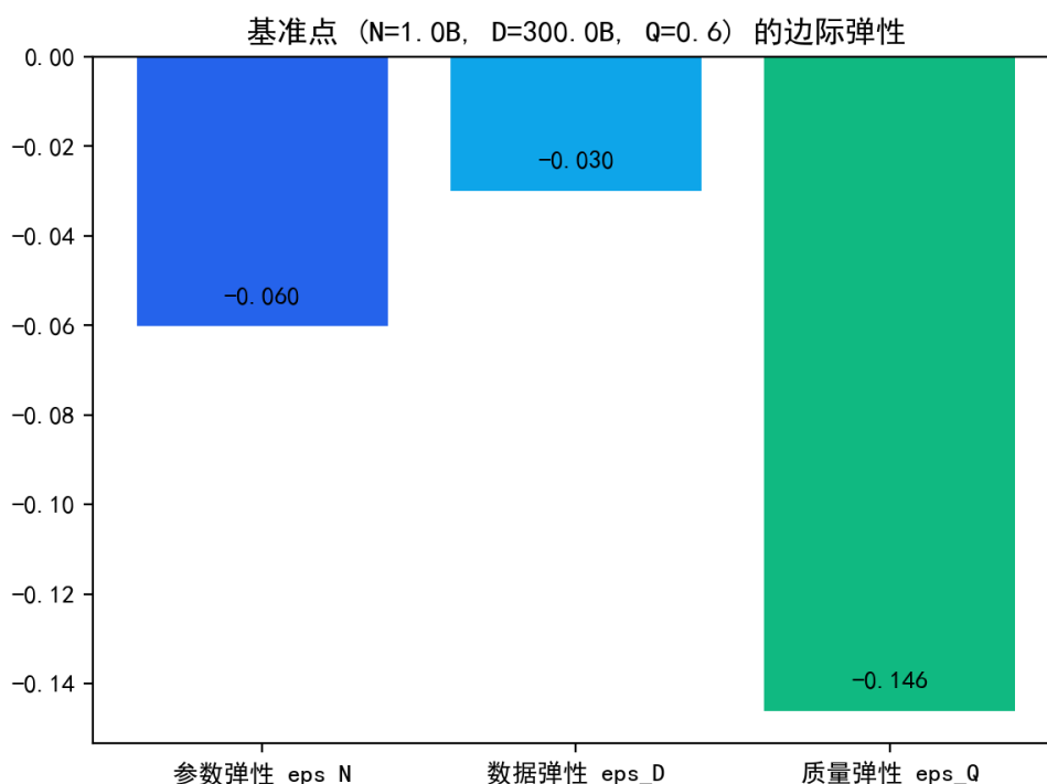
图 6.20 基准点处三个维度的损失弹性对比（质量弹性最高）。
