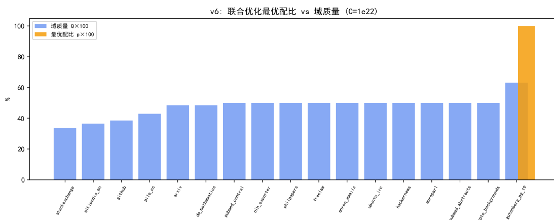
图 7.30 联合优化最优配比与域质量对比（ C = 10^{22} ）：配比向最高质量域（小说）集中。
