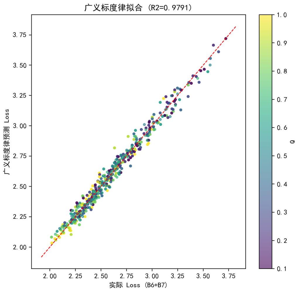
图 6.15 广义标度律在 B6+B7 数据上的拟合（质量-参数数量交互形式， R^2 = 0.979 ）。
