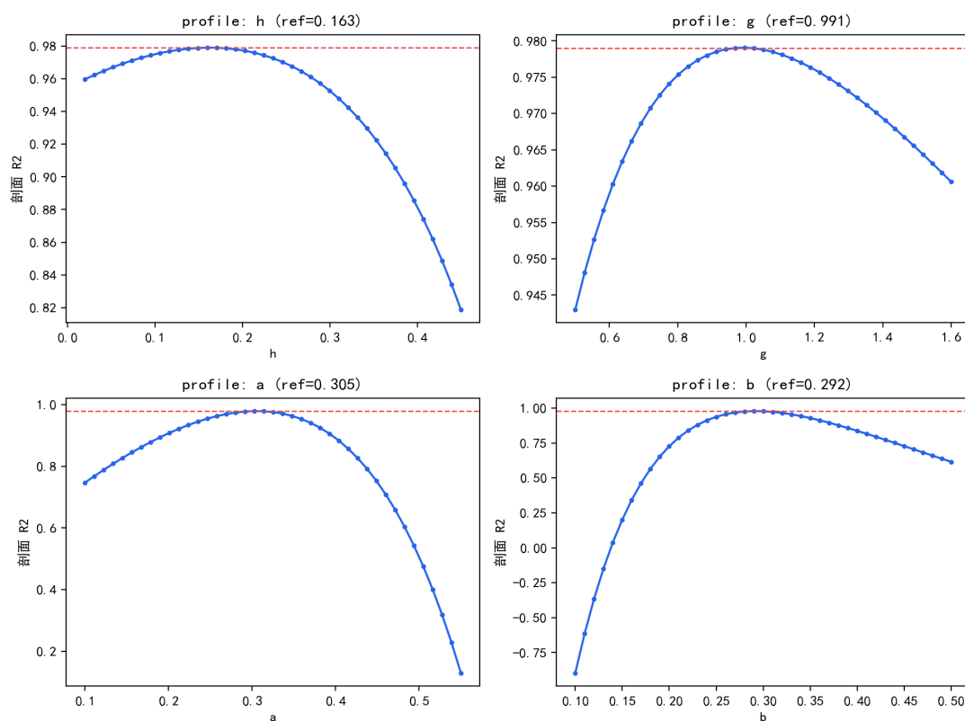
图 6.18 关键参数的剖面似然曲线（红色虚线为 90% 似然比阈值）。
