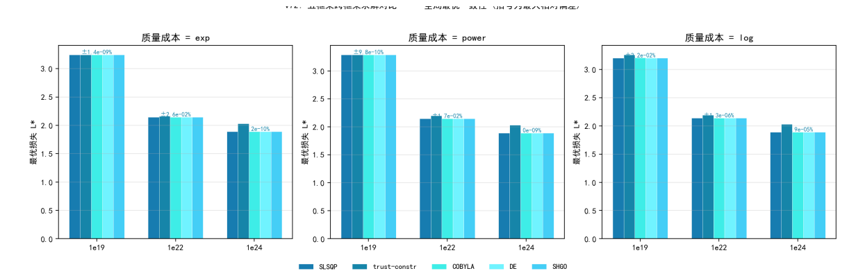
图 7.36 五框架求解对比：SLSQP/COBYLA/DE/SHGO 在 9 实例上一致到 10^{-6} 量级（括号号为四框架最大相对偏差）， trust-constr 内点法在边界角点最优处失稳。
