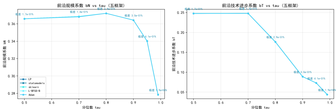
图 8.58 分位数族 \times 五框架：每个 \tau 上五框架一致； b_T 随 \tau 单调递减、 b_N 峰后回落。
