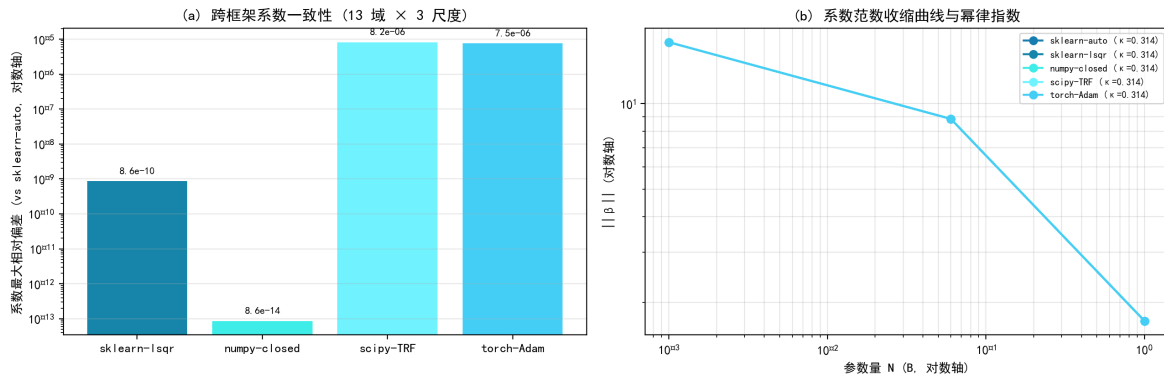
图 5.7 五框架岭回归交叉验证：系数范数收缩曲线完全重合， \kappa = 0.314031 （极差 3 \times 10^{-10} ）。
