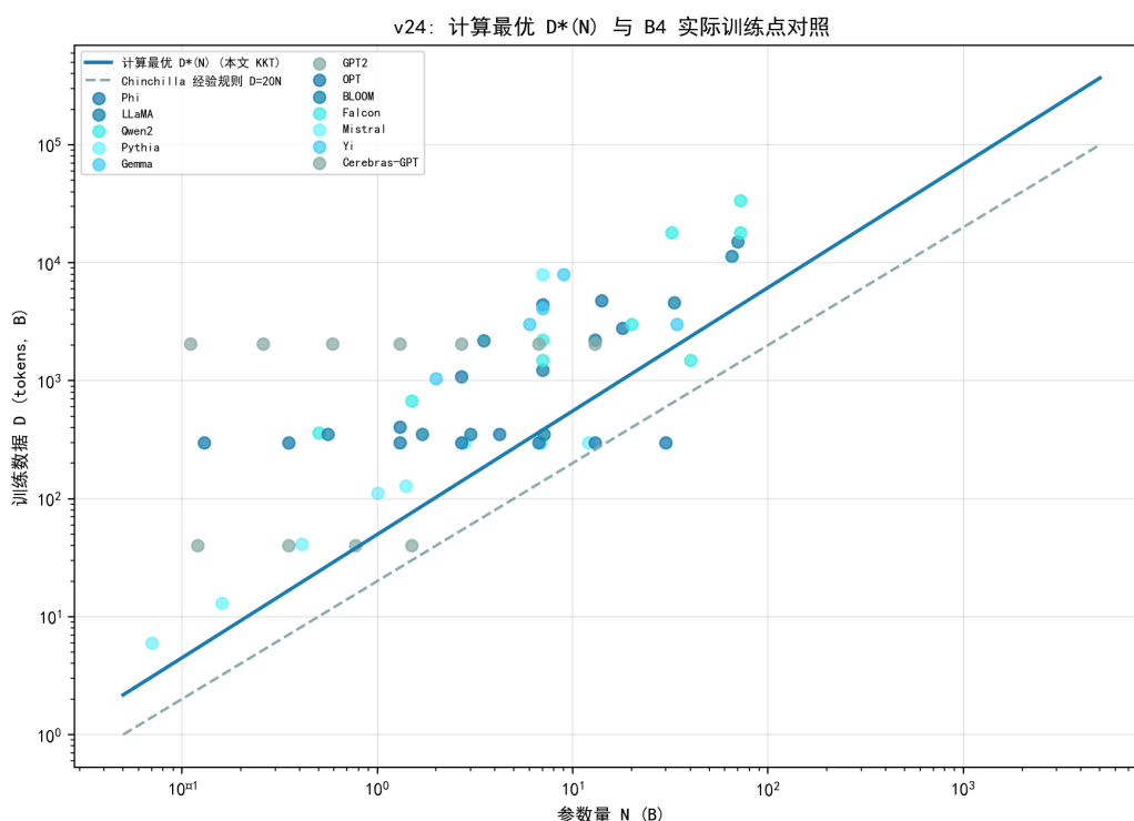
图 7.42 计算最优数据曲线 D^*(N) 、Chinchilla 经验规则与 B4 实际训练点。
