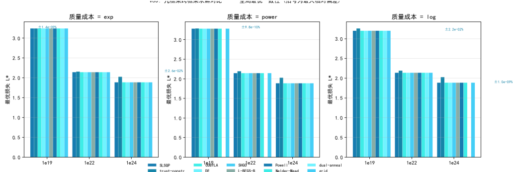
图 7.36 九框架求解对比：SLSQP/COBYLA/DE/SHGO/L-BFGS-B/Powell/Nelder-Mead/ 双退火/网格在 9 实例上一致到 10^{-6} 量级（括号为九路径最大相对偏差），trust-constr 内点法在边界角点最优处失稳。
