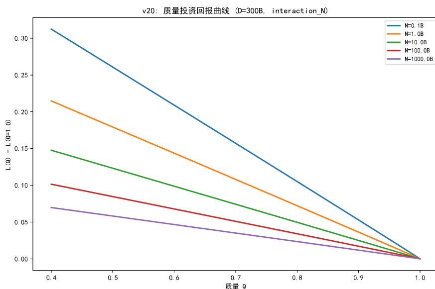
图 6.9 质量投资回报曲线 ( D = 300B ): L(Q) 相对 L(Q = 1) 随 N 变化。
