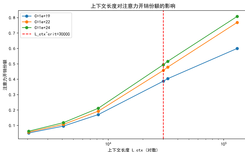
图 7.15 注意力开销份额随上下文长度的变化（红色虚线为临界点 30000）。
