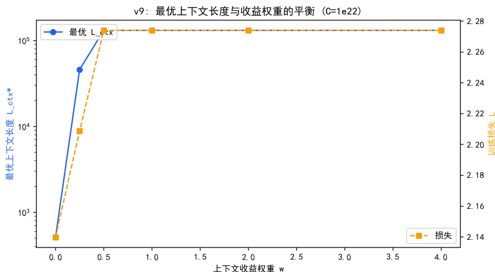
图 7.17 最优上下文长度与收益权重 w 的平衡 ( C = 10^{22} )。
