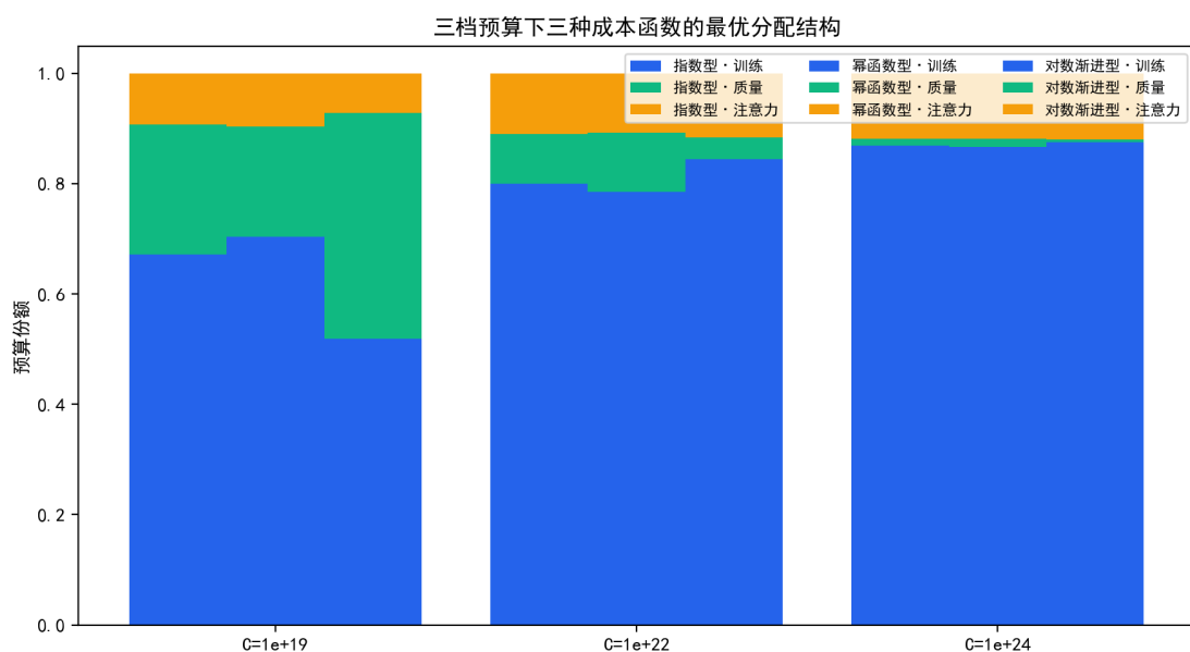
图 7.11 三档预算下三种质量成本函数的最优成本份额结构。
