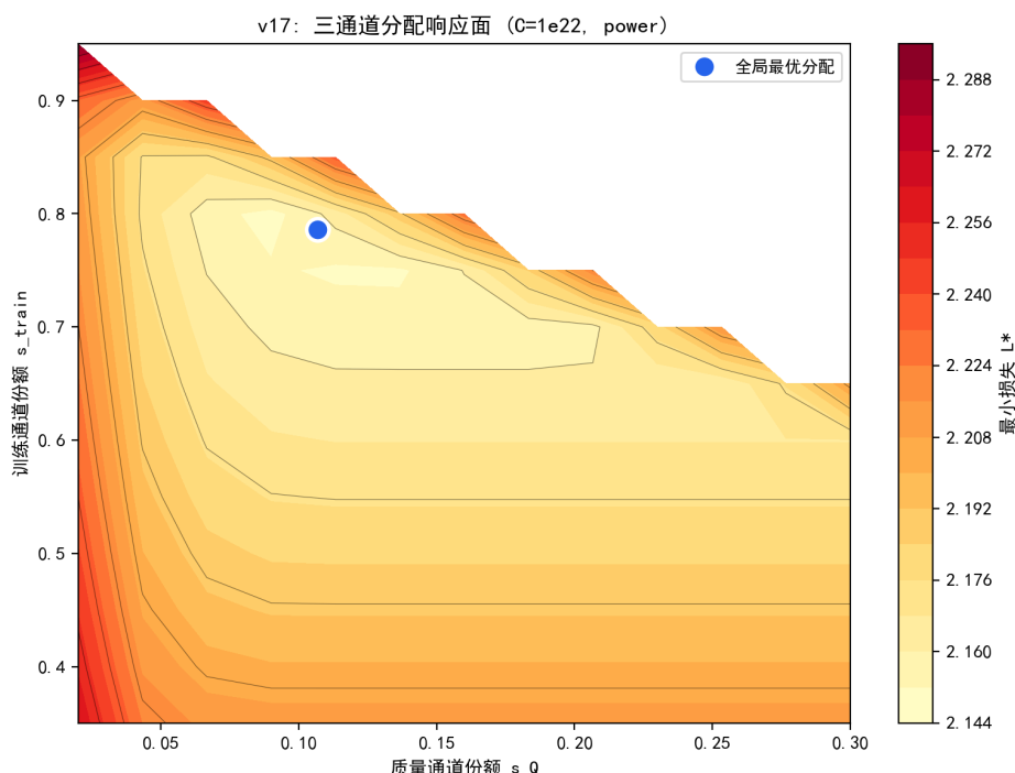
图 7.18 三通道分配响应面 ( C = 10^{22} , 幂成本; 蓝点为全局最优分配)。
