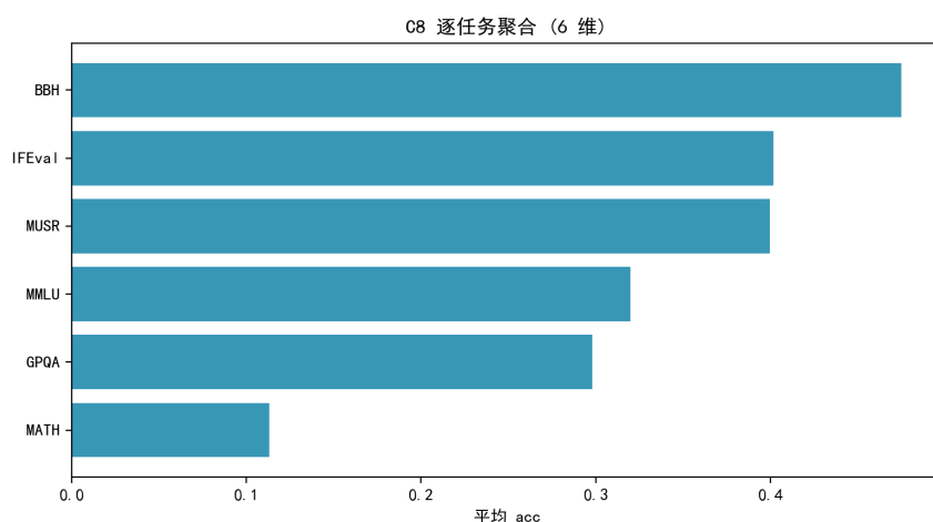
图 8.76 C8 逐任务聚合得分 (6 维)。
