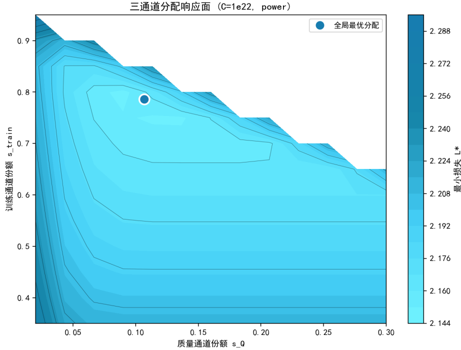
图 7.54 三通道分配响应面 ( C = 10^{22} , 幂成本; 蓝点为全局最优分配)。
