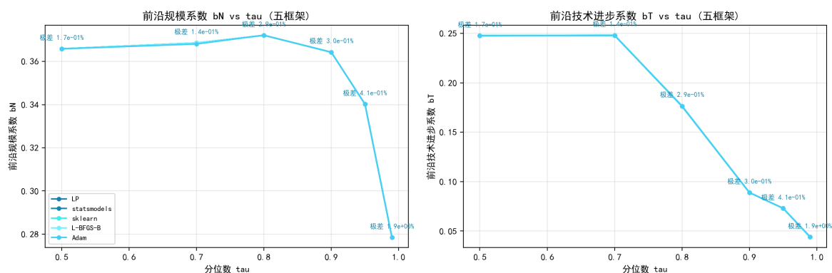
图 8.61 分位数族 \times 五框架：每个 \tau 上五框架一致； b_T 随 \tau 单调递减、 b_N 峰后回落。
