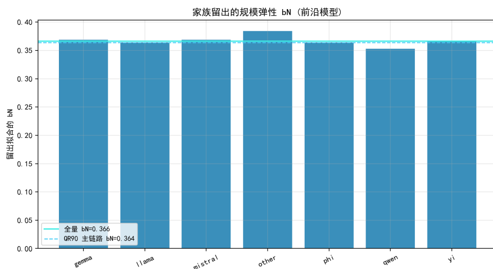
图 8.73 家族留下的规模弹性 b_N ：全家族稳定在 0.36 附近。
